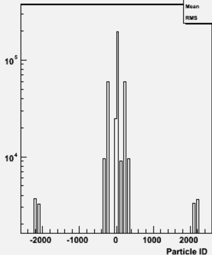
Particle ID : w102083 n3n3cce1e1_o
