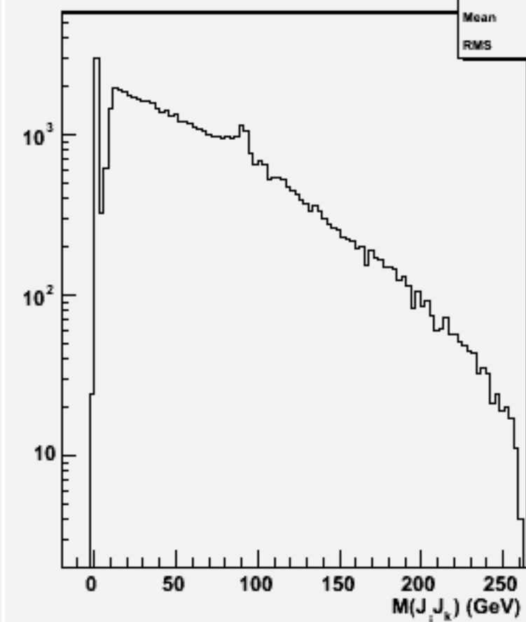
2jets mass(All comb)w102083 n3n3cce1e1_o
