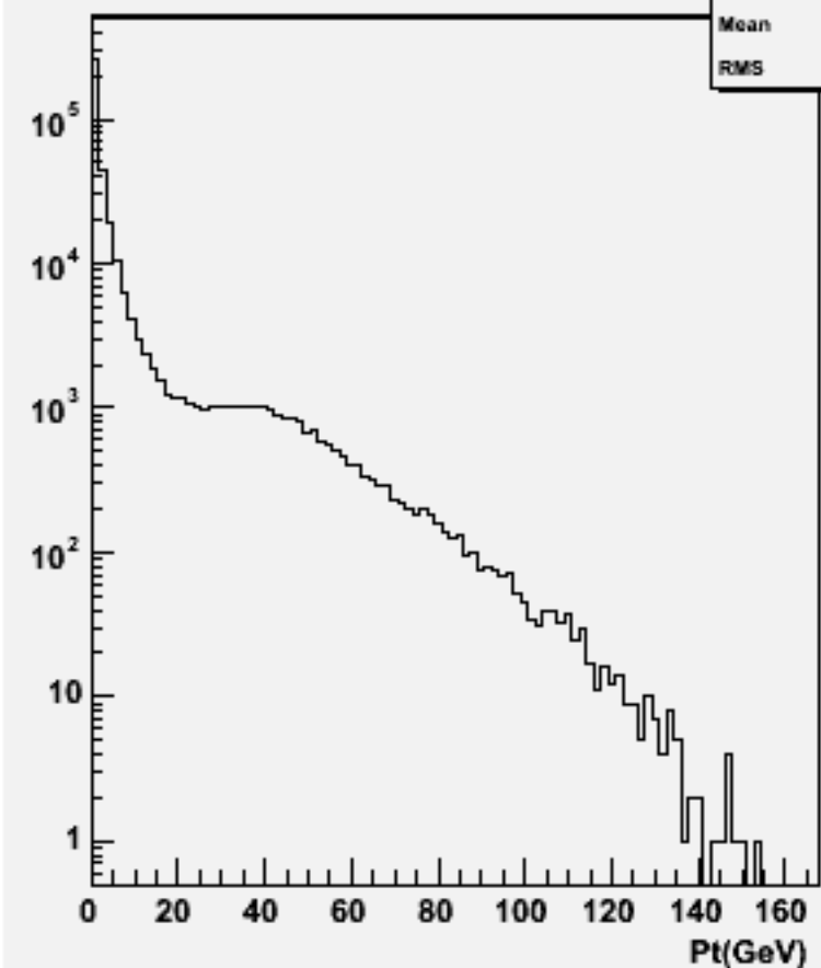
Particle Pt : w102083 n3n3cce1e1_o
