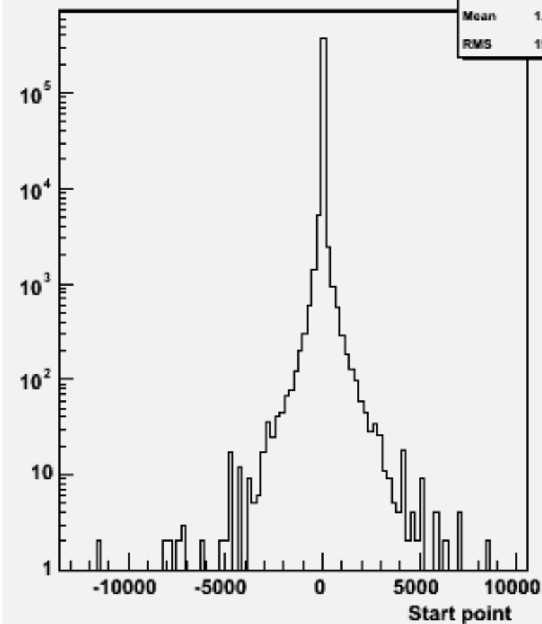
Start point Z : w102083 n3n3cce1e1_o
