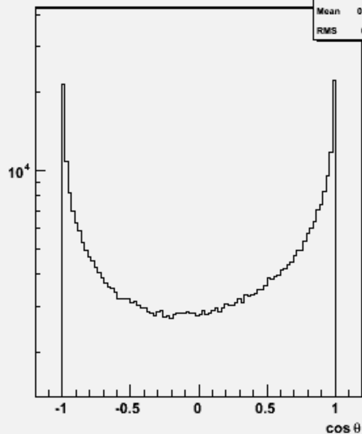
Particle cosθ : w102083 n3n3cce1e1_o
