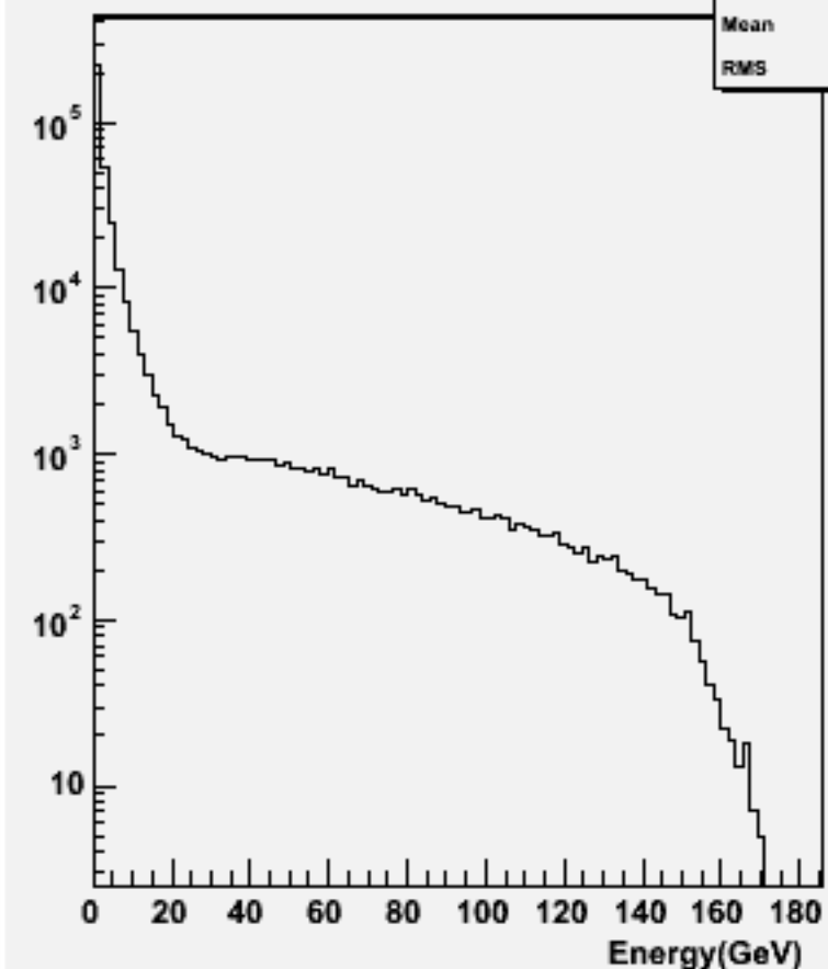
Particle Energy : w102083 n3n3cce1e1_o
