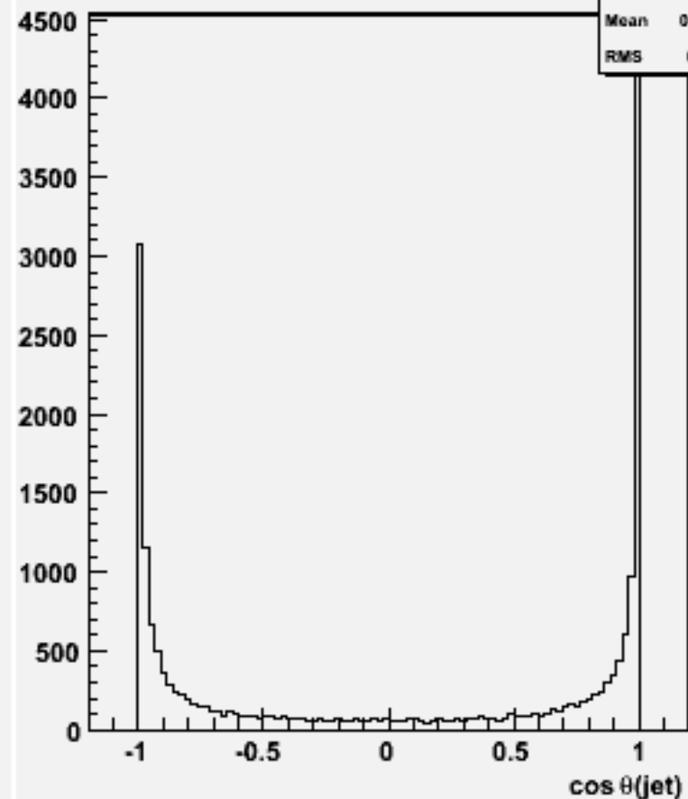
cos \theta for 2-jets :w102083 n3n3cce1e1_o
