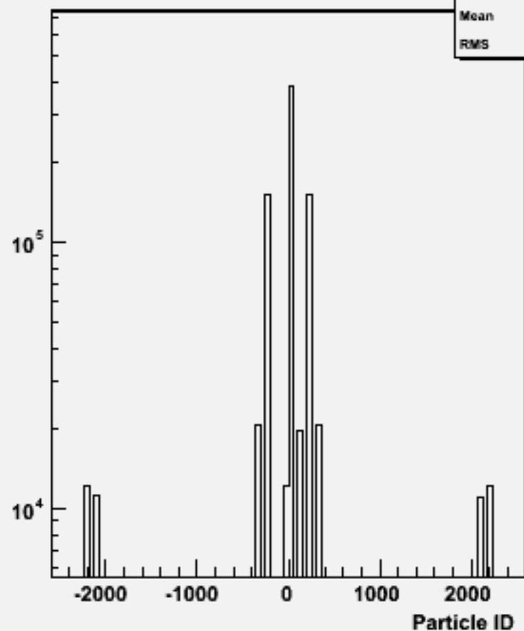
Particle ID : w102076 n3n3uuss_o
