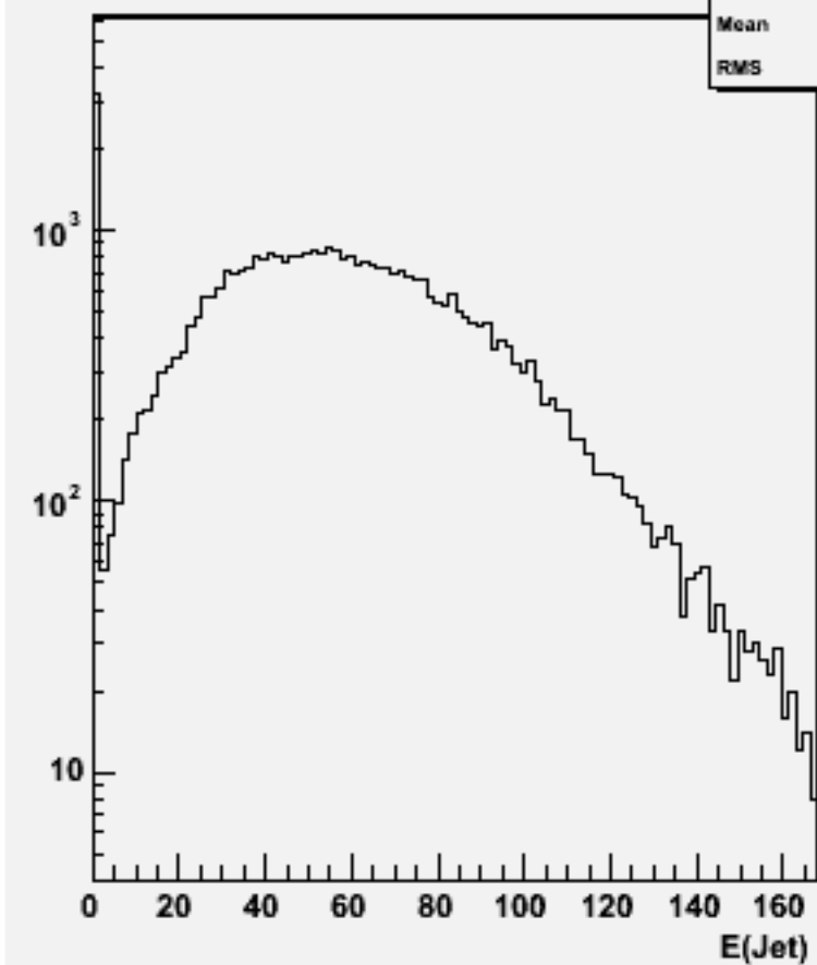
Jet energies(All jets)w102076 n3n3uuss_o
