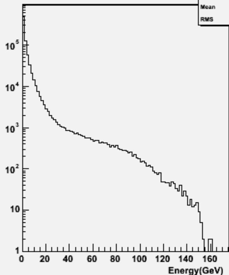
Particle Energy : w102076 n3n3uuss_o
