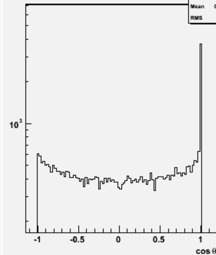
Jet cosθ (All jets)w102076 n3n3uuss_o
