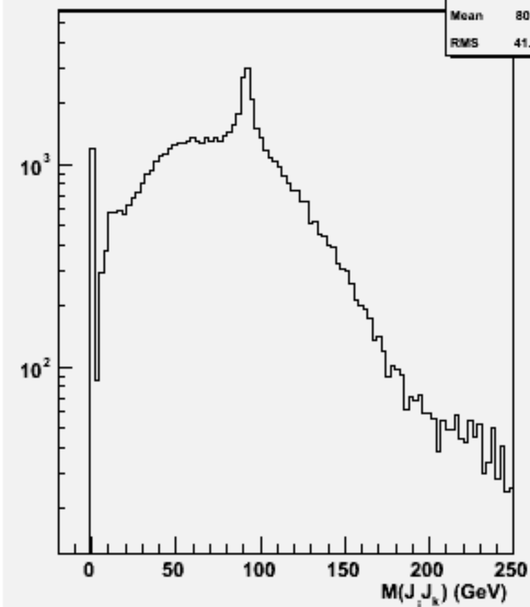
2jets mass(All comb)w102076 n3n3uuss_o
