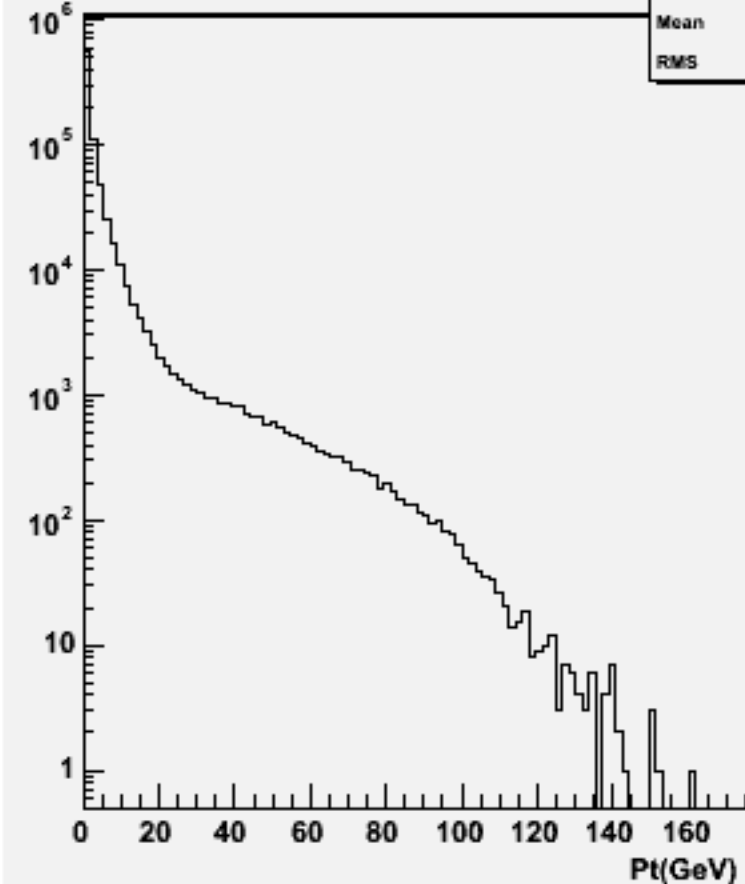
Particle Pt : w102076 n3n3uuss_o
