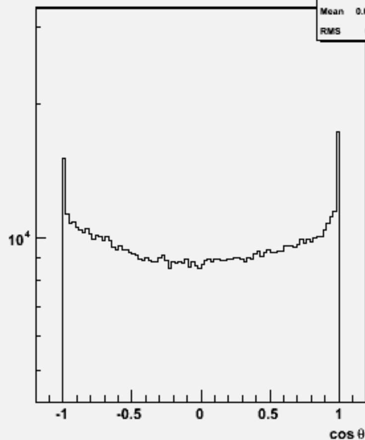
Particle cos \theta : w102076 n3n3uuss_o
