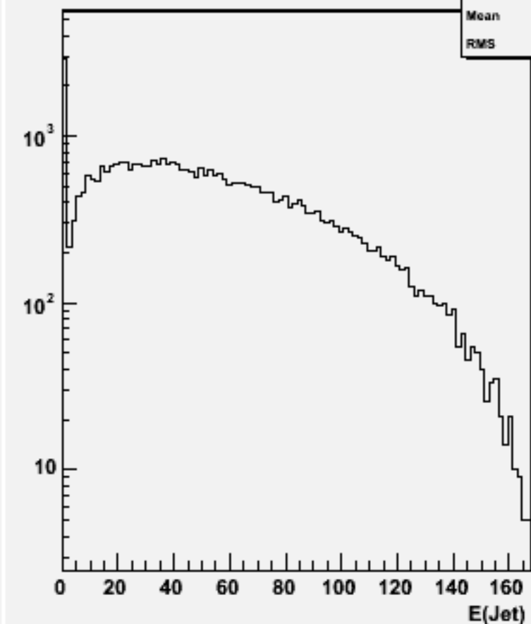
Jet energies(All jets)w102073 n3n3uue2e2_o
