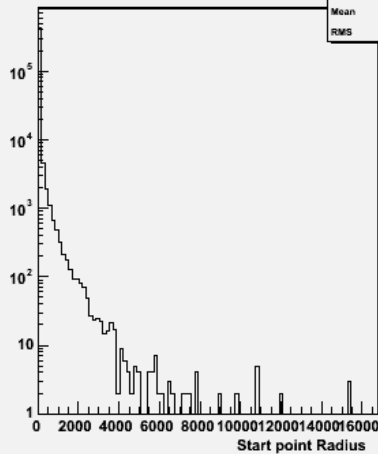
Start point R : w102073 n3n3uue2e2_o
