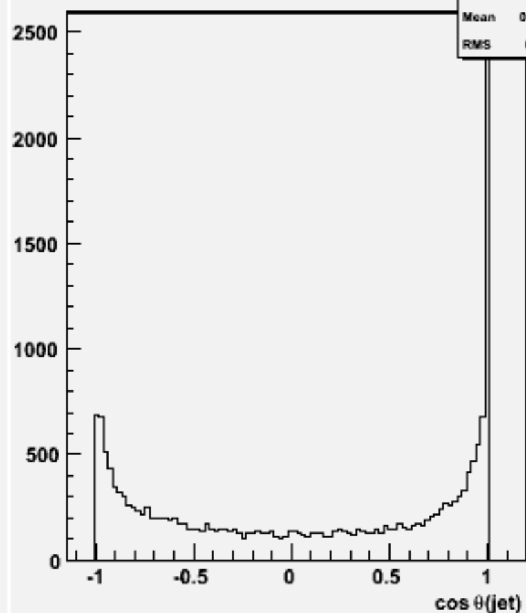
cos \theta for 2-jets :w102073 n3n3uue2e2_o
