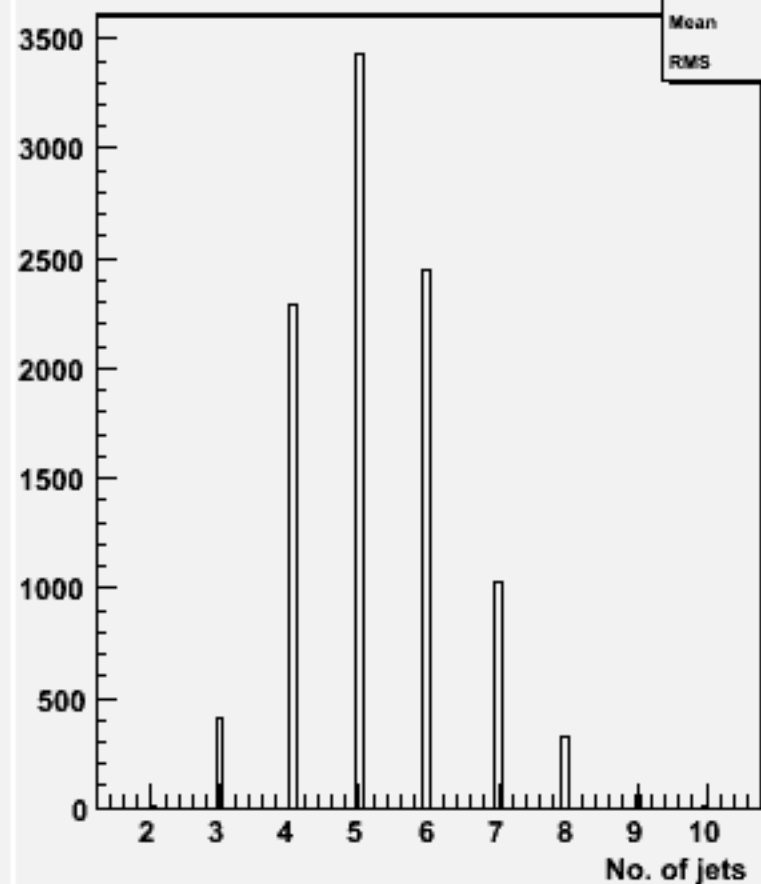
No. jets (ycut=0.001) : w102073 n3n3uue2e2_o
