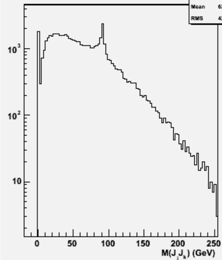
2jets mass(All comb)w102073 n3n3uue2e2_o
