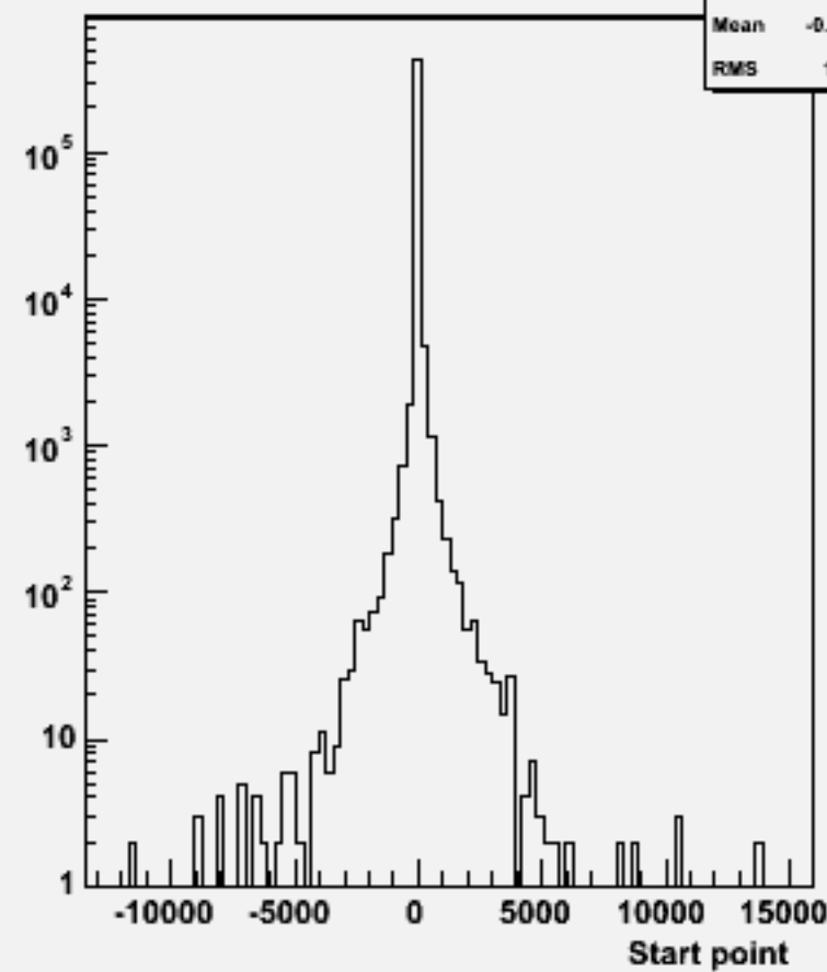
Start point Z : w102073 n3n3uue2e2_o
