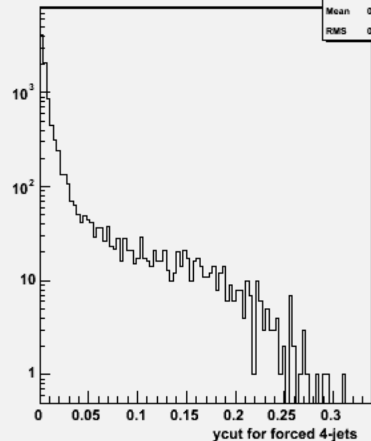
Ycut for 4-jets :w102072 n3n3uue2e2_o
