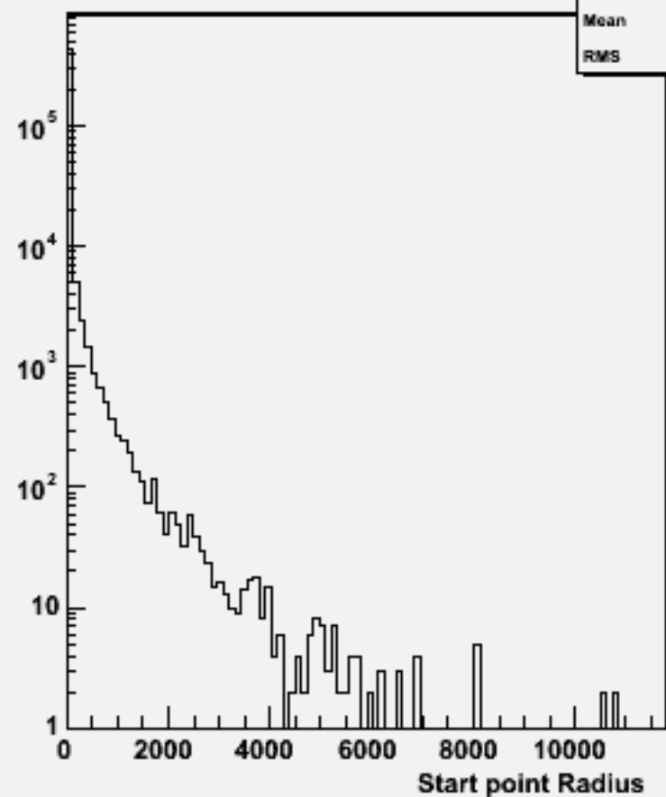
Start point R : w102072 n3n3uue2e2_o
