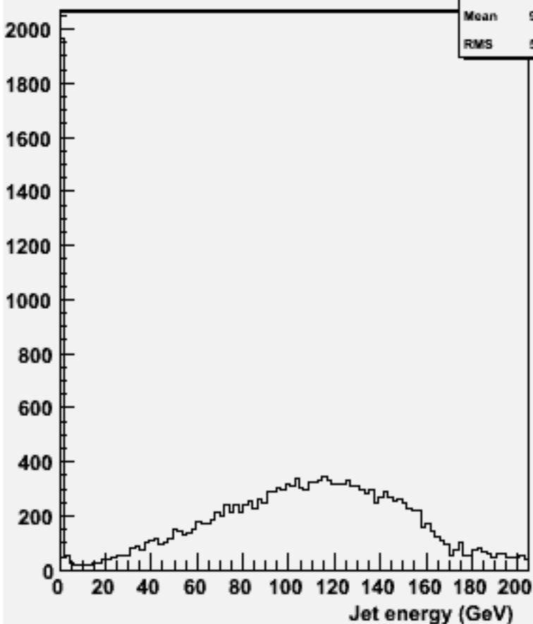
energy for 2-jets :w102072 n3n3uue2e2_o
