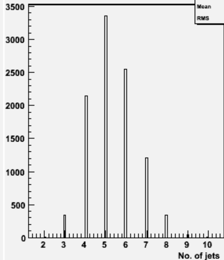
No. jets (ycut=0.001) : w102072 n3n3uue2e2_o
