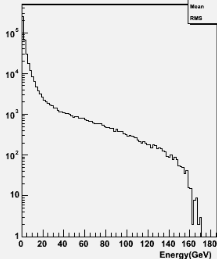
Start point R : w102072 n3n3uue2e2_o
