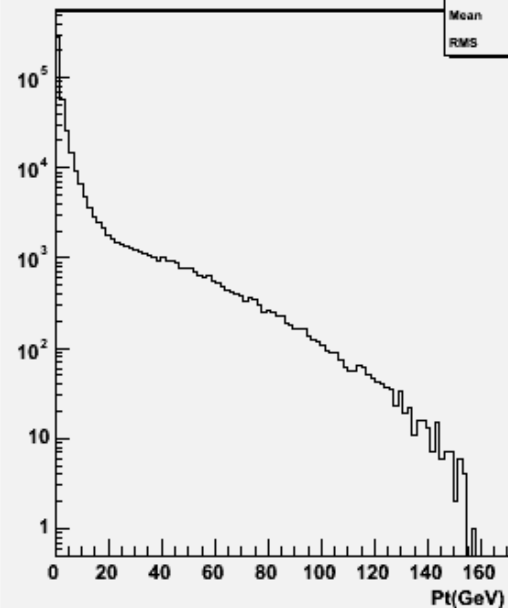
Start point Z : w102072 n3n3uue2e2_o
