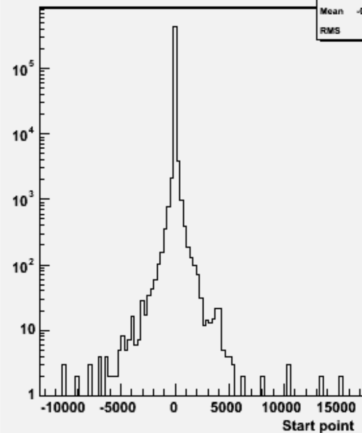
Start point Z : w102072 n3n3uue2e2_o
