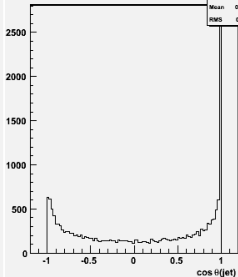
cos \theta for 2-jets :w102072 n3n3uue2e2_o
