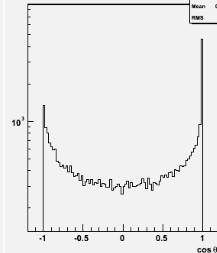
Jet cos \theta (All jets)w102072 n3n3uue2e2_o
