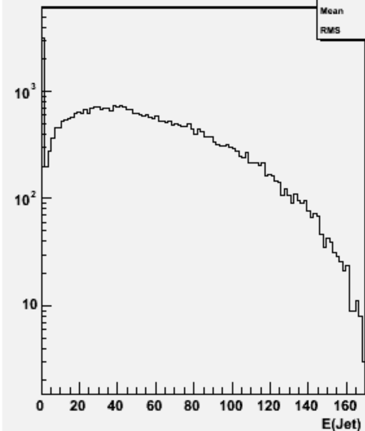
Jet energies(All jets)w102072 n3n3uue2e2_o
