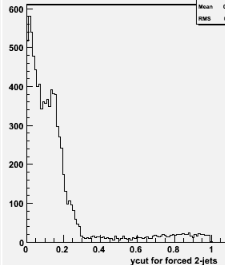
Ycut for 2-jets :w102072 n3n3uue2e2_o
