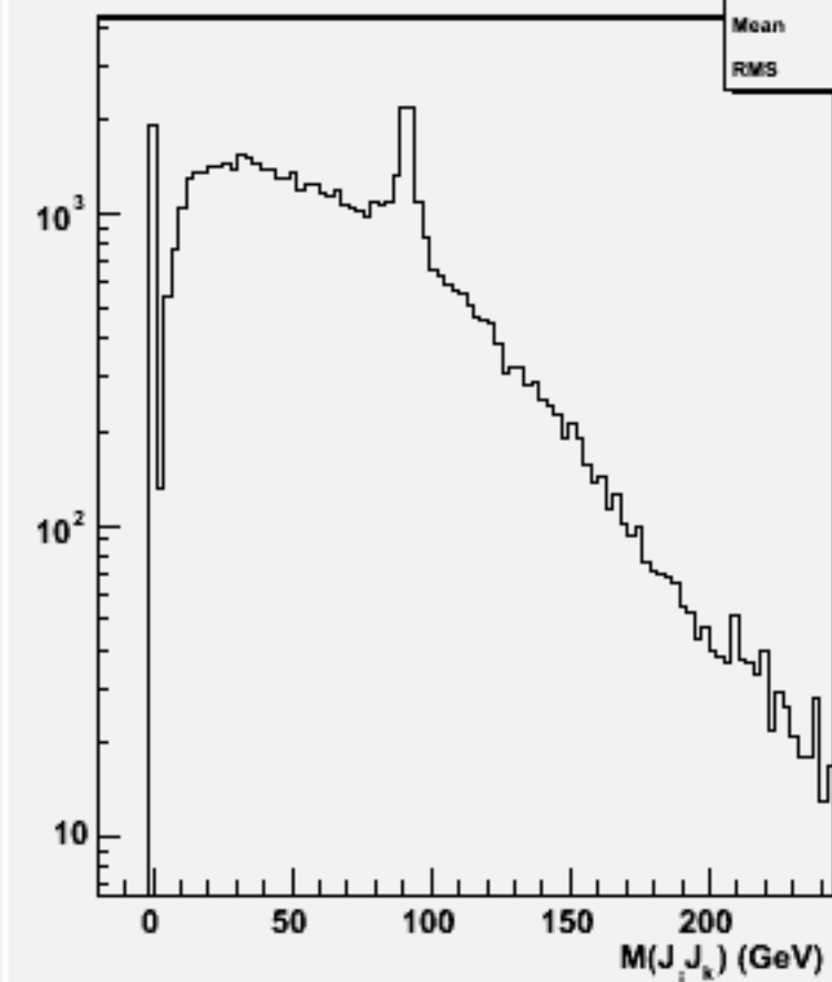
2jets mass(All comb)w102072 n3n3uue2e2_o
