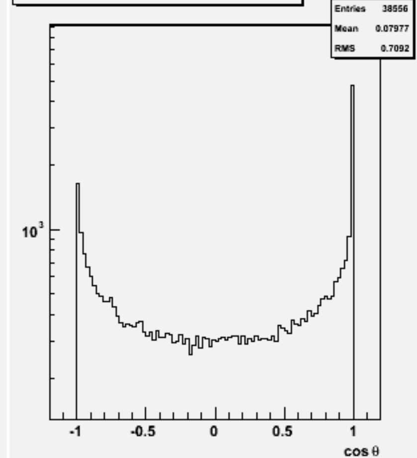
Jet cos \theta (All jets)w102068 n3n3uue1e1_o
