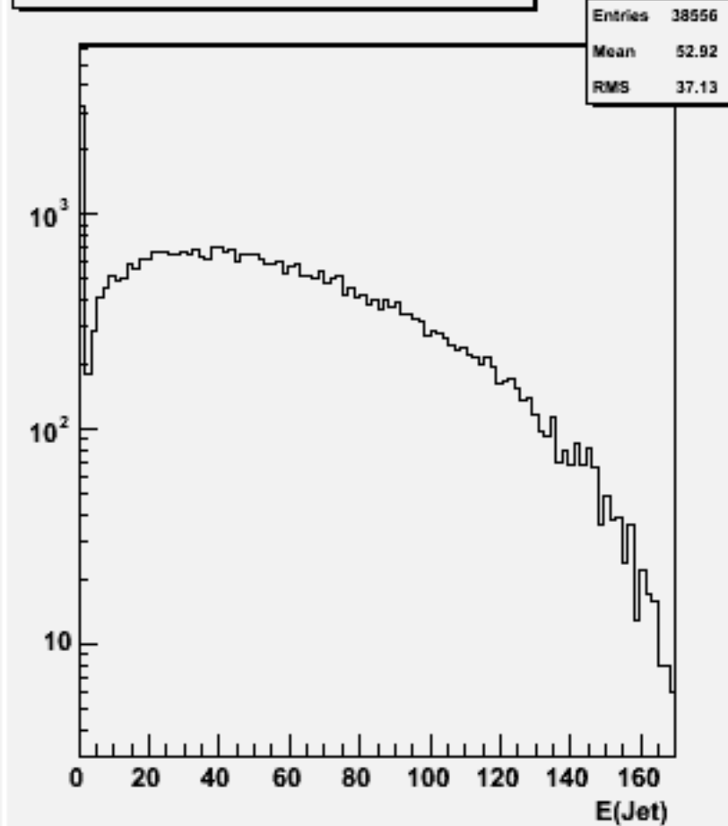
Jet energies(All jets)w102068 n3n3uue1e1_o
