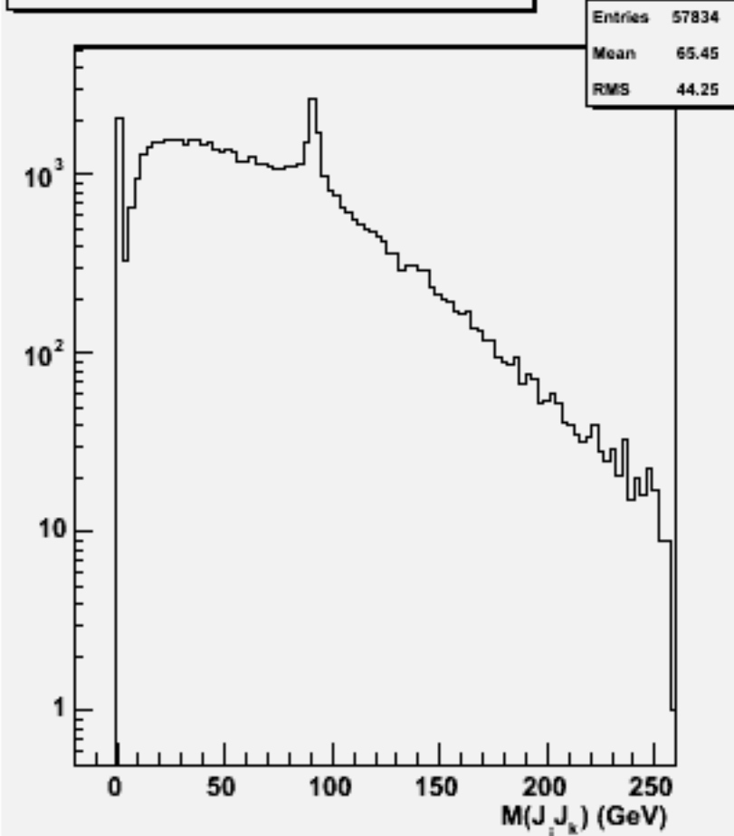
2jets mass(All comb)w102068 n3n3uue1e1_o
