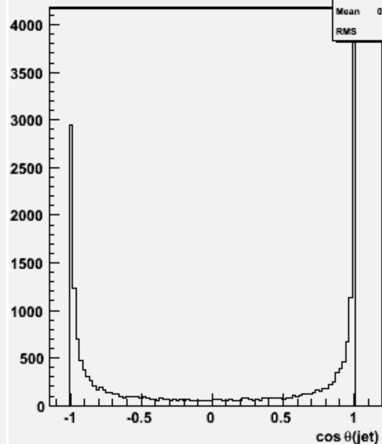
cos \theta for 2-jets :w102067 n3n3uue1e1_o
