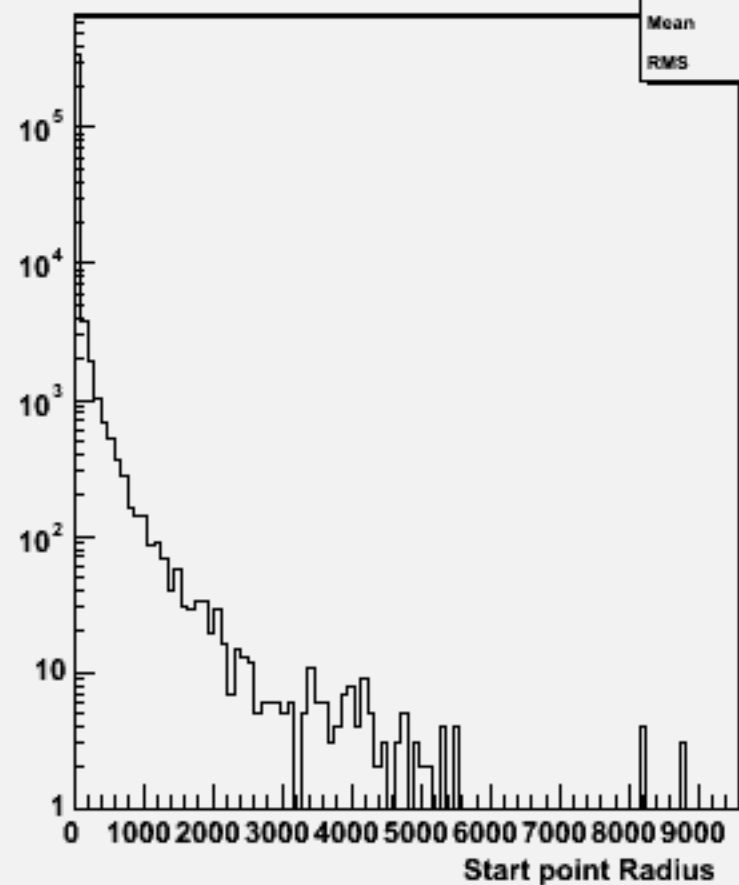
Start point R : w102067 n3n3uue1e1_o
