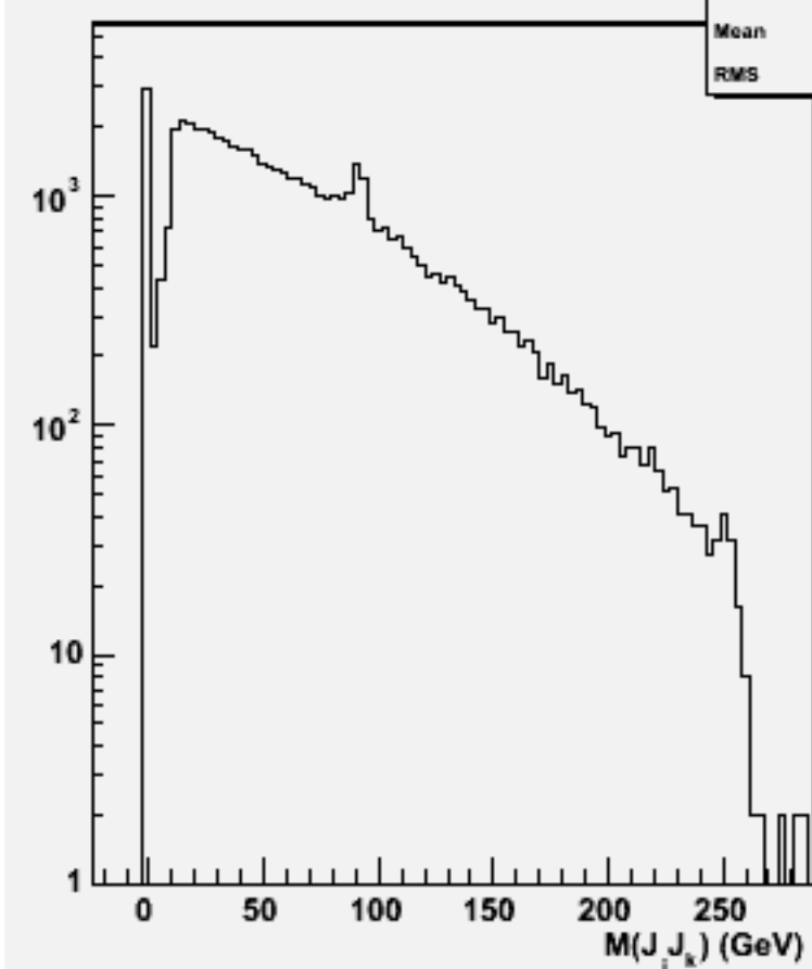
2jets mass(All comb)w102067 n3n3uue1e1_o
