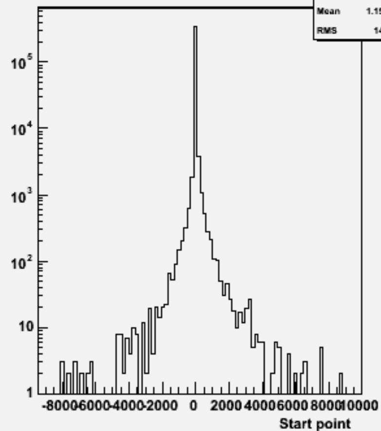
Start point Z : w102067 n3n3uue1e1_o
