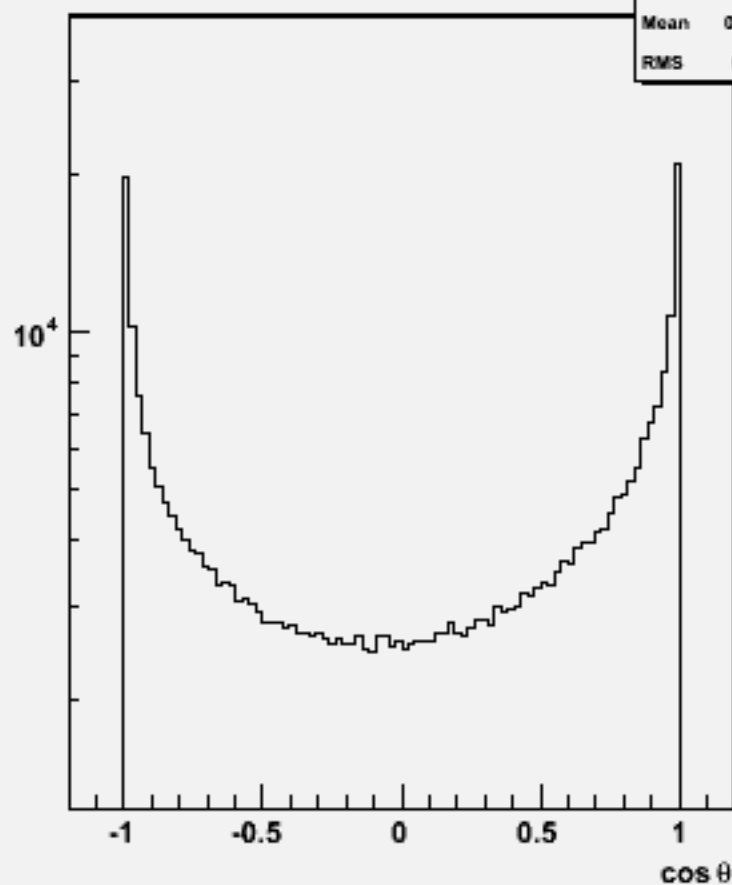
Particle cos \theta : w102067 n3n3uue1e1_o
