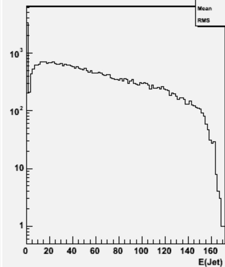
Jet energies(All jets)w102067 n3n3uue1e1_o
