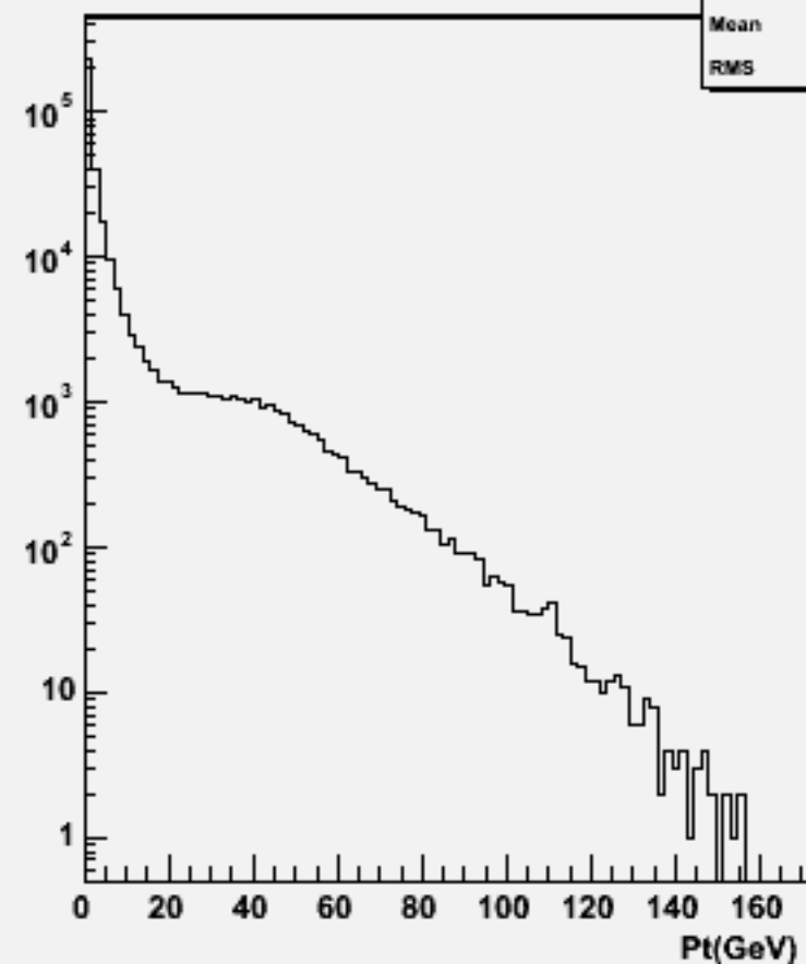
Particle Pt : w102067 n3n3uue1e1_o
