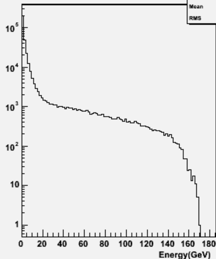
Particle Energy : w102067 n3n3uue1e1_o
