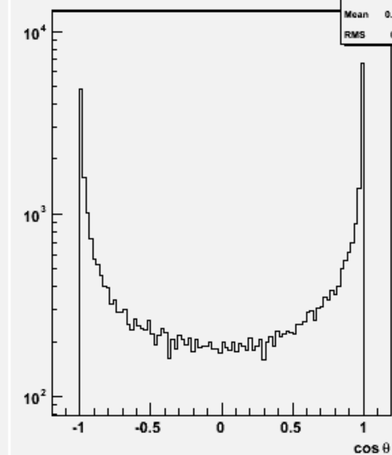
Jet cos \theta (All jets)w102067 n3n3uue1e1_o
