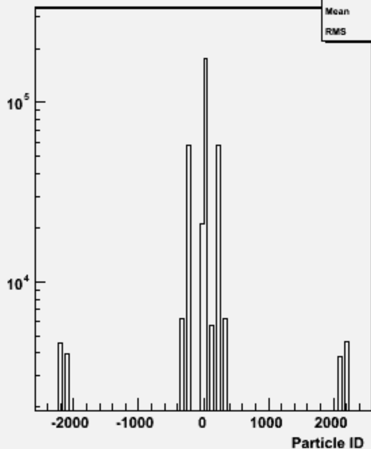
Particle ID : w102067 n3n3uue1e1_o
