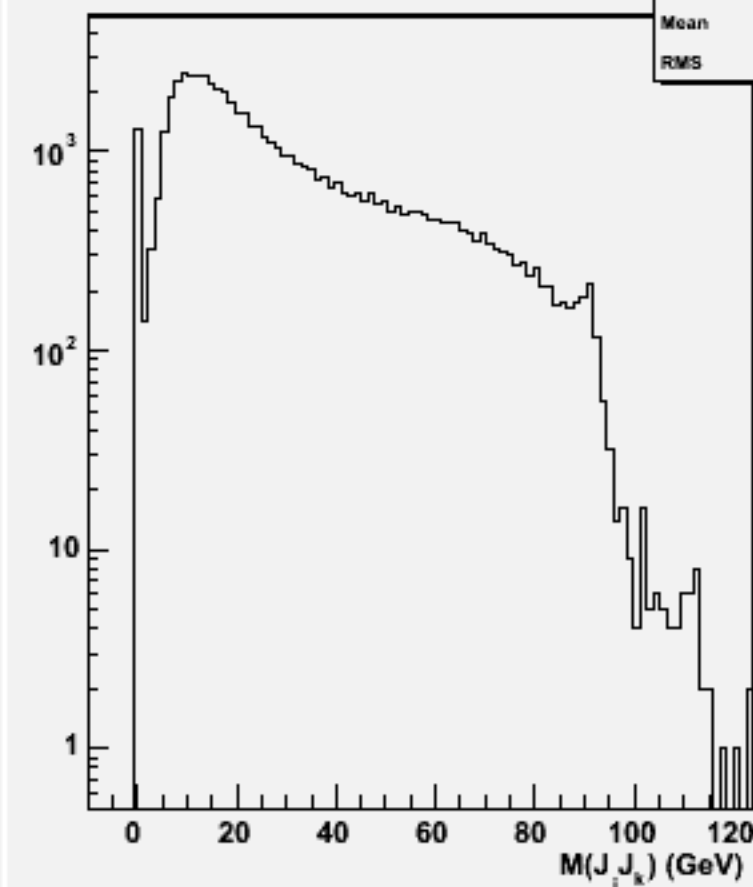
2jets mass(All comb)w102064 n3n3n3n3bb_o
