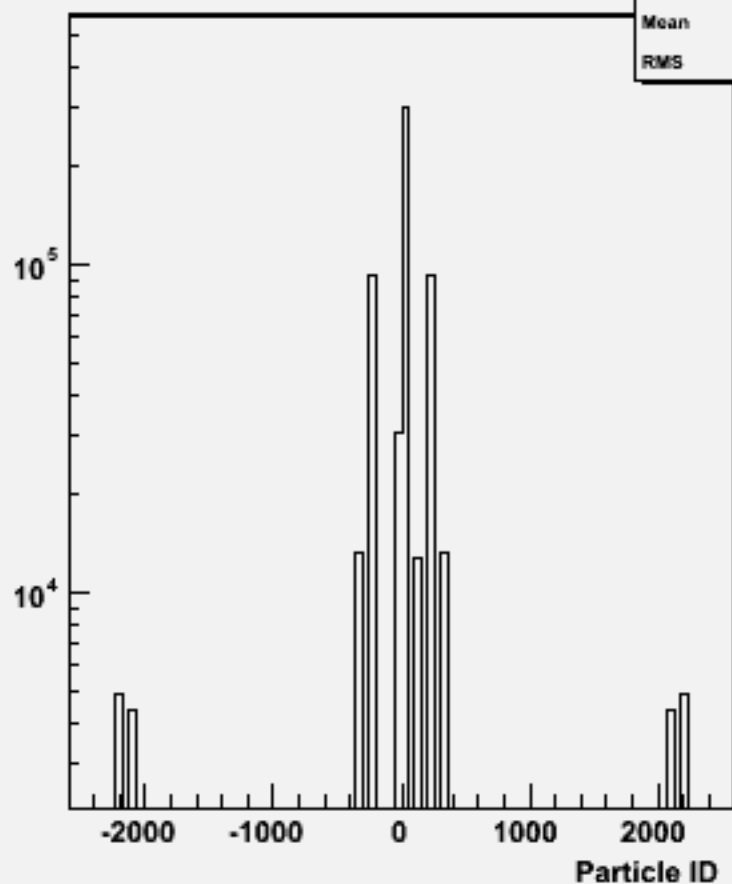
Particle ID : w102064 n3n3n3n3bb_o
