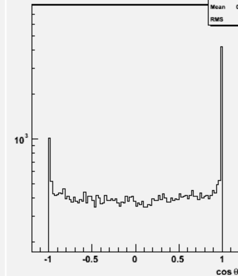
Jet cos \theta (All jets)w102064 n3n3n3n3bb_o
