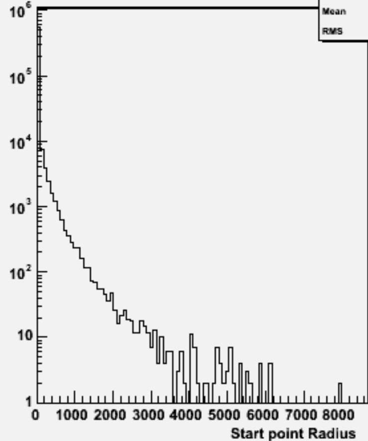
Start point R : w102064 n3n3n3n3bb_o
