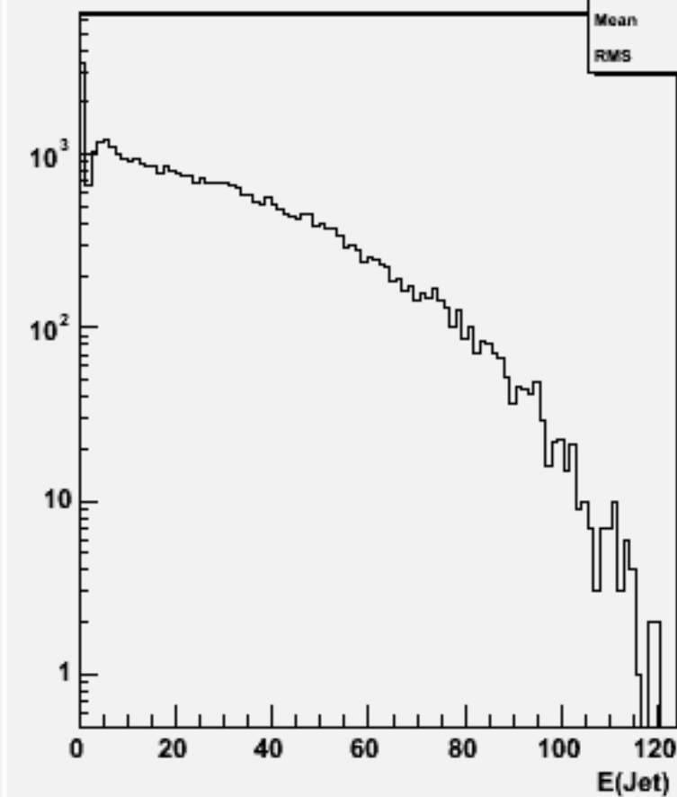
Jet energies(All jets)w102064 n3n3n3n3bb_o
