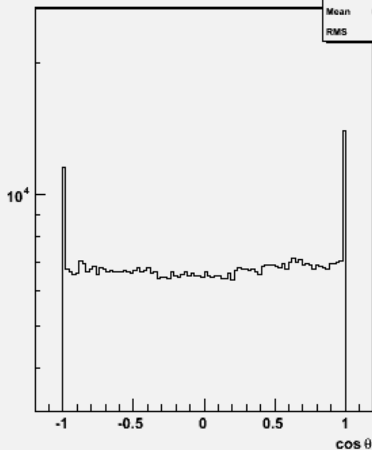
Particle cosθ : w102064 n3n3n3n3bb_o
