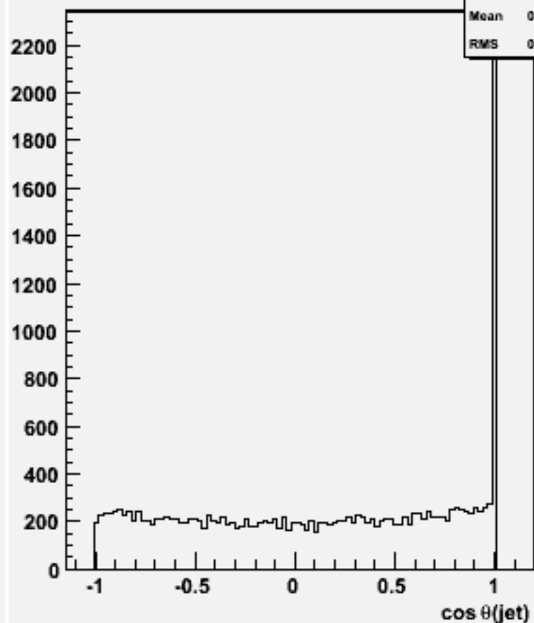
cos \theta for 2-jets :w102064 n3n3n3n3bb_o
