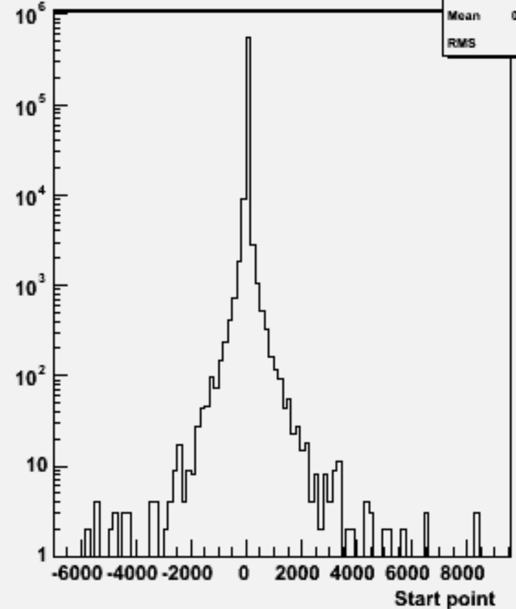
Start point Z : w102064 n3n3n3n3bb_o
