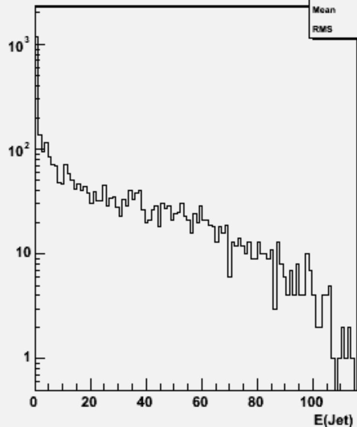
Jet energies(All jets)w102052 n3n3n3n3e2e2_o
