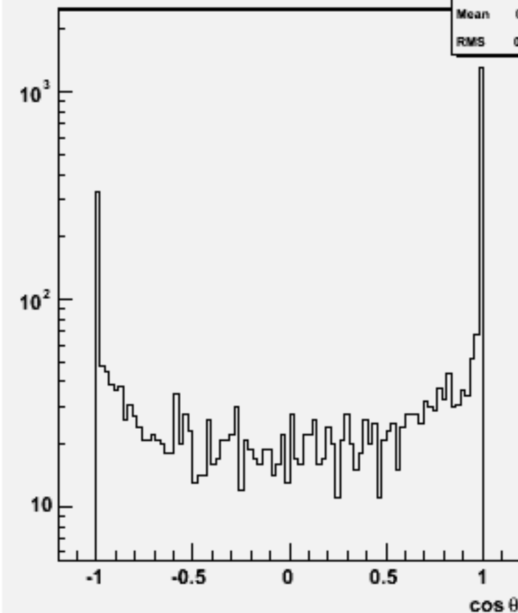
Jet cos \theta (All jets)w102052 n3n3n3n3e2e2_o
