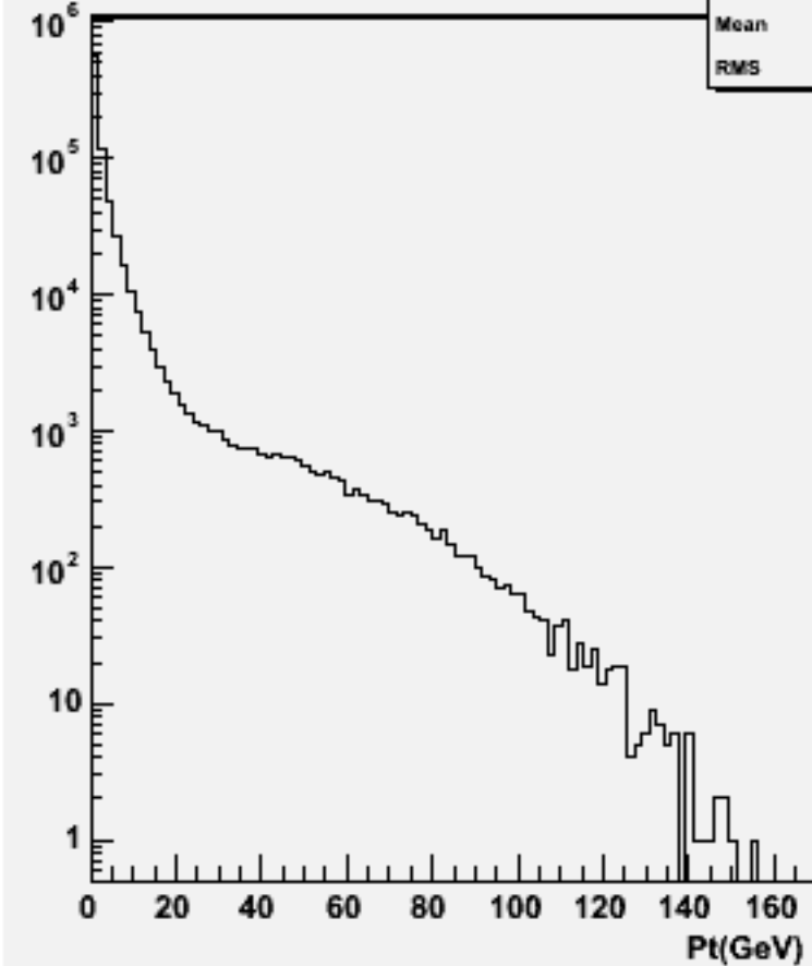
Particle Pt : w102041 n2n2ccdd_o
