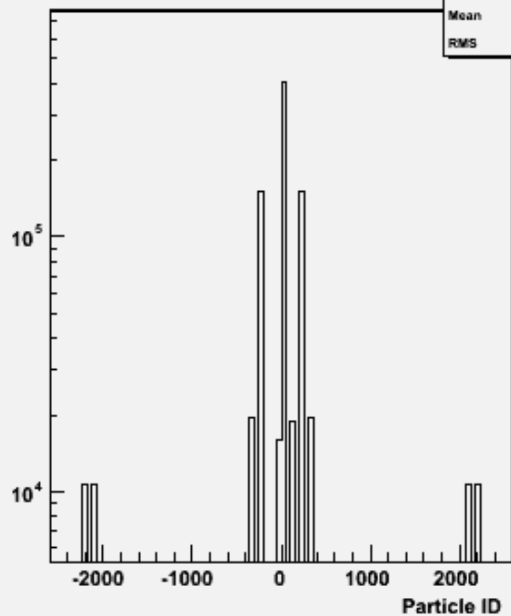
Particle ID : w102041 n2n2ccdd_o
