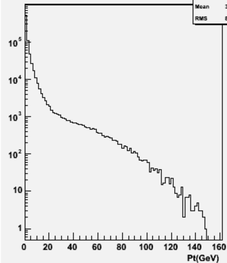
Particle Pt : w102025 n2n2uuss_o
