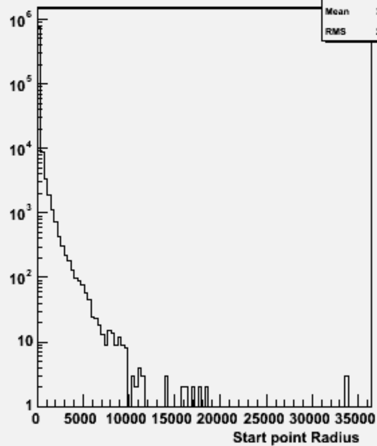
Start point R : w102025 n2n2uuss_o
