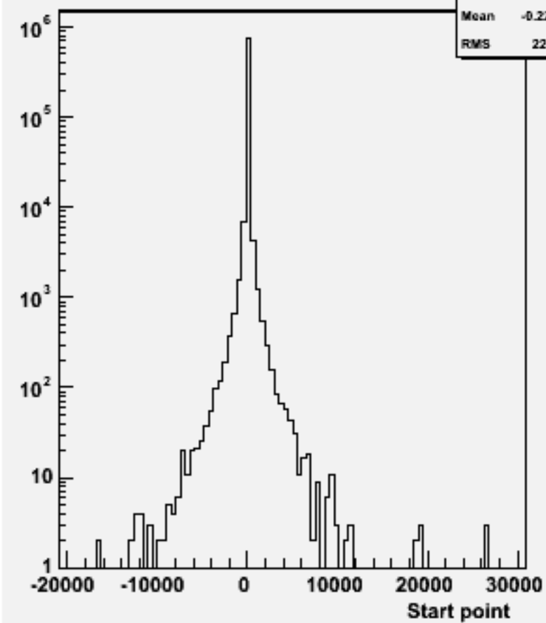
Start point Z : w102025 n2n2uuss_o
