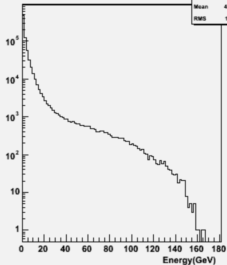
Particle Energy : w102025 n2n2uuss_o
