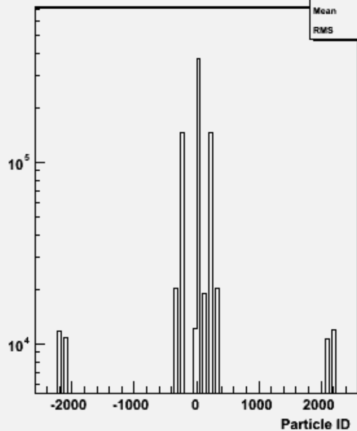
Particle ID : w102025 n2n2uuss_o
