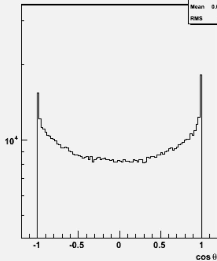
Particle cos \theta : w102025 n2n2uuss_o
