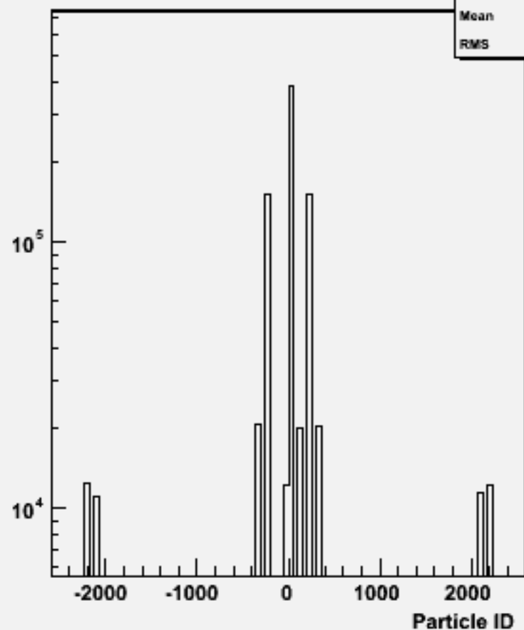
Particle ID : w102024 n2n2uuss_o
