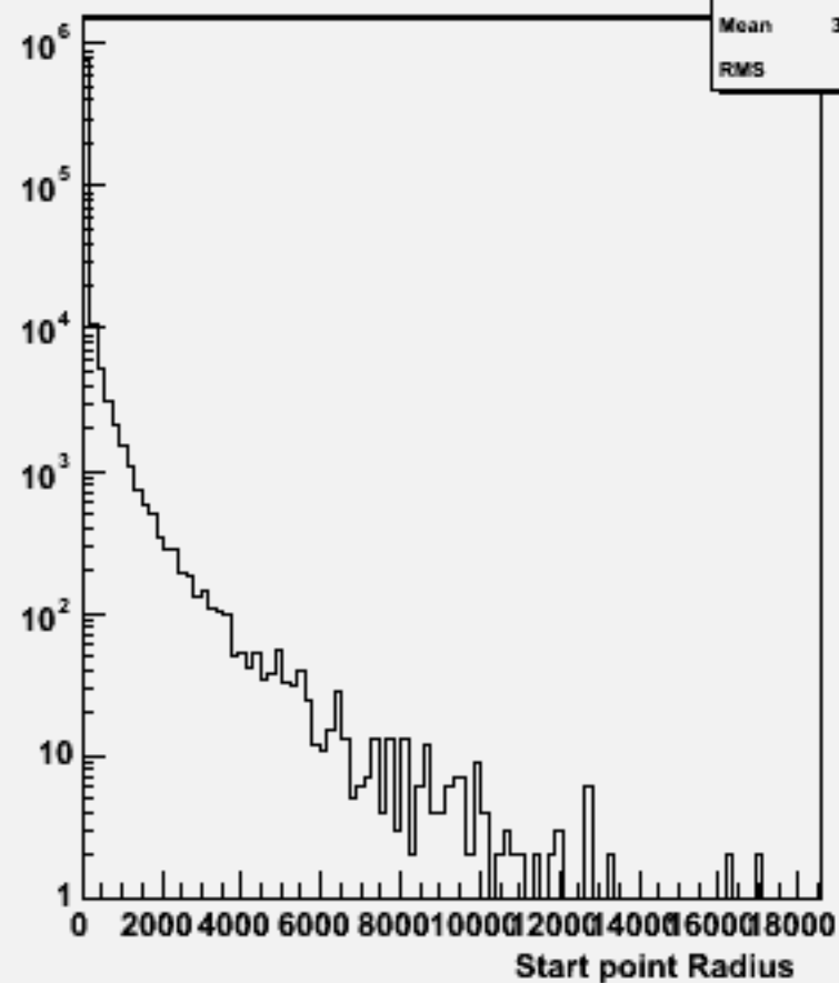
Start point R : w102024 n2n2uuss_o
