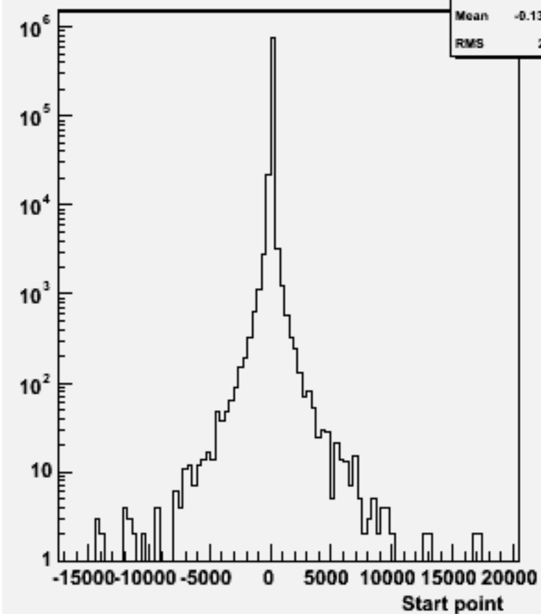
Start point Z : w102024 n2n2uuss_o
