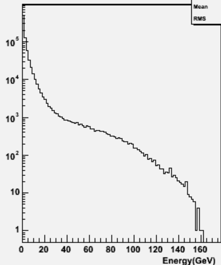
Particle Energy : w102024 n2n2uuss_o
