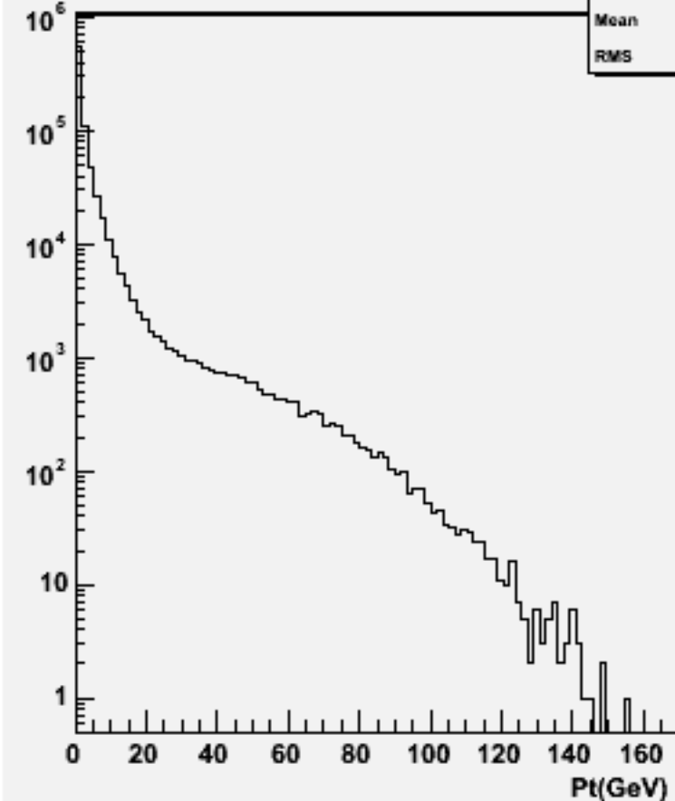
Particle Pt : w102024 n2n2uuss_o
