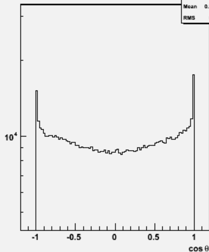
Particle cos \theta : w102024 n2n2uuss_o
