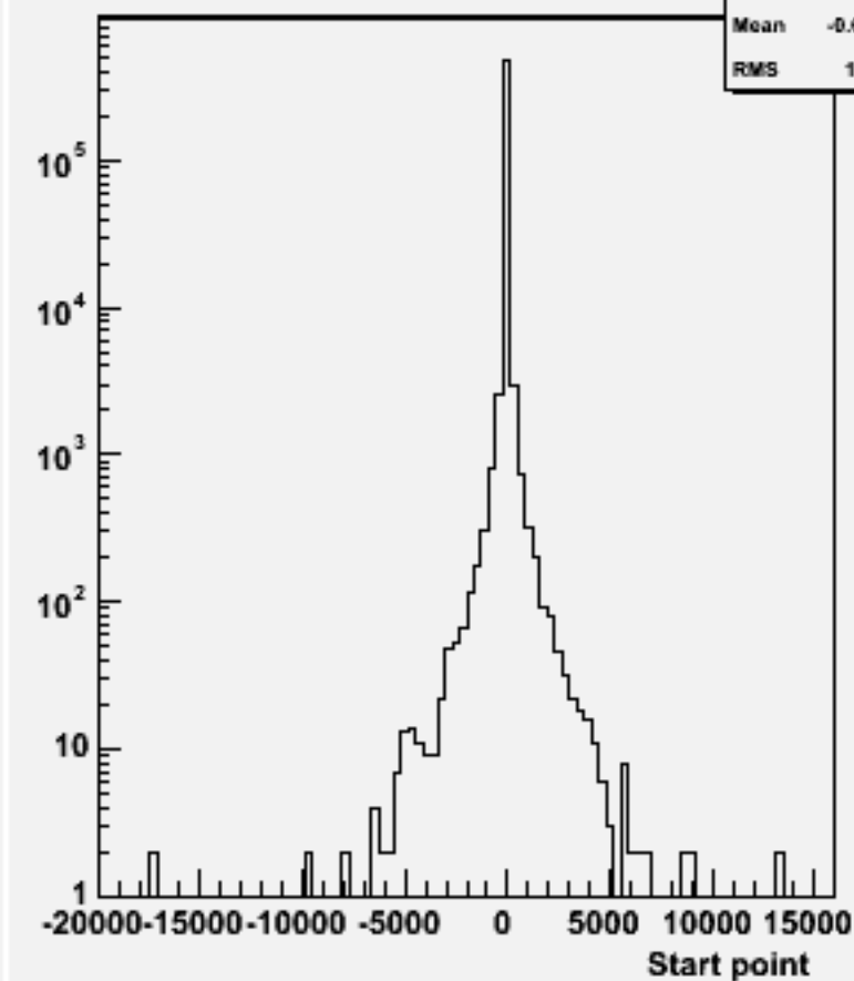
Start point Z : w102021 n2n2uue3e3_o
