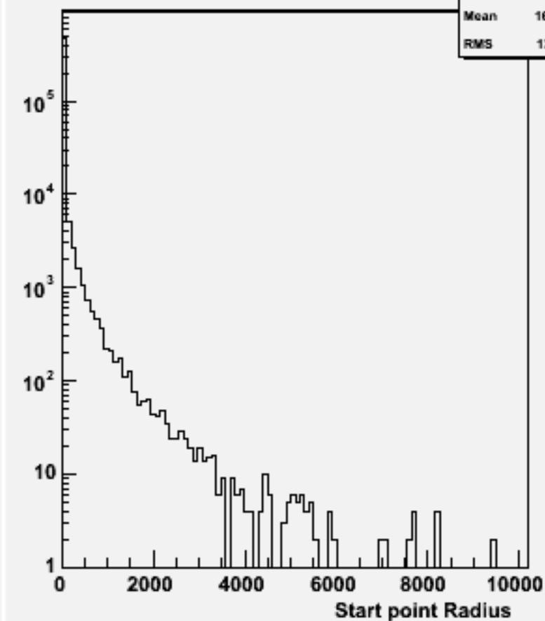
Start point R : w102021 n2n2uue3e3_o
