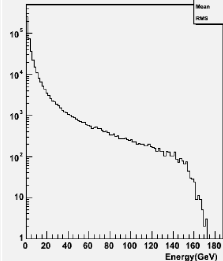
Start point R : w102021 n2n2uue3e3_o
