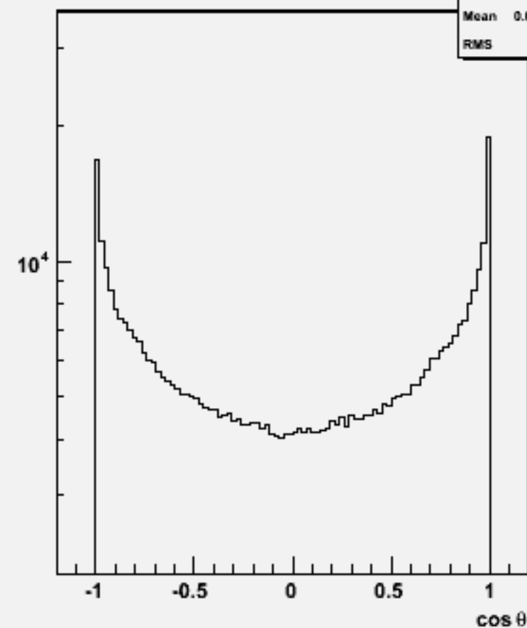
Particle cos \theta : w102021 n2n2uue3e3_o
