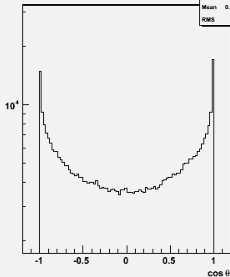
Particle cosθ : w102017 n2n2uue1e1_o
