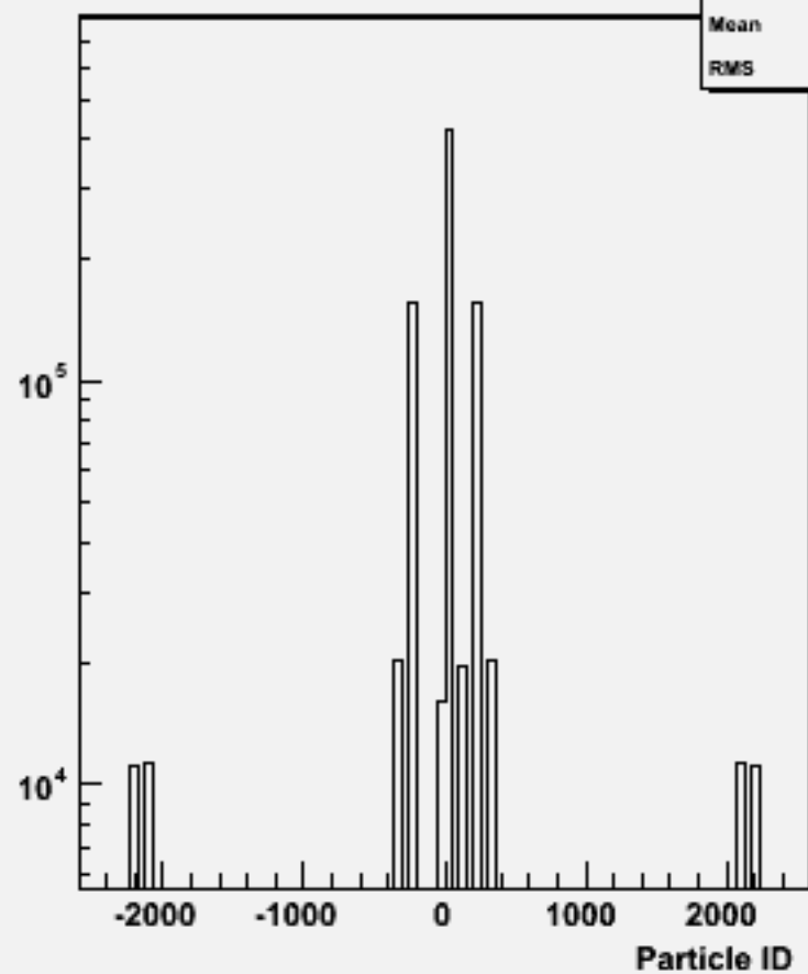
Particle ID : w101972 n1n1ccdd_o
