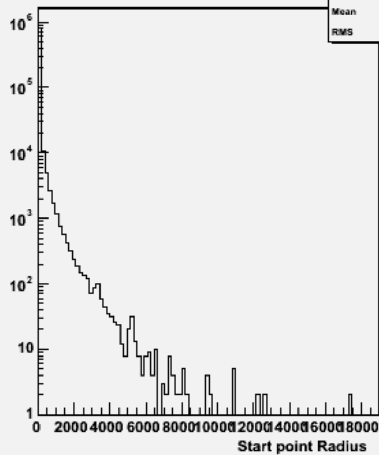
Start point R : w101972 n1n1ccdd_o
