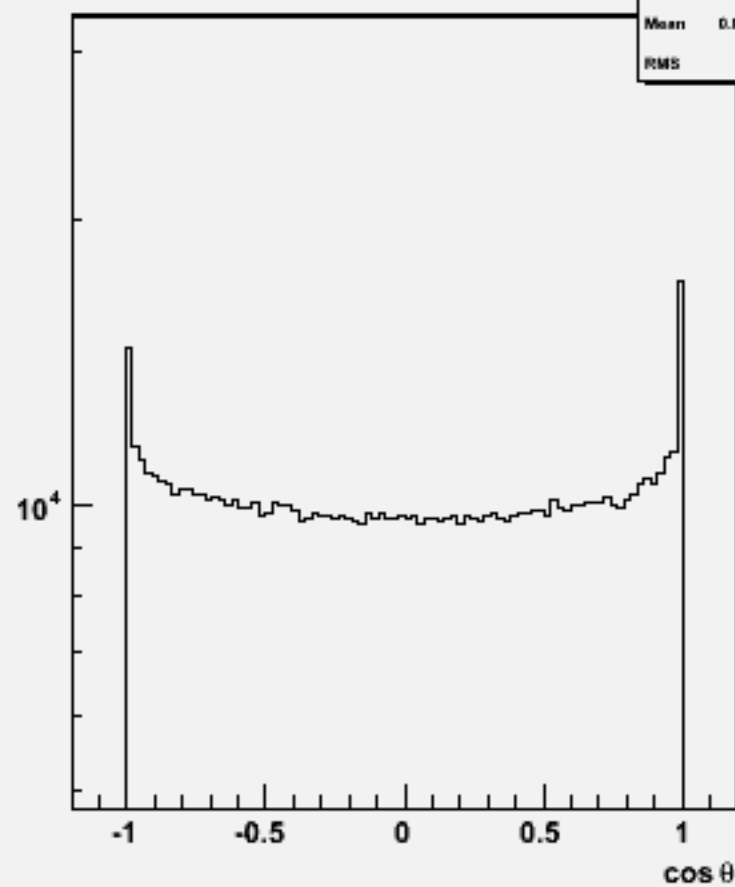
Particle cos \theta : w101972 n1n1ccdd_o
