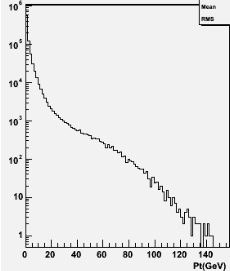
Particle Pt : w101972 n1n1ccdd_o
