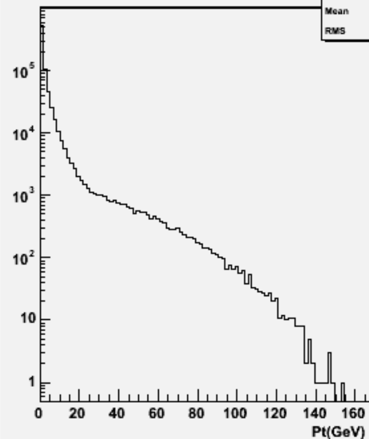
Particle Pt : w101957 n1n1uuss_o
