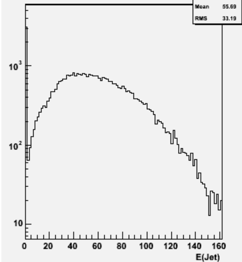
Jet energies(All jets)w101957 n1n1uuss_o
