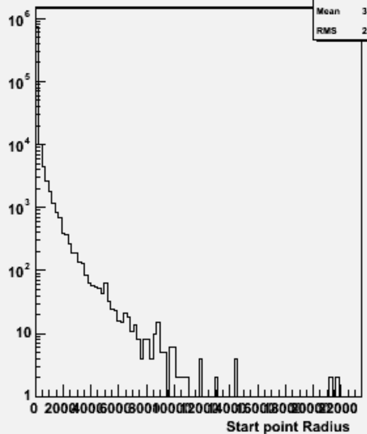
Start point R : w101957 n1n1uuss_o
