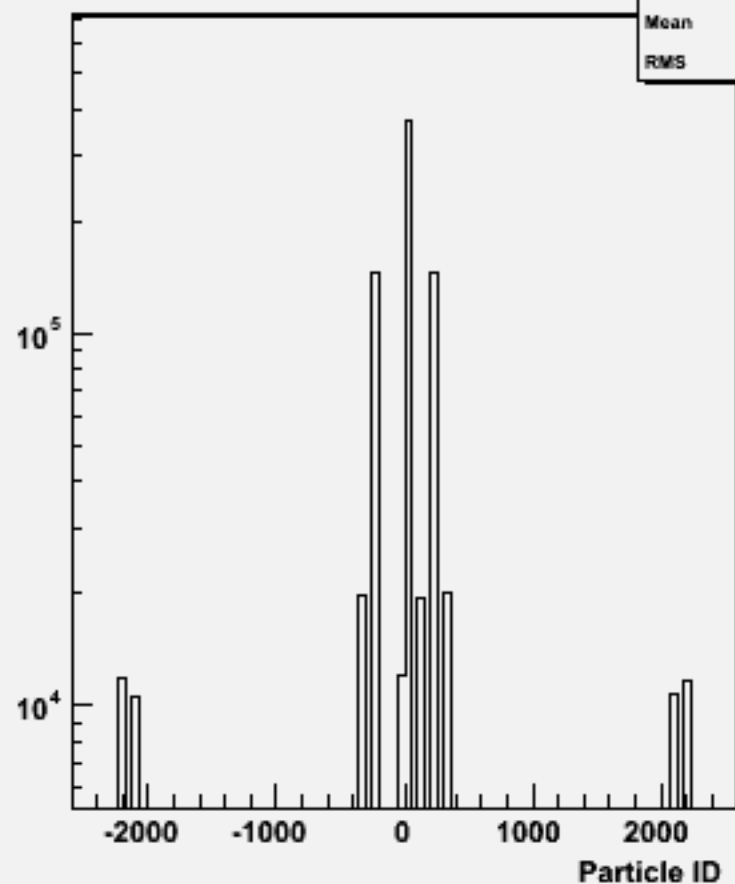
Particle ID : w101957 n1n1uuss_o
