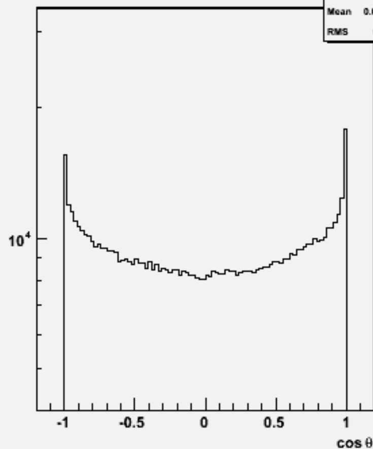
Particle cos \theta : w101957 n1n1uuss_o
