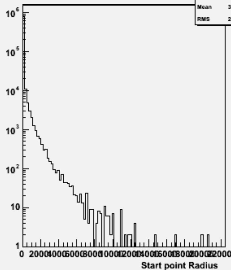
Start point R : w101956 n1n1uuss_o
