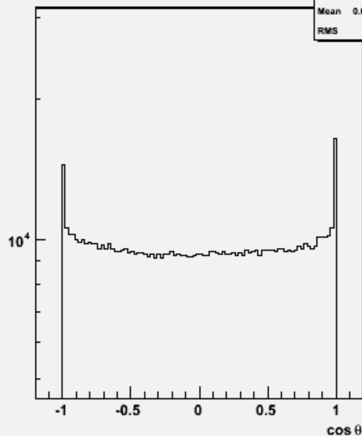
Particle cos \theta : w101956 n1n1uuss_o
