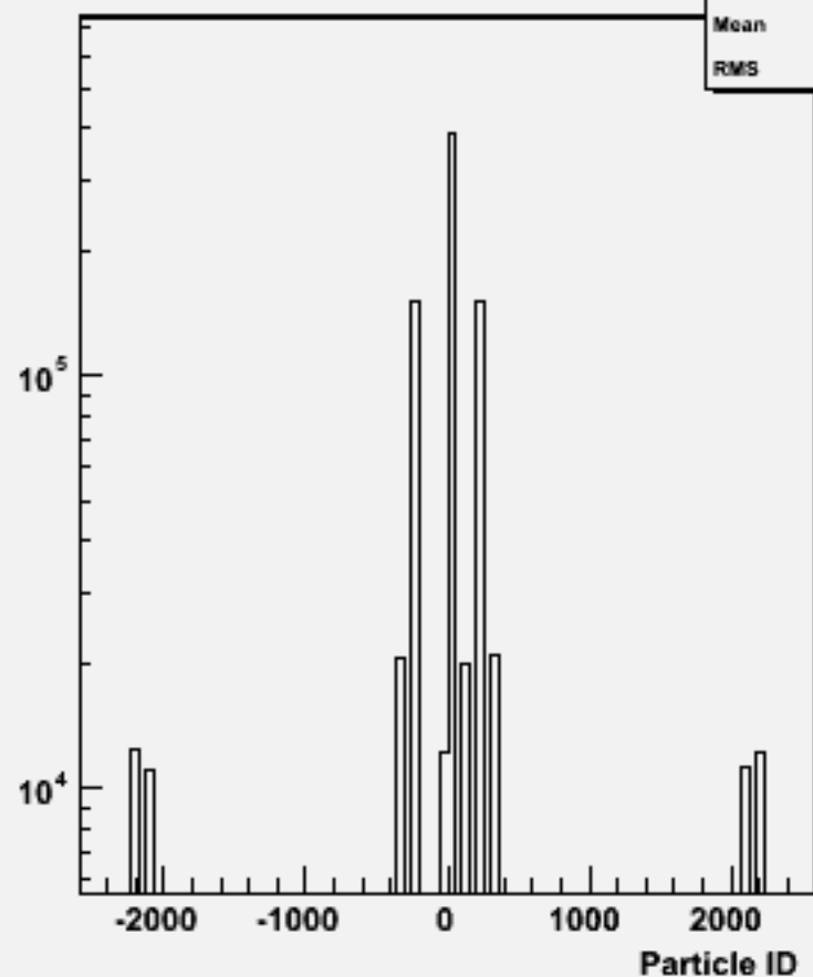
Particle ID : w101956 n1n1uuss_o
