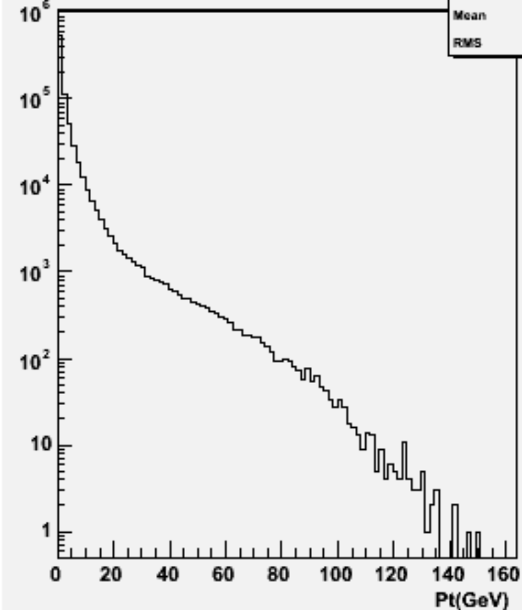
Particle Pt : w101956 n1n1uuss_o
