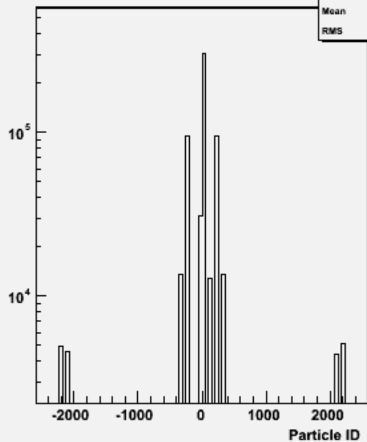
Particle ID : w101944 n1n1n3n3bb_o
