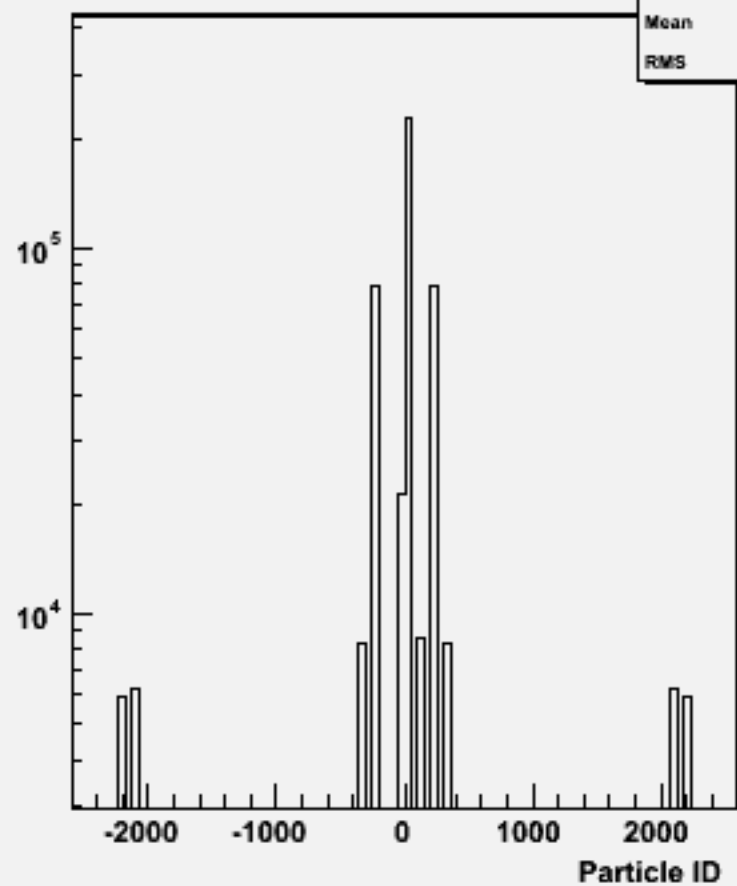
Particle ID : w101937 n1n1n3n3dd_o
