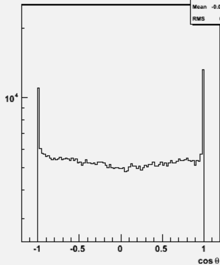
Particle cos \theta : w101937 n1n1n3n3dd_o
