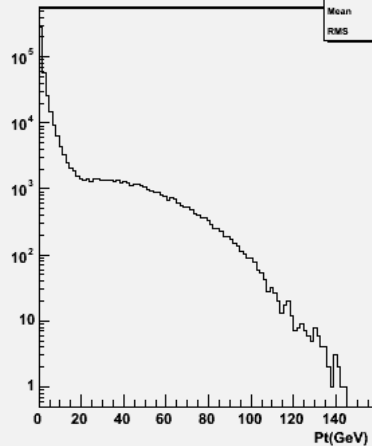
Particle Pt : w101937 n1n1n3n3dd_o
