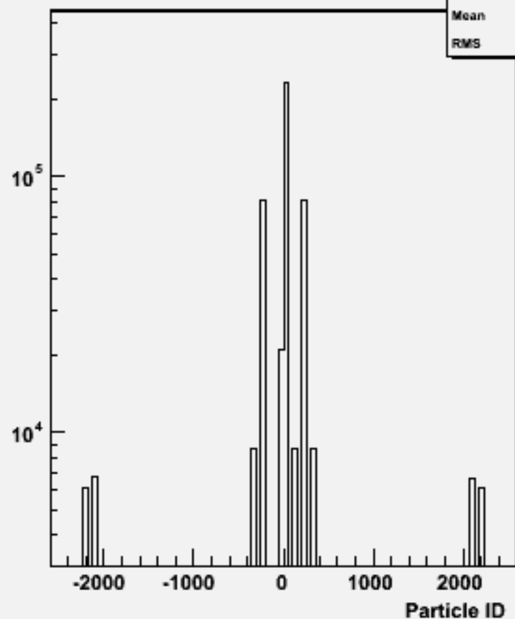
Particle ID : w101936 n1n1n3n3dd_o
