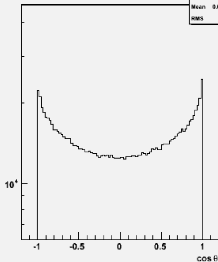
Particle cosθ : w101892 ccccccc_o
