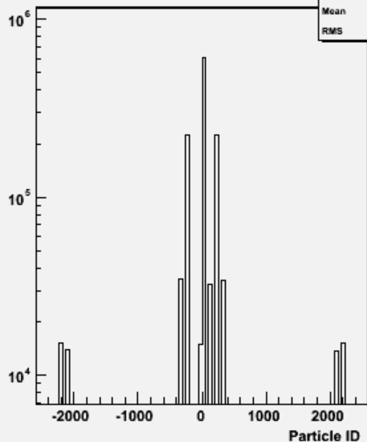
Particle ID : w101892 ccccccc_o
