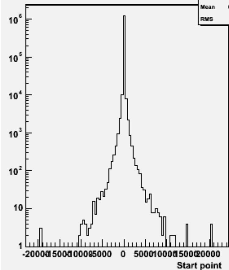
Start point Z : w101892 ccccccc_o
