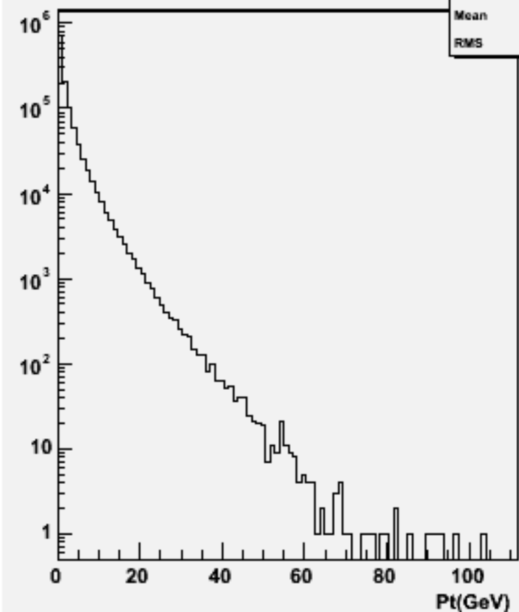
Particle Pt : w101892 ccccccc_o
