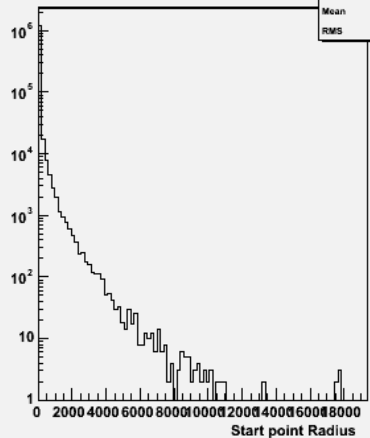
Start point R : w101892 ccccccc_o
