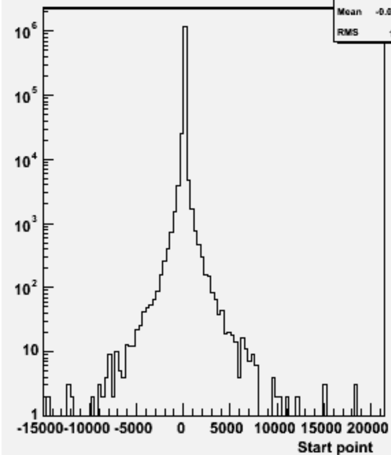
Start point Z : w101888 uucccc_o
