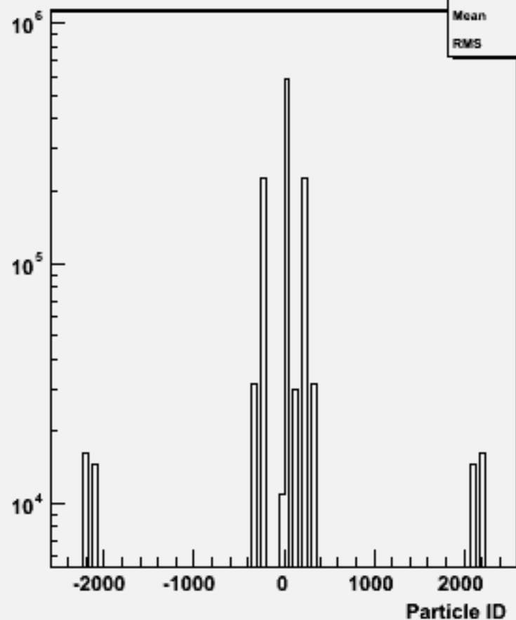
Particle ID : w101888 uucccc_o
