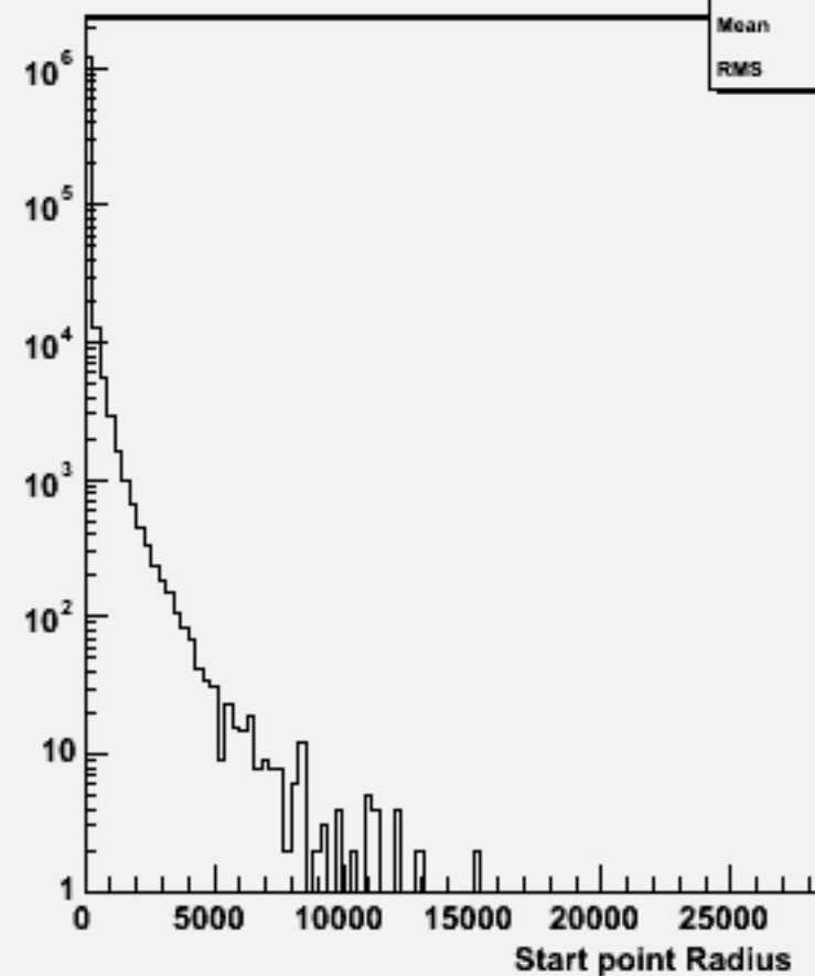
Start point R : w101888 uucccc_o
