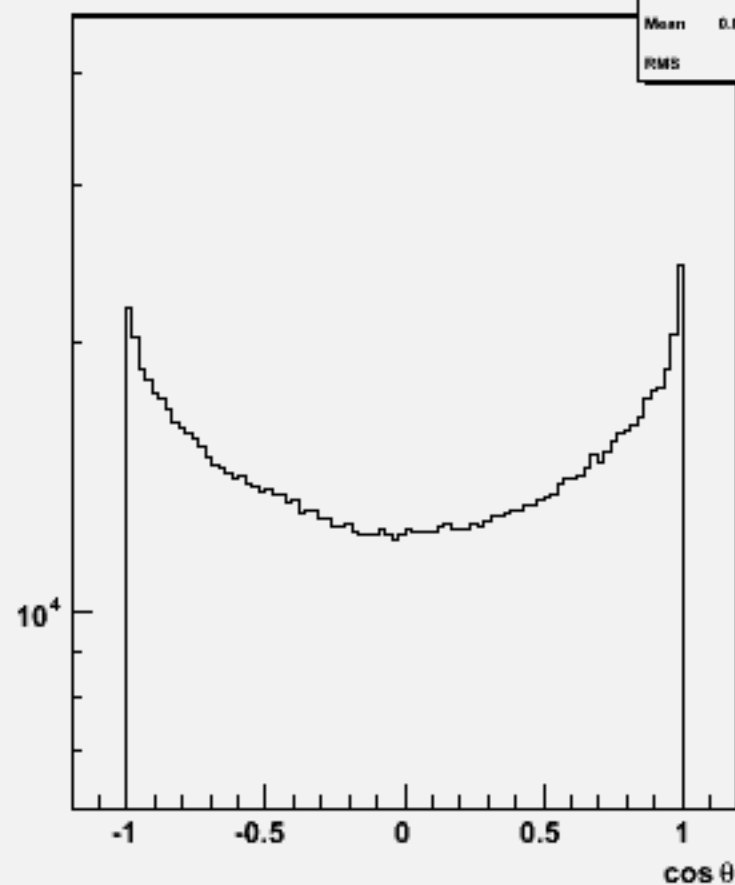
Particle cosθ : w101888 uucccc_o
