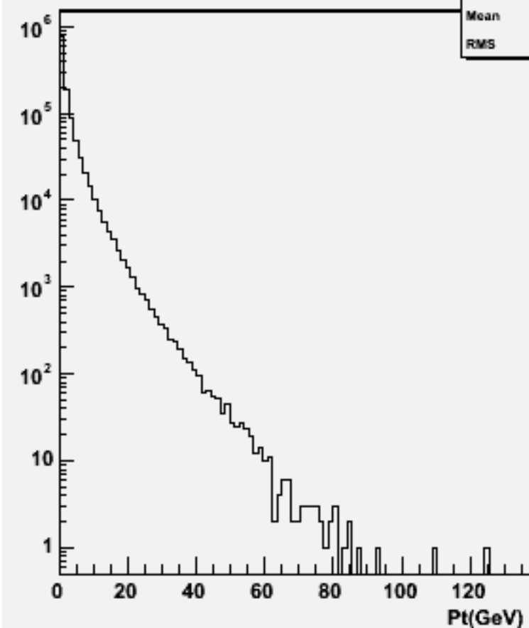
Particle Pt : w101888 uucccc_o
