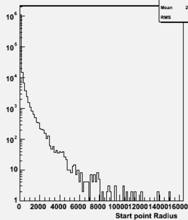
Start point R : w101885 uuucc_o
