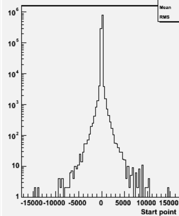
Start point Z : w101885 uuucc_o
