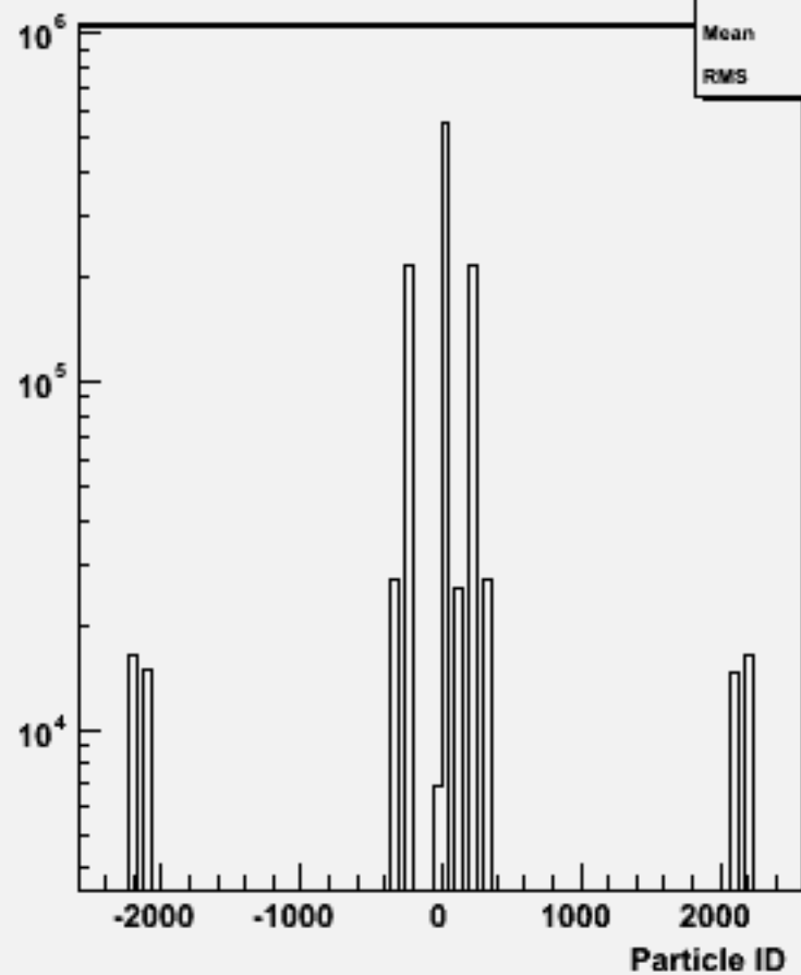
Particle ID : w101885 uuucc_o
