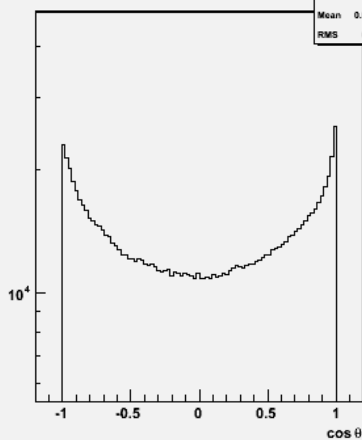
Particle cosθ : w101885 uuucc_o
