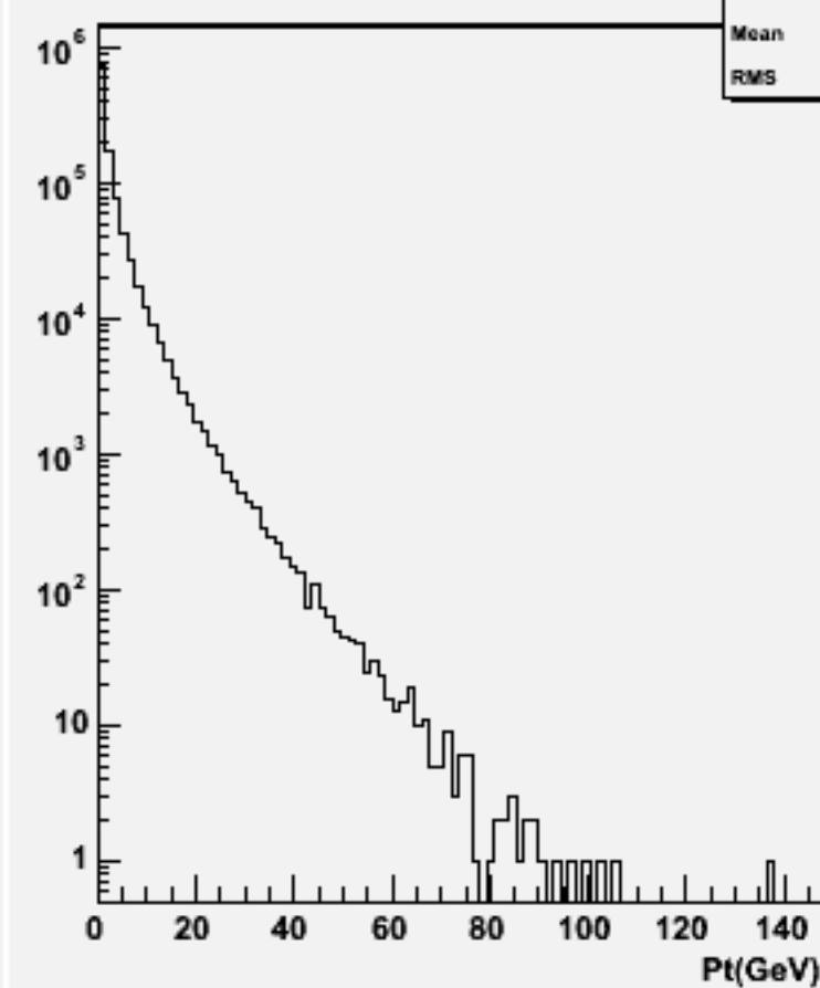
Particle Pt : w101885 uuucc_o
