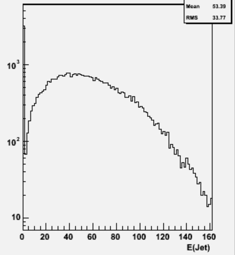
Jet energies(All jets)w101877 n3n3cccc_o
