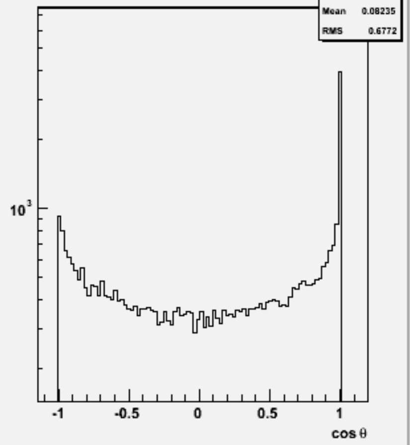
Jet cosθ (All jets)w101877 n3n3cccc_o
