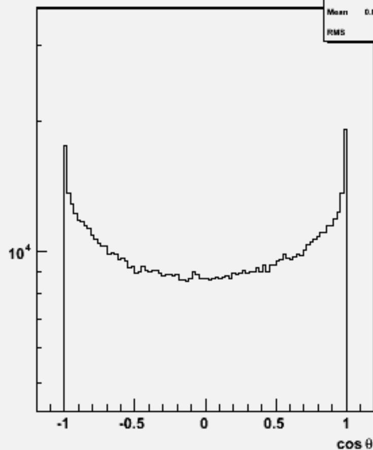
Particle cos \theta : w101876 n3n3cccc_o
