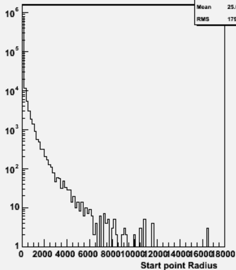
Start point R : w101876 n3n3cccc_o
