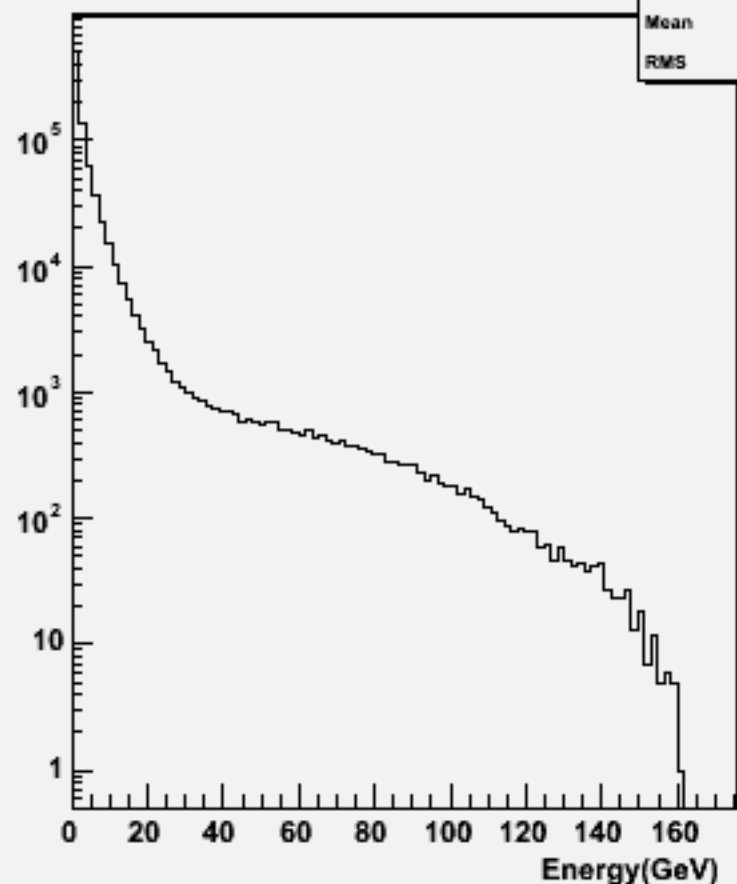
Particle Energy : w101876 n3n3cccc_o
