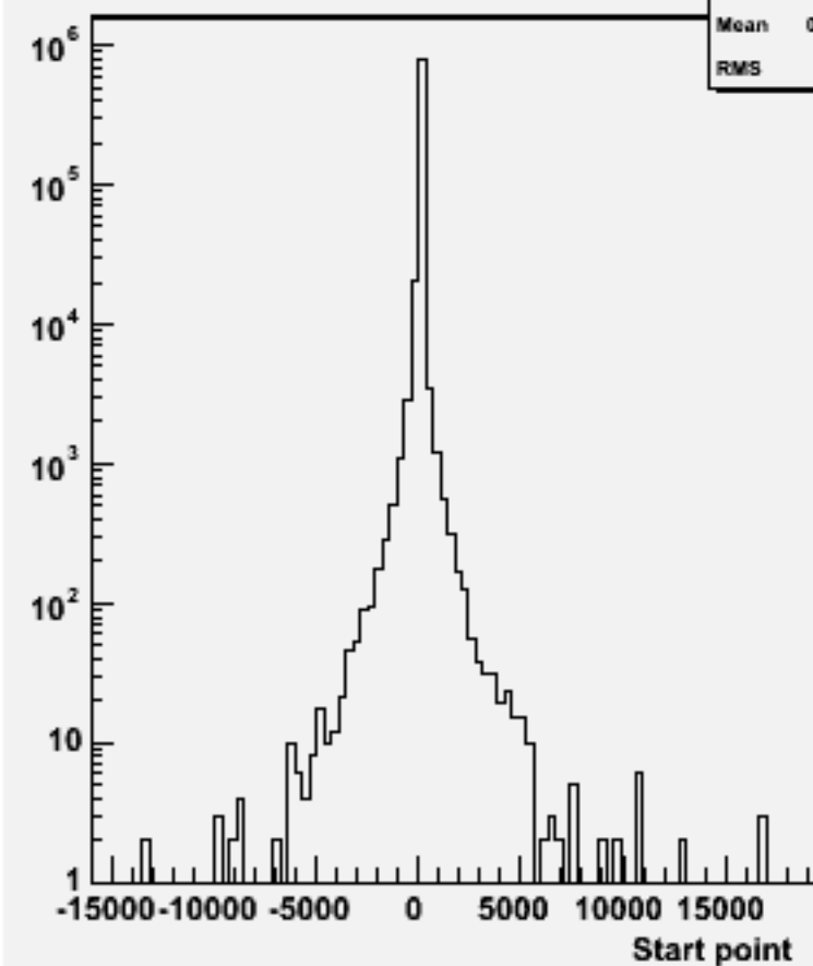
Start point Z : w101876 n3n3cccc_o
