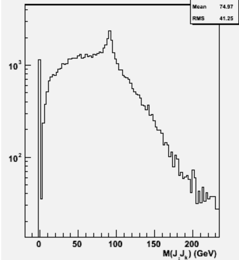
2jets mass(All comb)w101876 n3n3cccc_o
