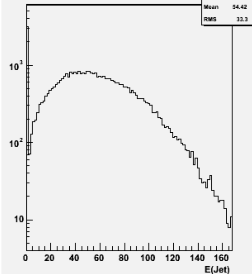
Jet energies(All jets)w101876 n3n3cccc_o
