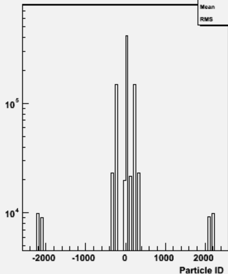
Particle ID : w101876 n3n3cccc_o
