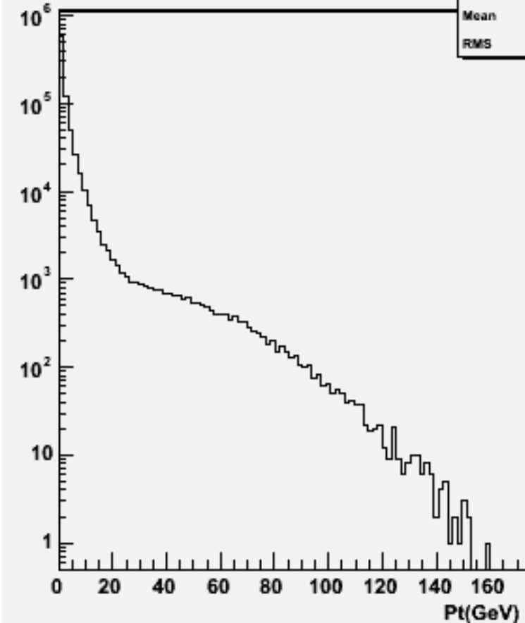
Particle Pt : w101876 n3n3cccc_o
