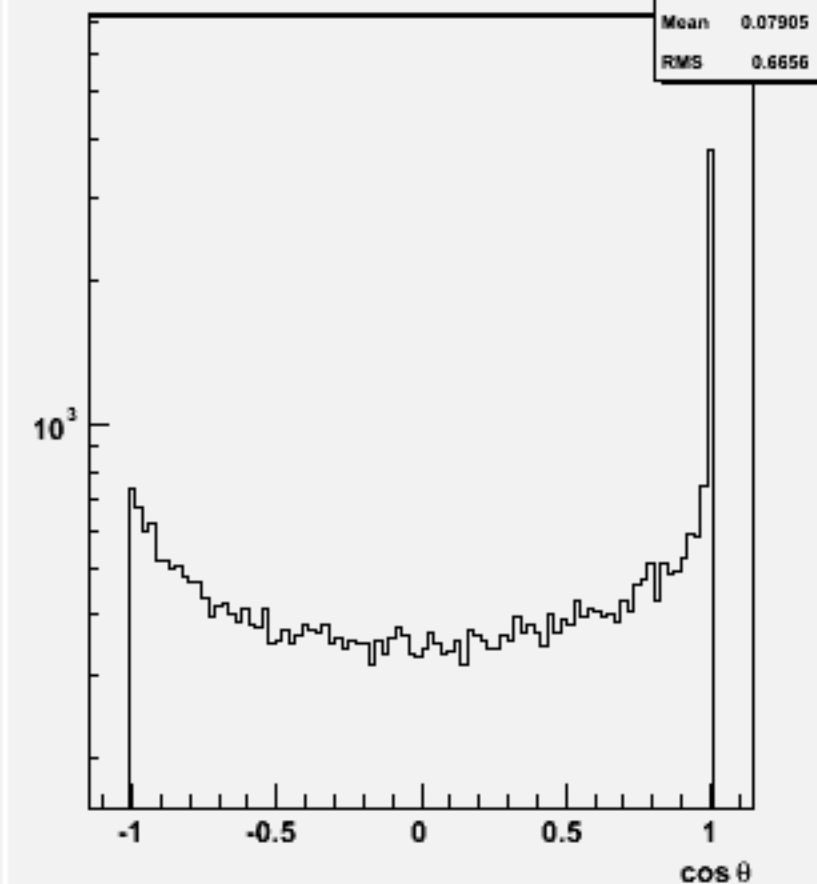
Jet cos \theta (All jets)w101876 n3n3cccc_o
