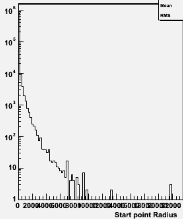
Start point R : w101872 n3n3uucc_o
