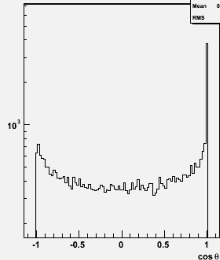
Jet cos \theta (All jets)w101872 n3n3uucc_o
