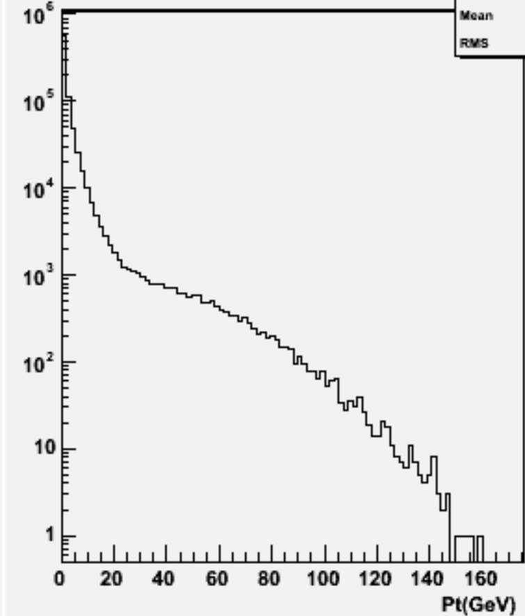
Particle Pt : w101872 n3n3uucc_o
