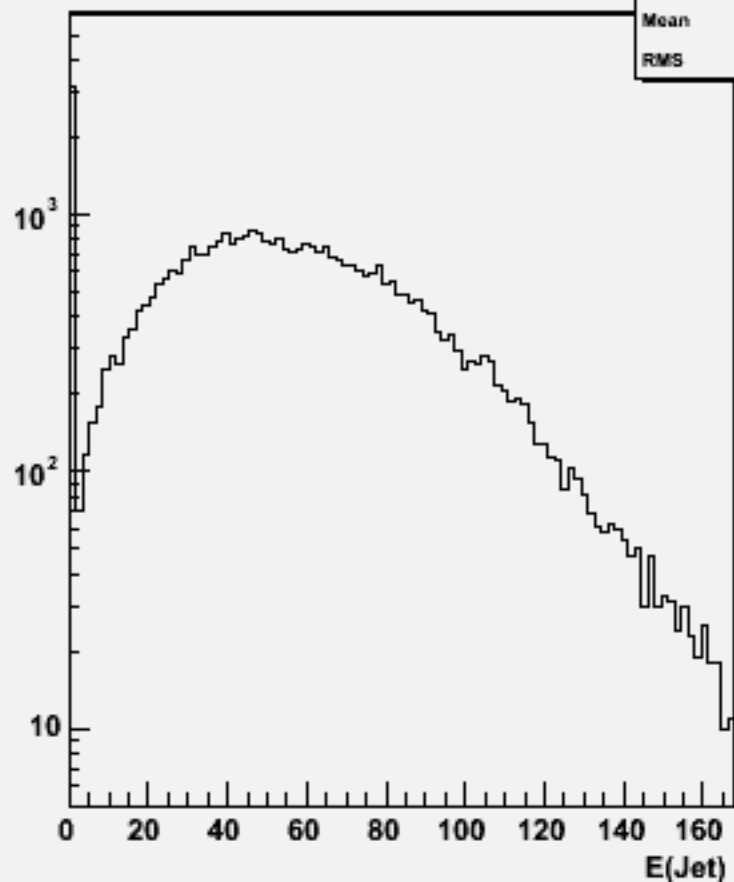
Jet energies(All jets)w101872 n3n3uucc_o
