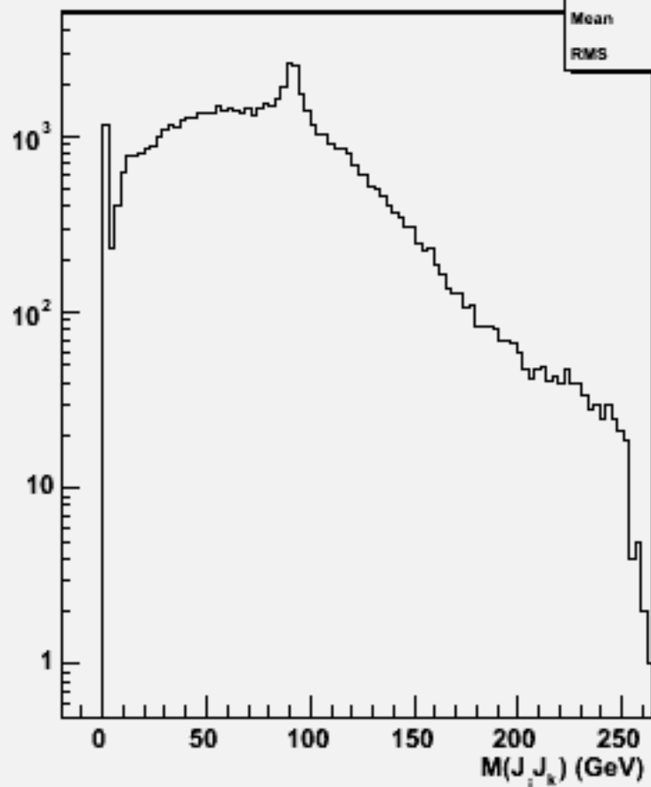
2jets mass(All comb)w101872 n3n3uucc_o
