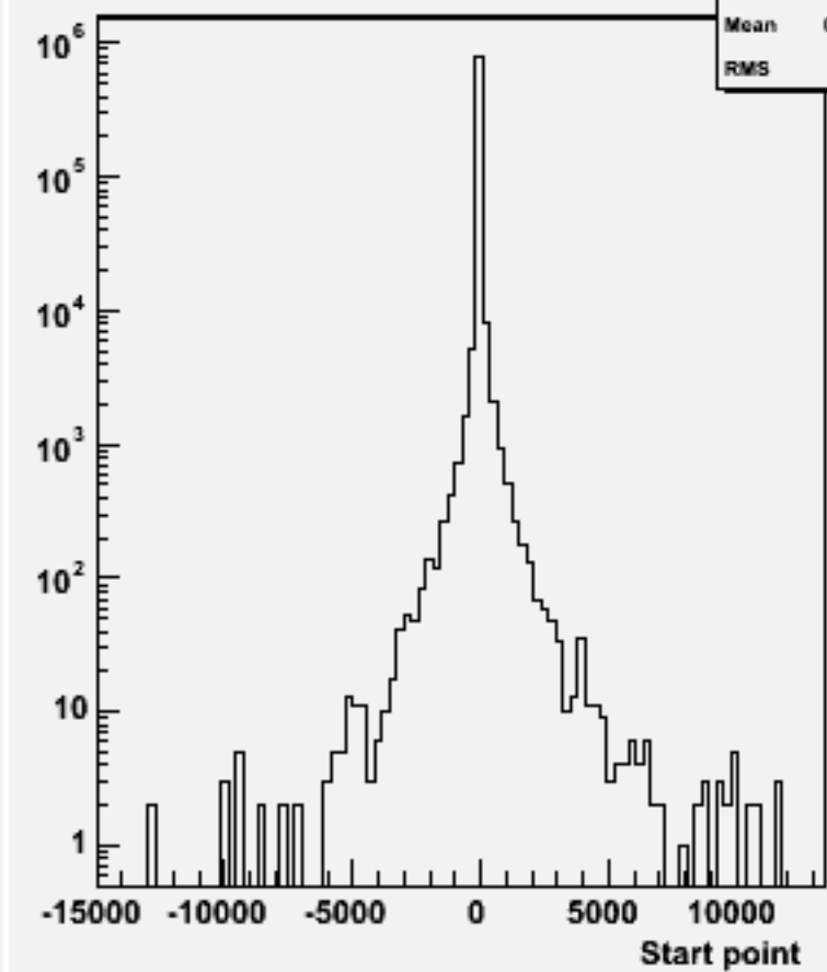
Start point Z : w101872 n3n3uucc_o
