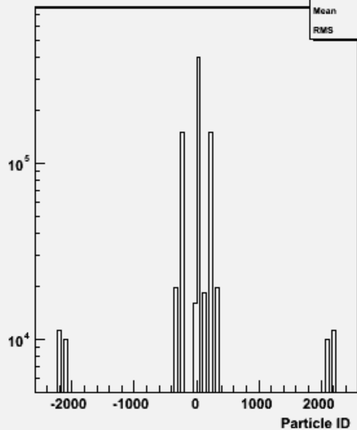
Particle ID : w101872 n3n3uucc_o
