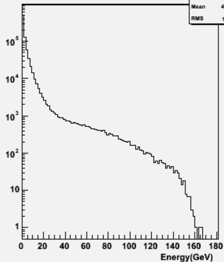
Particle Energy : w101872 n3n3uucc_o
