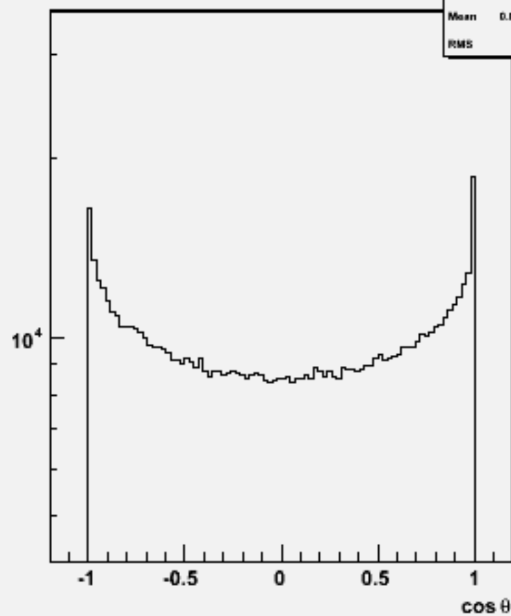
Particle cos \theta : w101872 n3n3uucc_o
