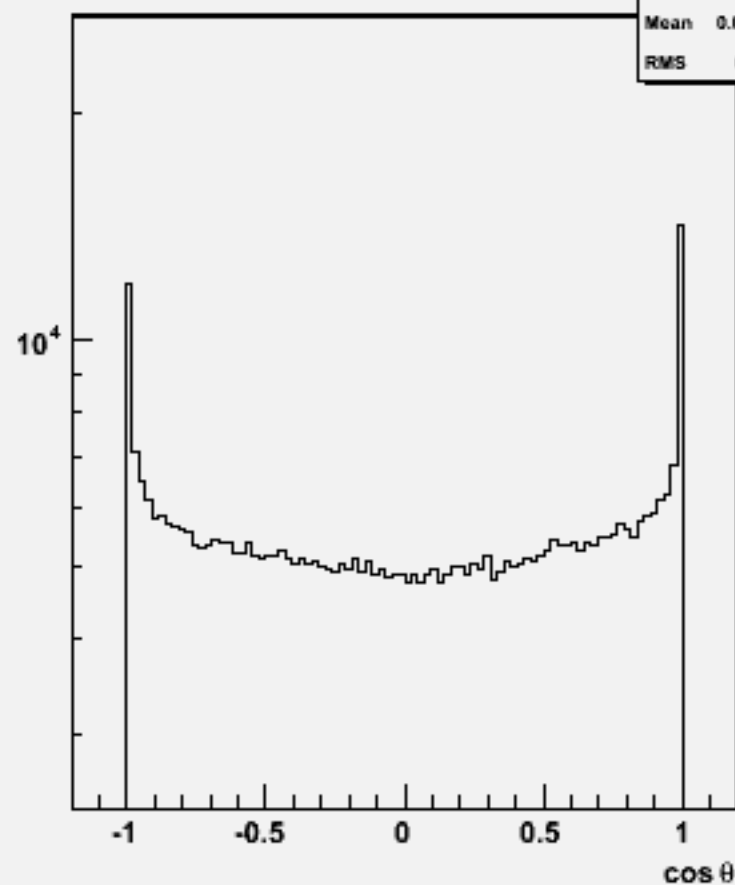
Particle cosθ : w101864 n3n3n3n3cc_o
