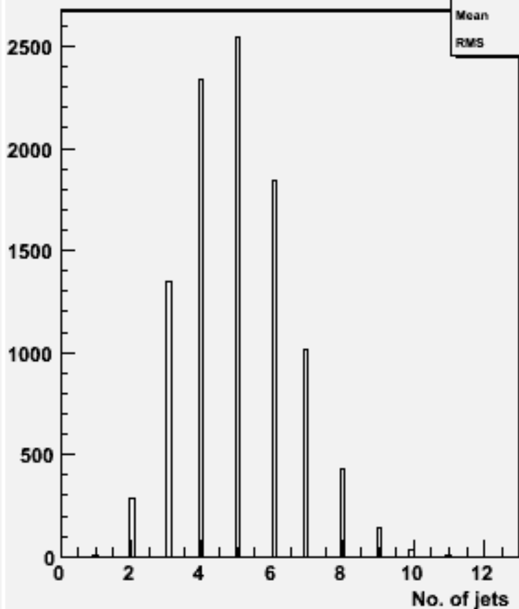
No. jets (ycut=0.001) : w101864 n3n3n3n3cc_o
