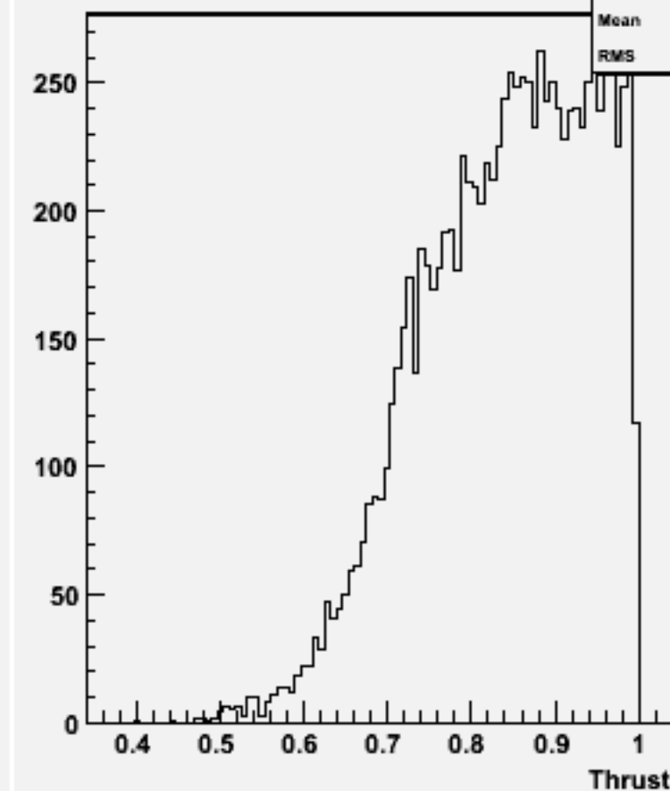
Thrust w101864 n3n3n3n3cc_o
