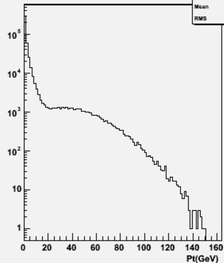
Start point Z : w101864 n3n3n3n3cc_o
