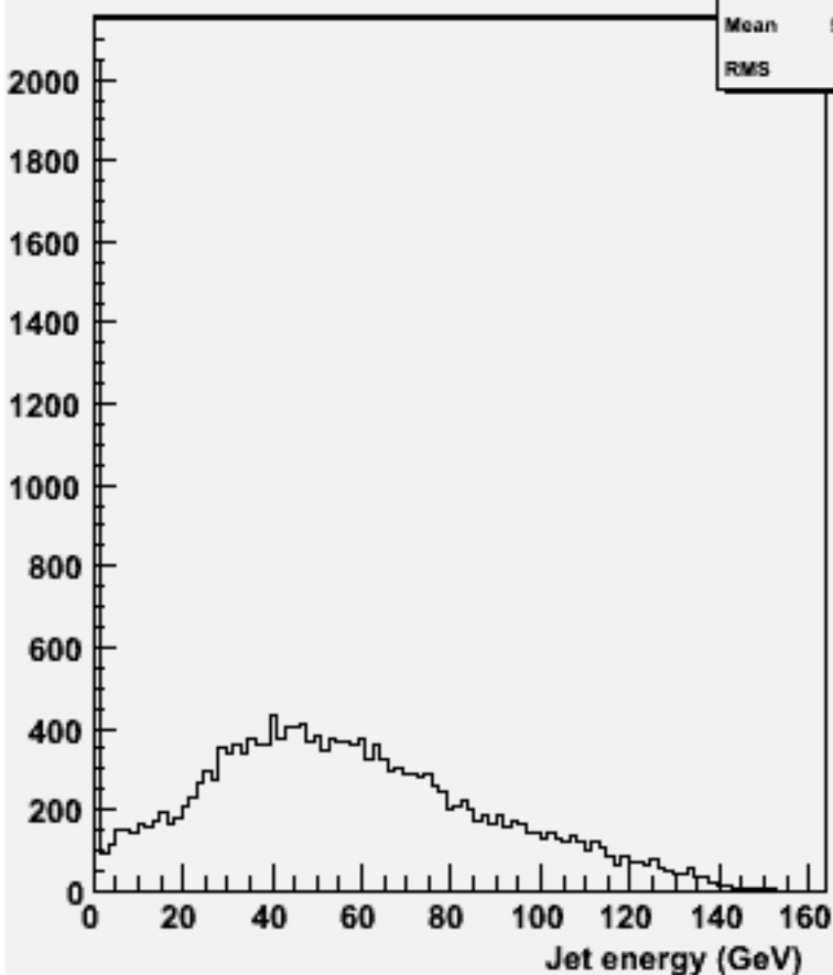
energy for 2-jets :w101864 n3n3n3n3cc_o
