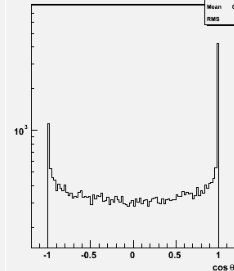
Jet cos \theta (All jets)w101864 n3n3n3n3cc_o
