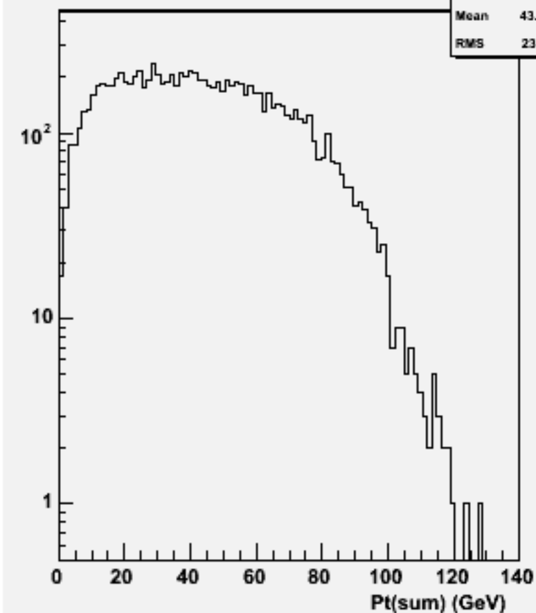
Pt Sum: w101864 n3n3n3n3cc_o
