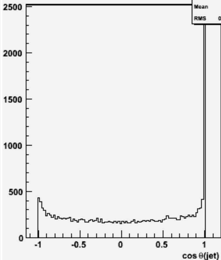
cos \theta for 2-jets :w101864 n3n3n3n3cc_o
