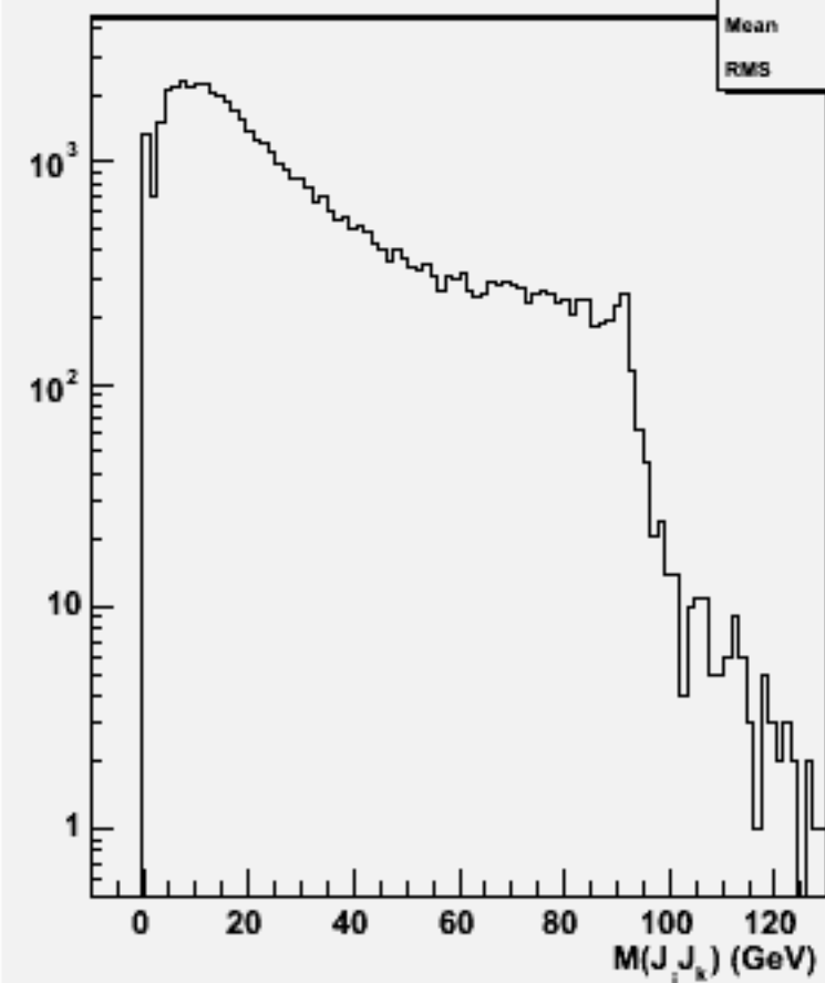
2jets mass(All comb)w101864 n3n3n3n3cc_o
