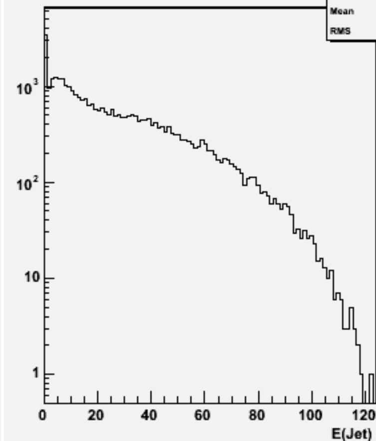
Jet energies(All jets)w101864 n3n3n3n3cc_o
