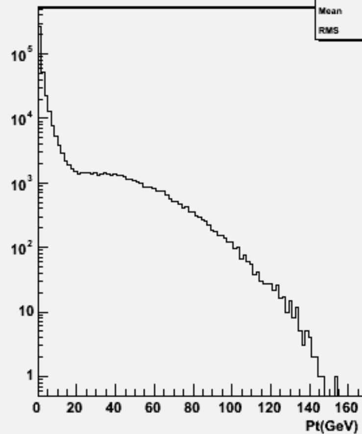
Particle Pt : w101860 n3n3n3n3uu_o
