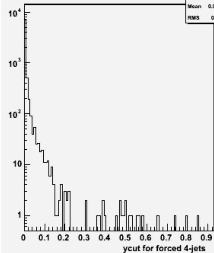
Ycut for 4-jets :w101860 n3n3n3n3uu_o
