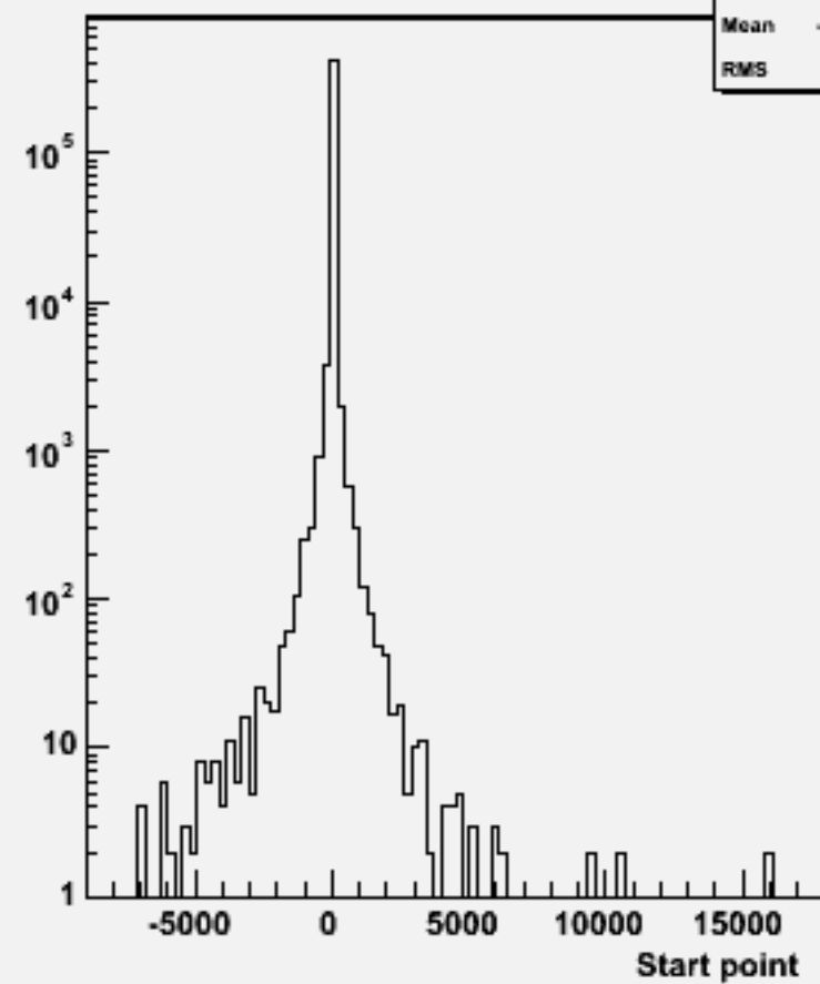
Start point Z : w101860 n3n3n3n3uu_o
