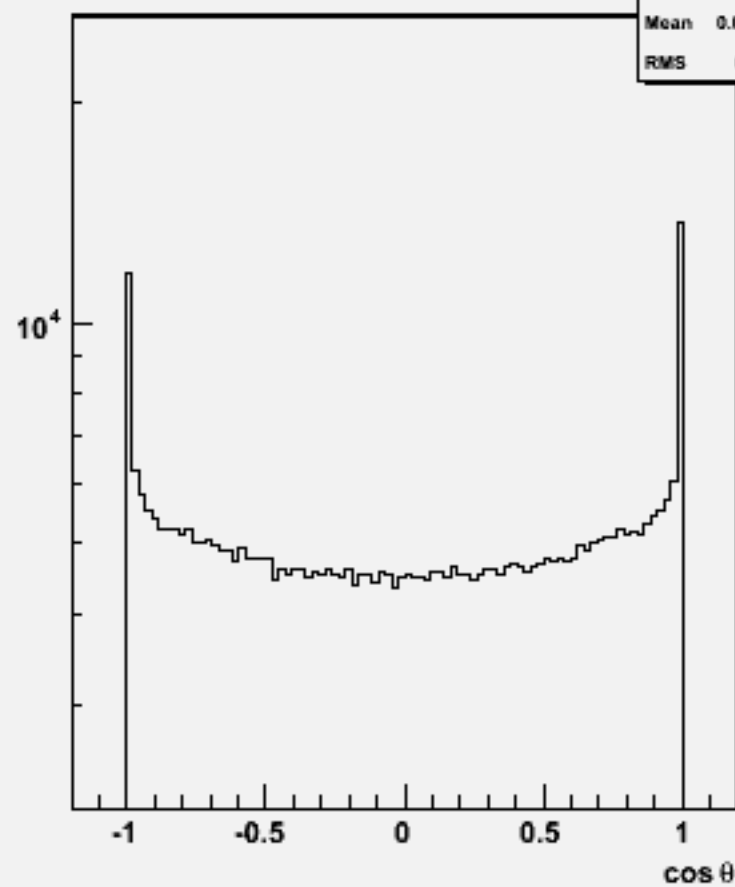
Particle cosθ : w101860 n3n3n3n3uu_o
