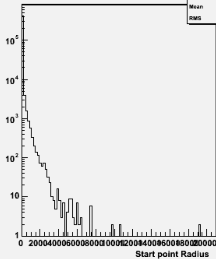
Start point R : w101860 n3n3n3n3uu_o
