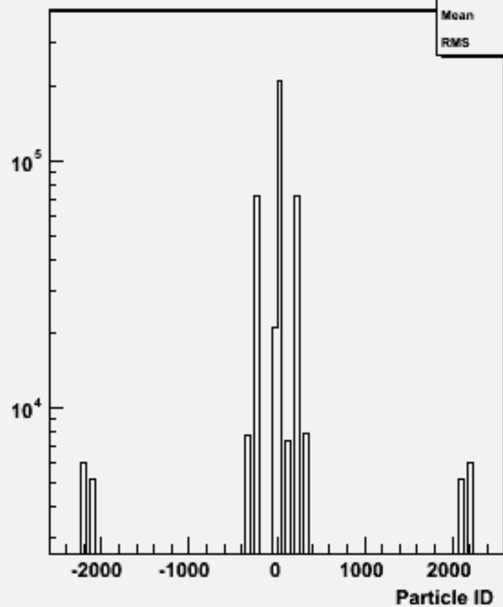
Particle ID : w101860 n3n3n3n3uu_o
