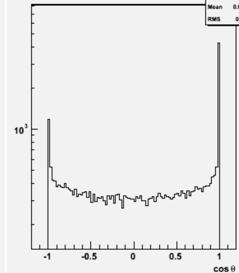
Jet cos \theta (All jets)w101860 n3n3n3n3uu_o
