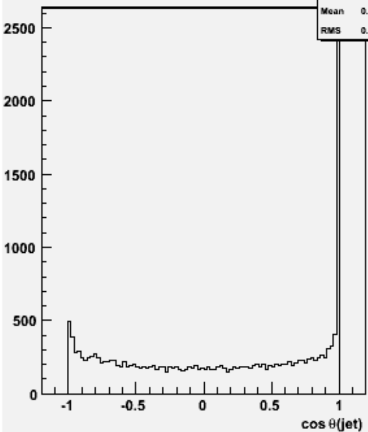
cos \theta for 2-jets :w101860 n3n3n3uu_o
