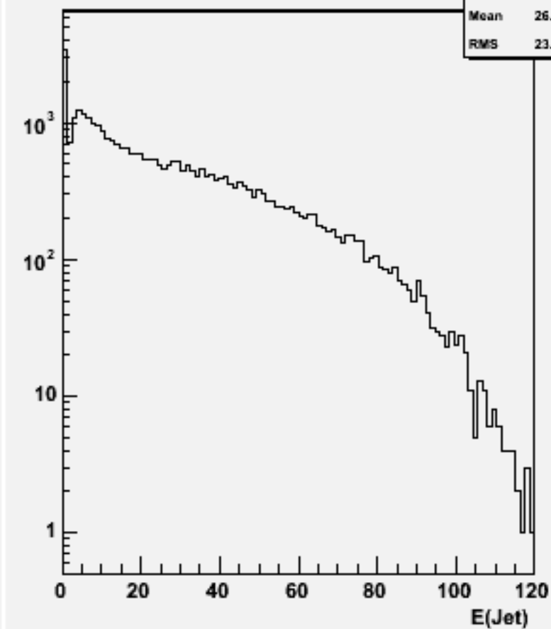
Jet energies(All jets)w101860 n3n3n3n3uu_o
