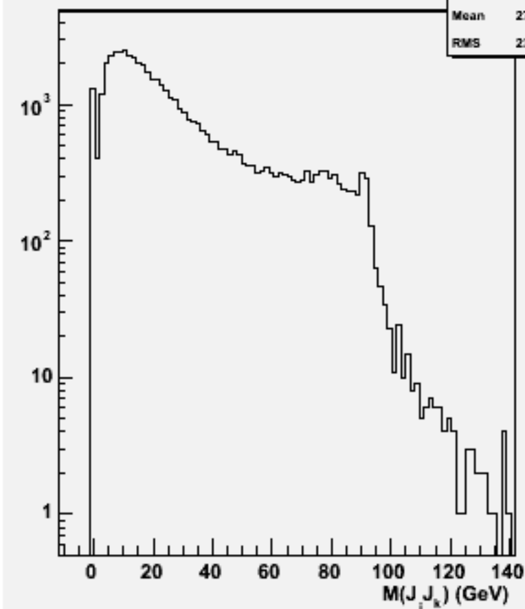
2jets mass(All comb)w101860 n3n3n3n3uu_o
