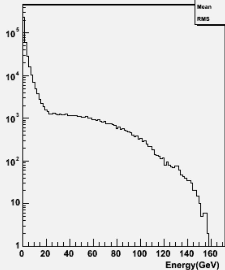
Particle Energy : w101860 n3n3n3n3uu_o
