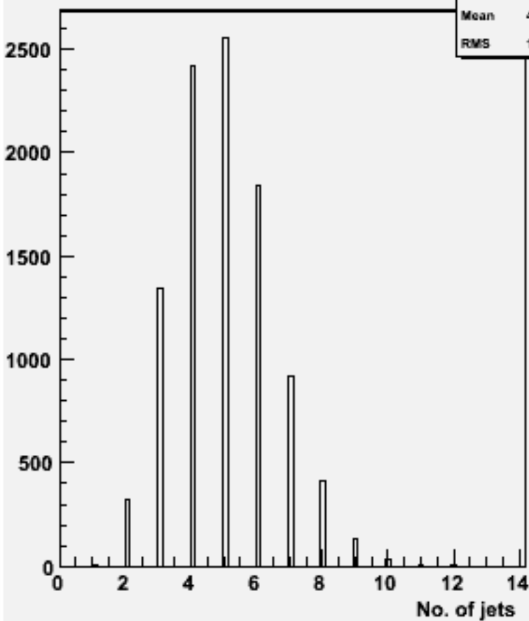
No. jets (ycut=0.001) : w101860 n3n3n3uu_o
