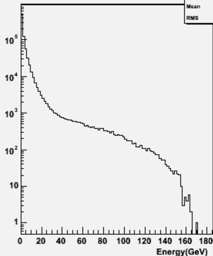
Particle Energy : w101853 n2n2uucc_o
