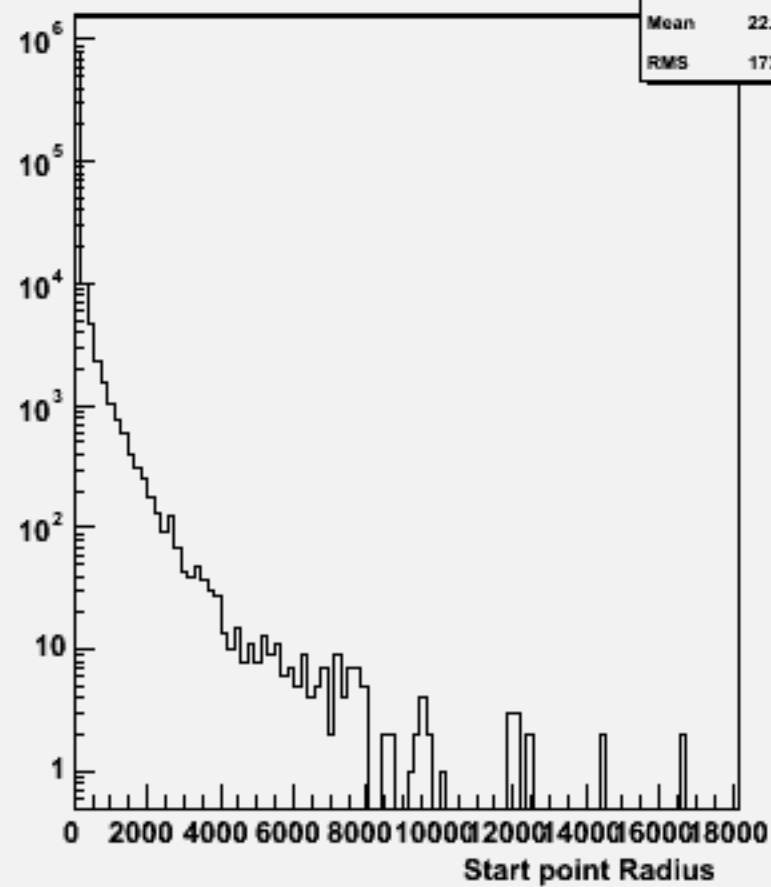
Start point R : w101852 n2n2uucc_o
