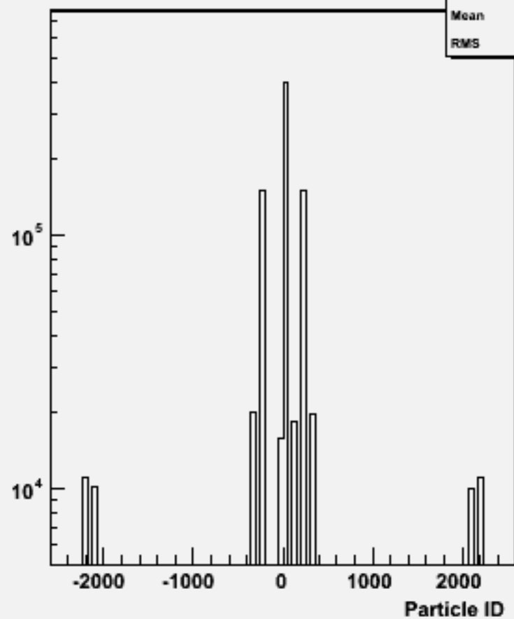
Particle ID : w101852 n2n2uucc_o
