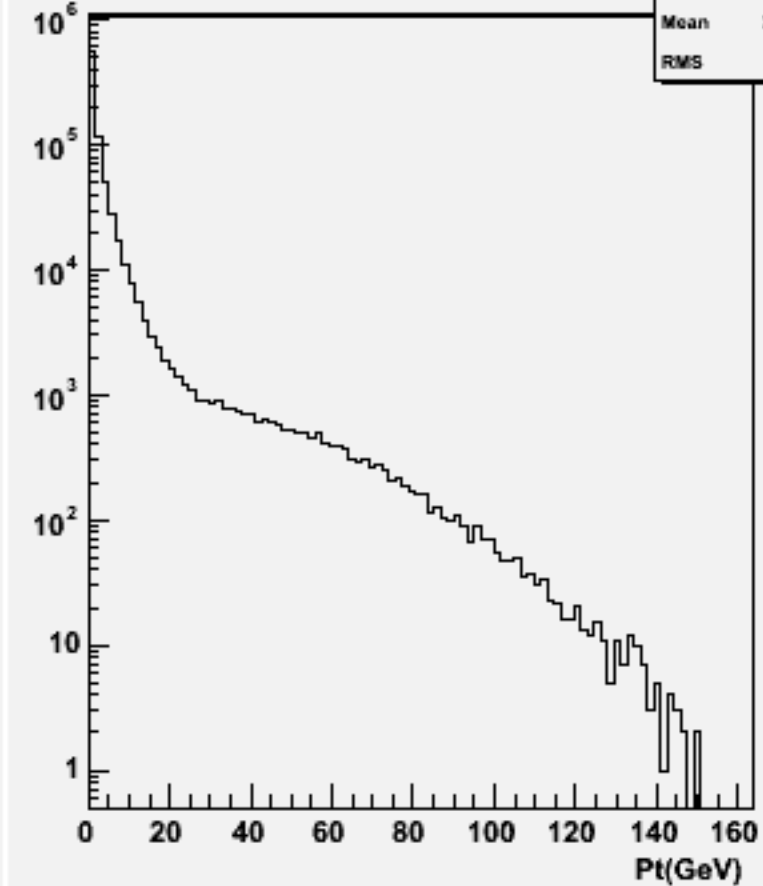
Particle Pt : w101852 n2n2uucc_o
