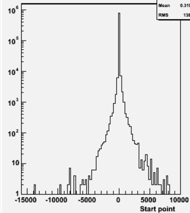
Start point Z : w101852 n2n2uucc_o
