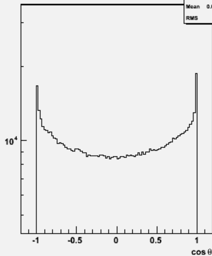
Particle cos \theta : w101852 n2n2uucc_o
