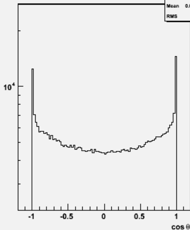
Particle cos \theta : w101817 n1n1n3n3cc_o
