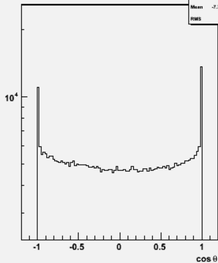
Particle cos \theta : w101812 n1n1n3n3uu_o
