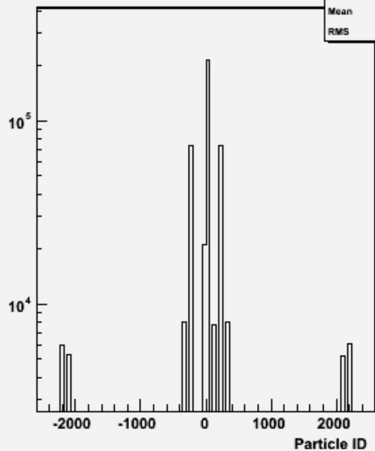
Particle ID : w101812 n1n1n3n3uu_o
