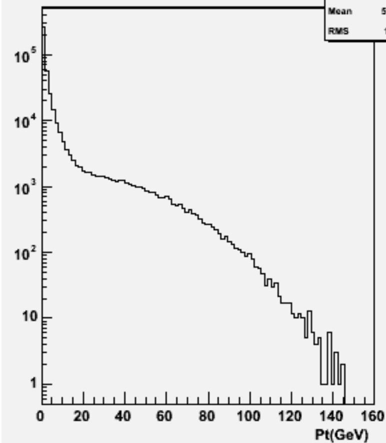
Particle Pt : w101812 n1n1n3n3uu_o
