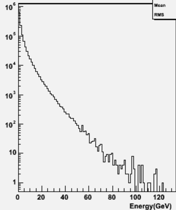
Start point R : w101793 cccssc_o
