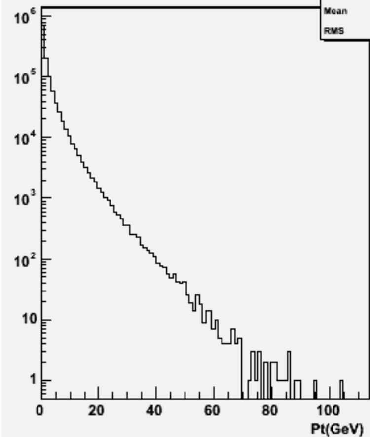
Start point Z : w101793 cccssc_o
