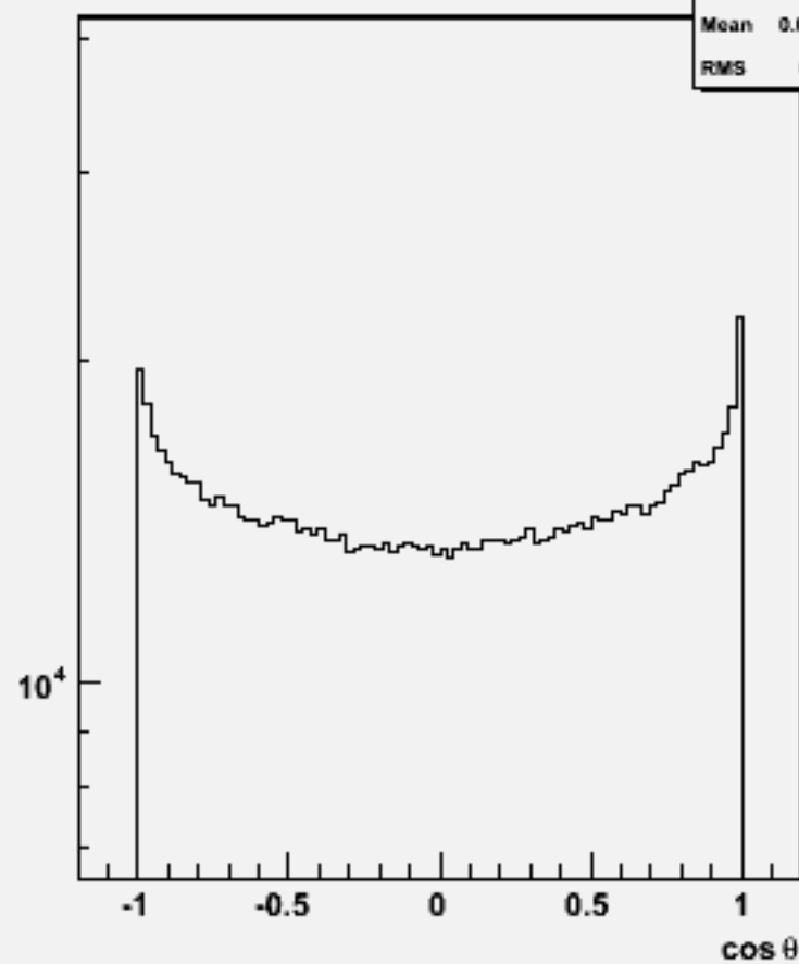
Particle cosθ : w101793 cccssc_o
