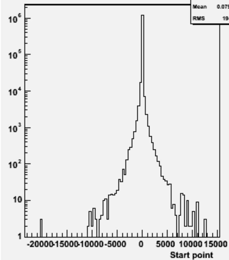
Start point Z : w101793 cccssc_o
