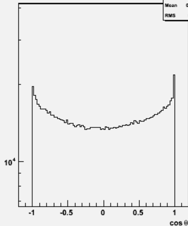
Particle cosθ : w101792 cccssc_o
