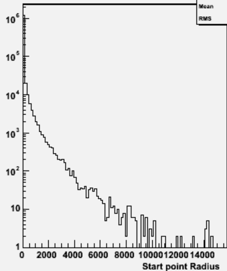
Start point R : w101792 cccssc_o
