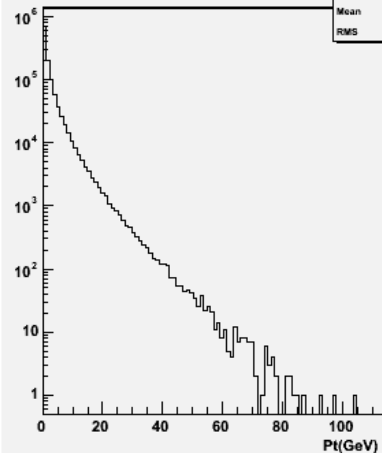
Particle Pt : w101789 cccsdu_o
