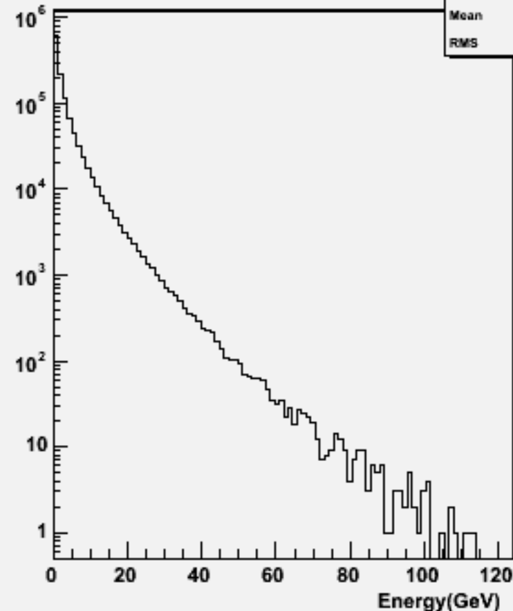
Particle Energy : w101789 cccsdu_o
