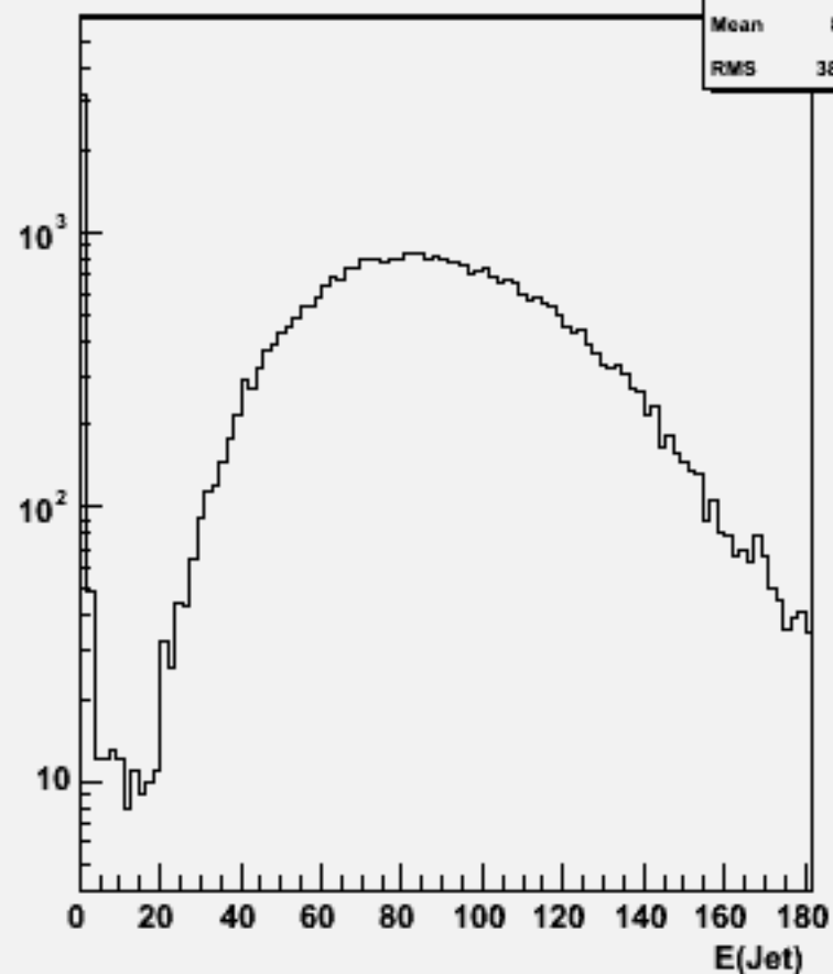
Jet energies(All jets)w101789 cccsdu_o
