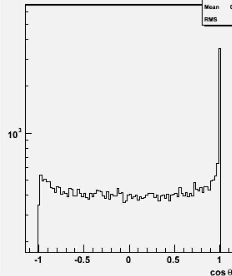
Jet cos \theta (All jets)w101789 cccsdu_o
