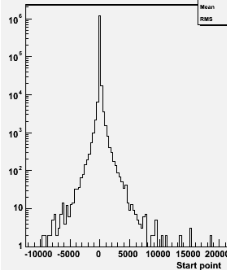
Start point Z : w101789 cccsdu_o
