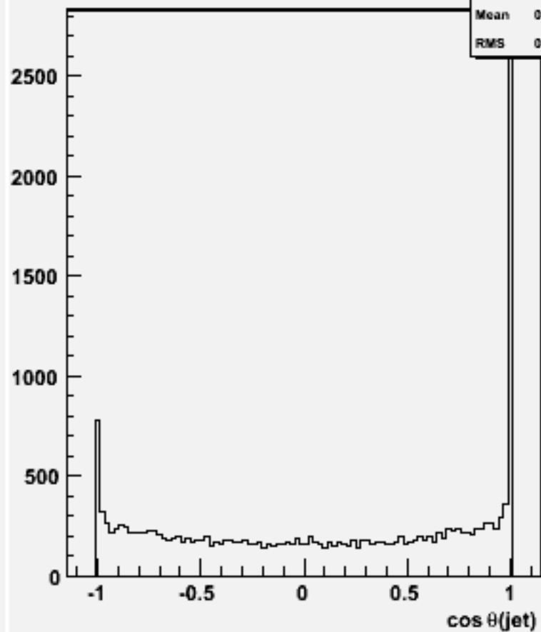
cos \theta for 2-jets :w101789 cccsdu_o
