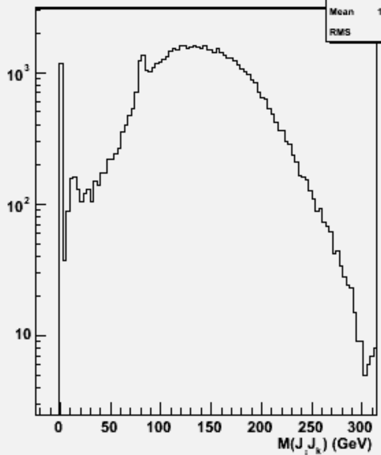
2jets mass(All comb)w101789 cccsdu_o
