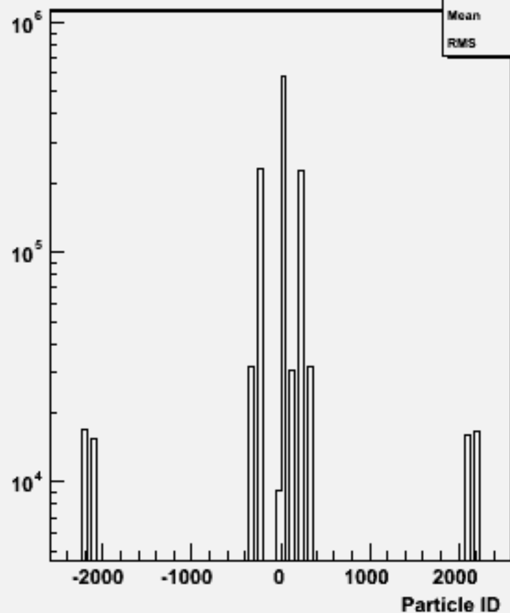
Particle ID : w101789 cccsdu_o
