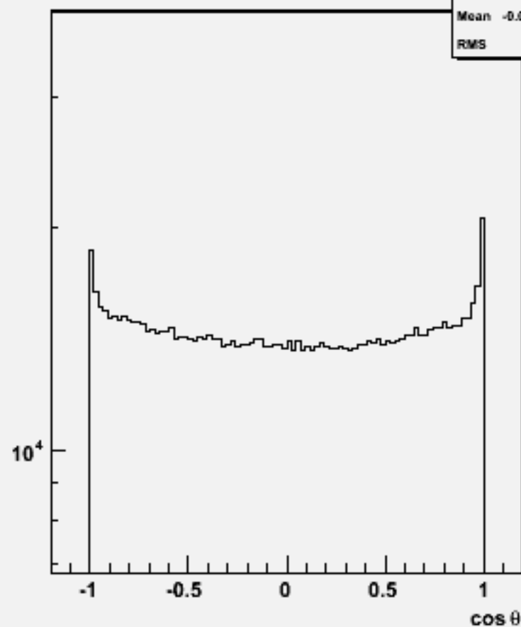
Particle cosθ : w101789 cccsdu_o
