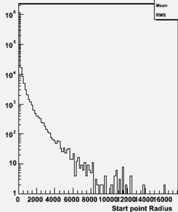
Start point R : w101789 cccsdu_o
