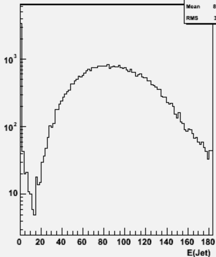
Jet energies(All jets)w101788 cccsdu_o
