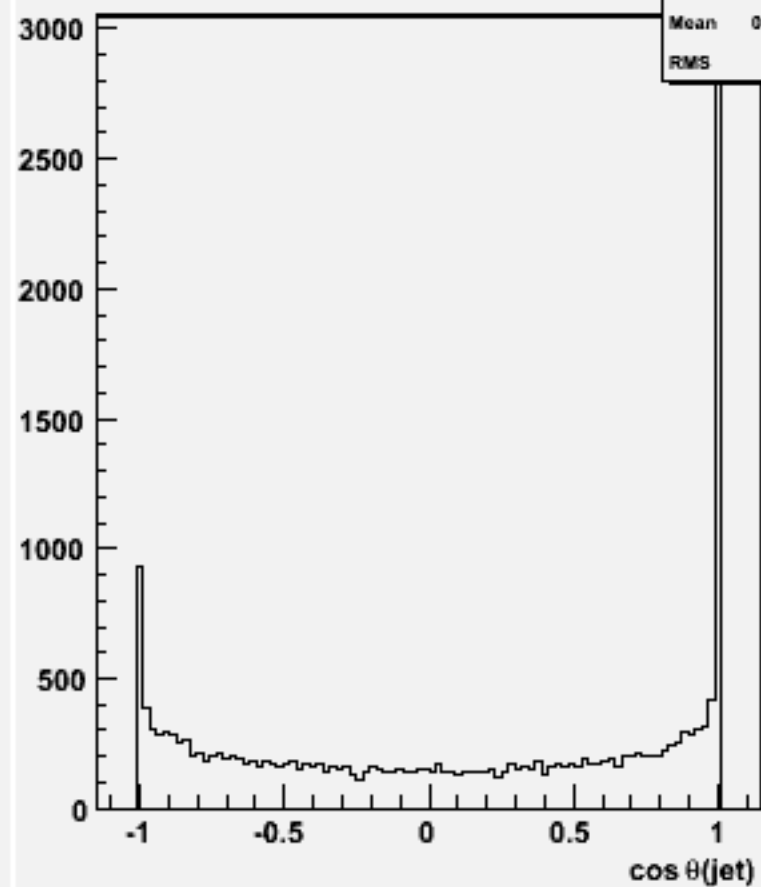
cos \theta for 2-jets :w101788 cccsdu_o
