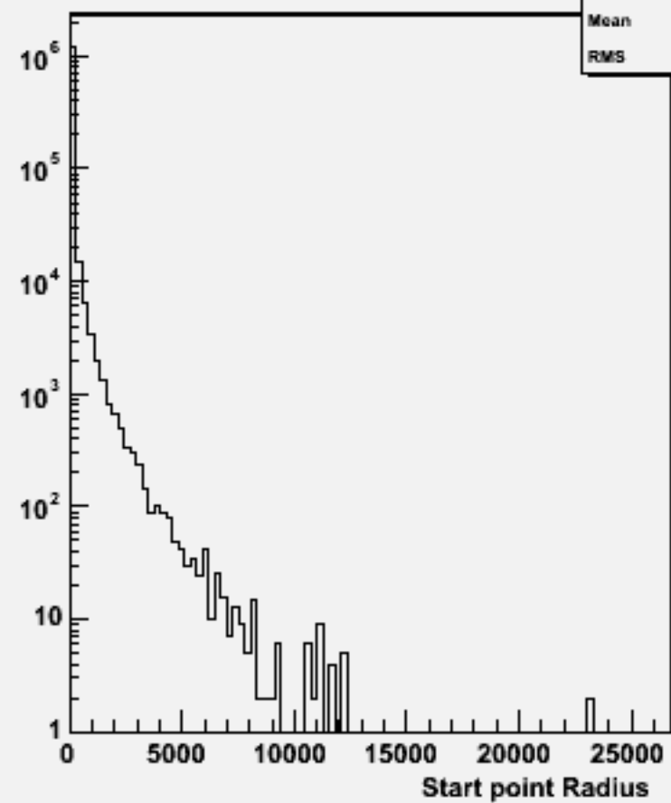
Start point R : w101788 cccsdu_o
