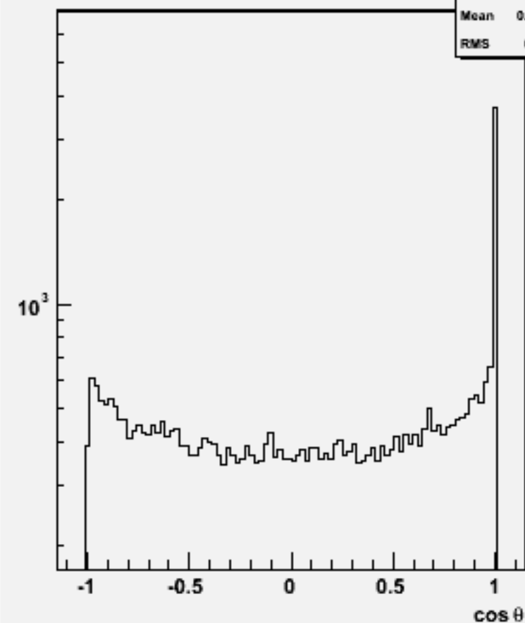
Jet cos \theta (All jets)w101788 cccsdu_o
