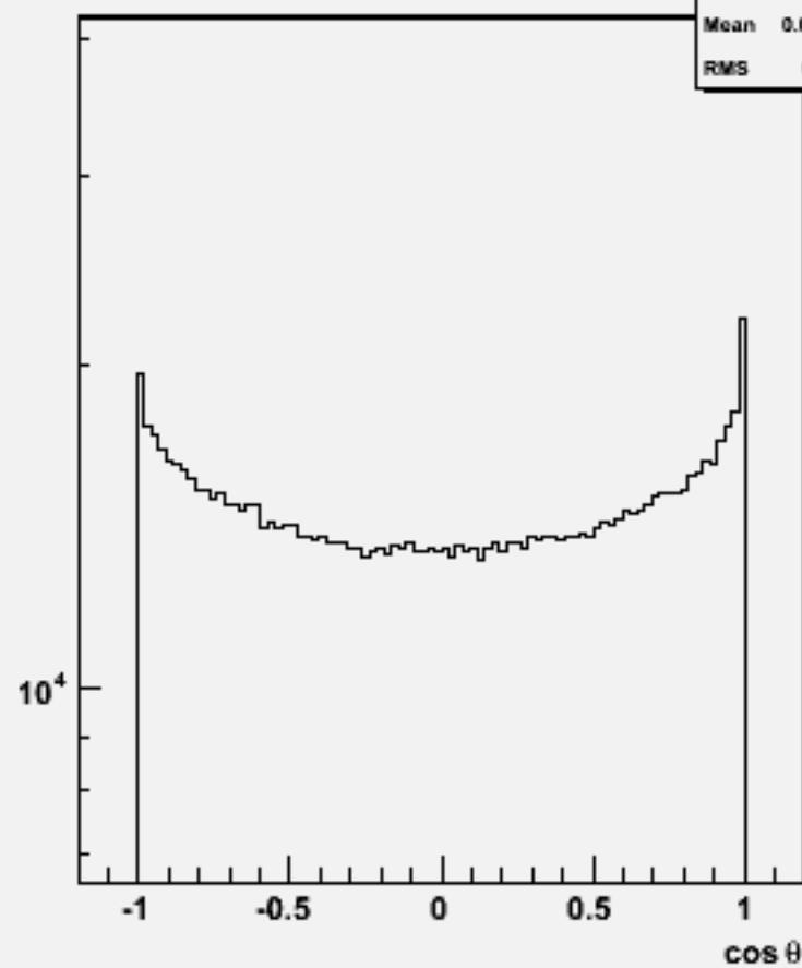
Particle cos \theta : w101788 cccsdu_o
