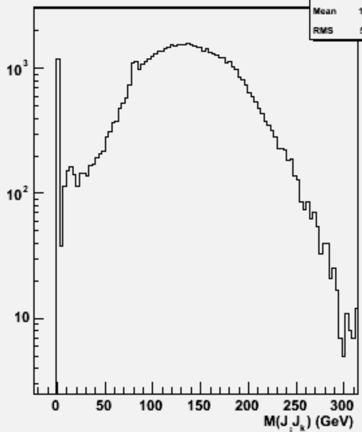
2jets mass(All comb)w101788 cccsdu_o
