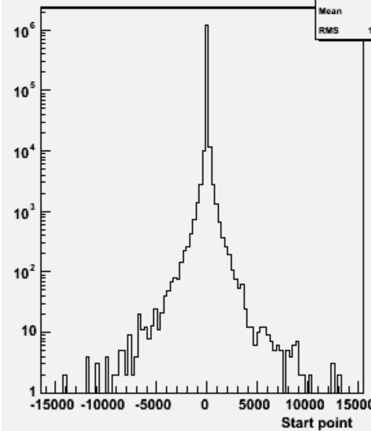
Start point Z : w101788 cccsdu_o
