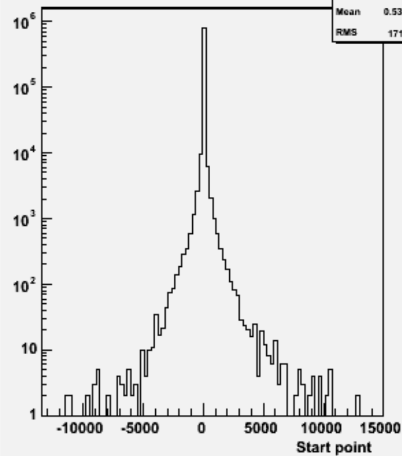
Start point Z : w101781 cccse2n2_o
