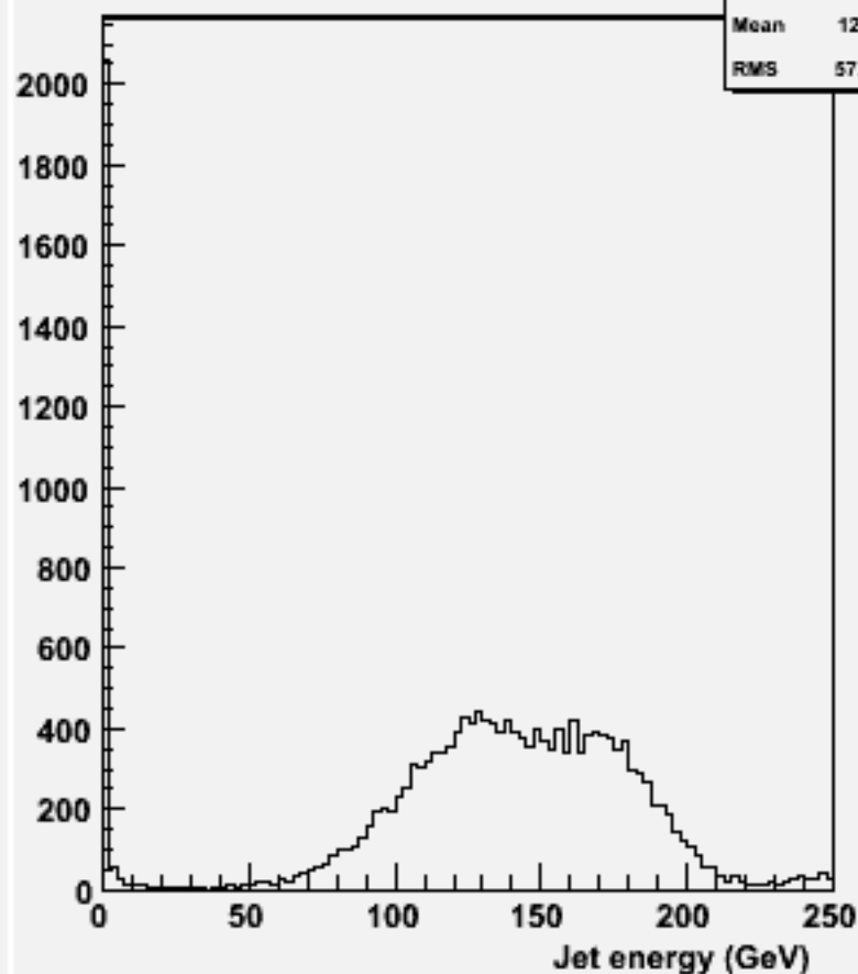
energy for 2-jets :w101781 cccse2n2_o
