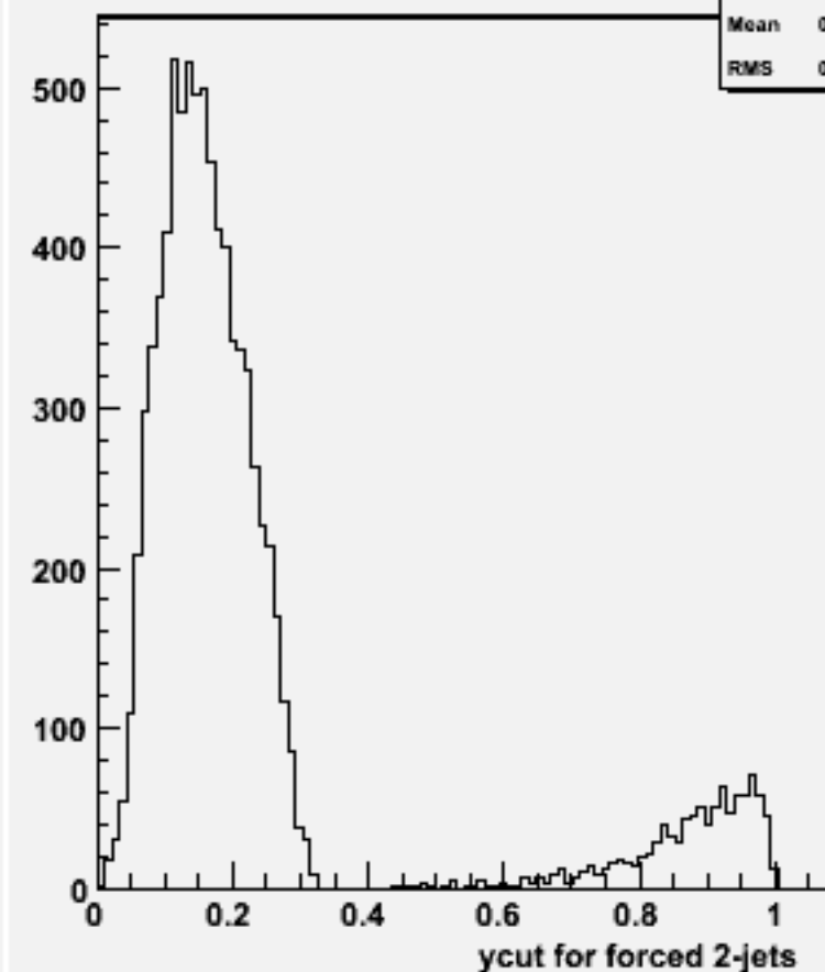
Ycut for 2-jets :w101781 cccse2n2_o
