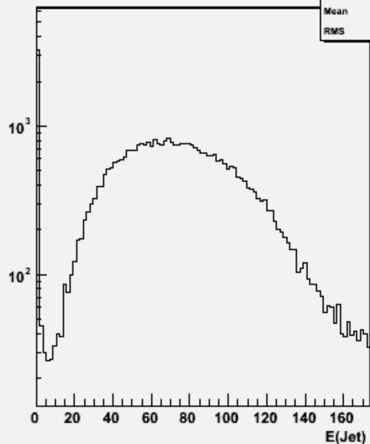
Jet energies(All jets)w101781 cccse2n2_o
