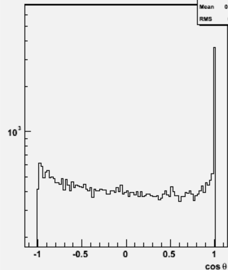
Jet cosθ (All jets)w101781 cccse2n2_o
