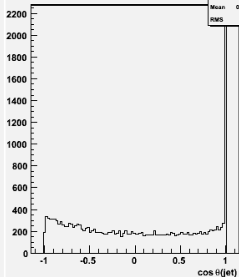
cos \theta for 2-jets :w101781 cccse2n2_o
