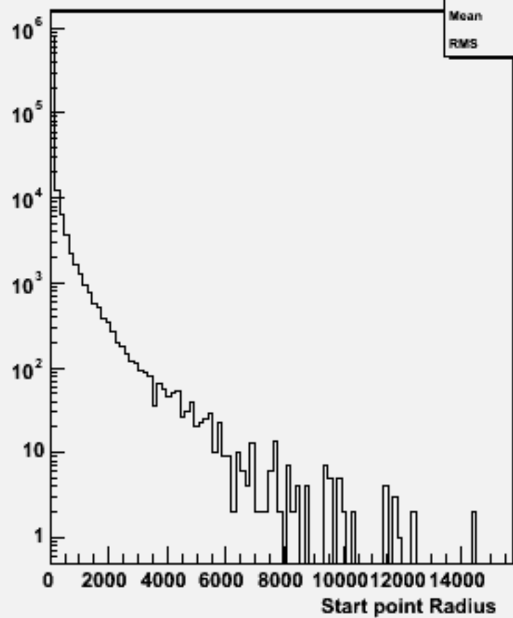
Start point R : w101781 cccse2n2_o
