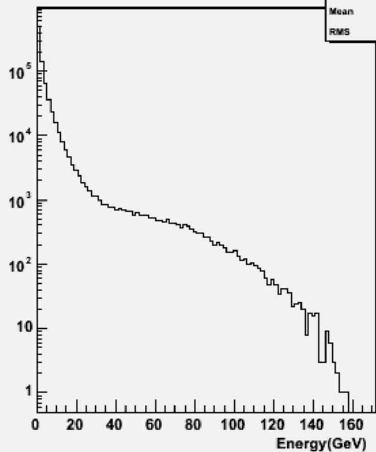
Particle Energy : w101781 cccse2n2_o
