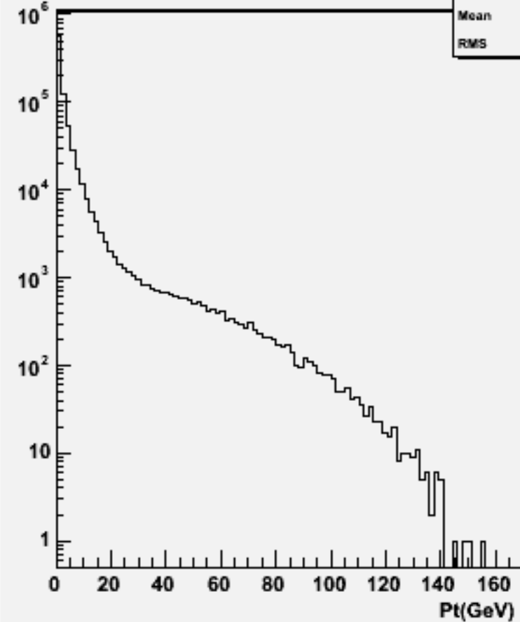
Particle Pt : w101781 cccse2n2_o
