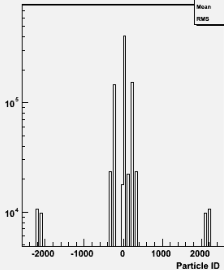
Particle ID : w101781 cccse2n2_o
