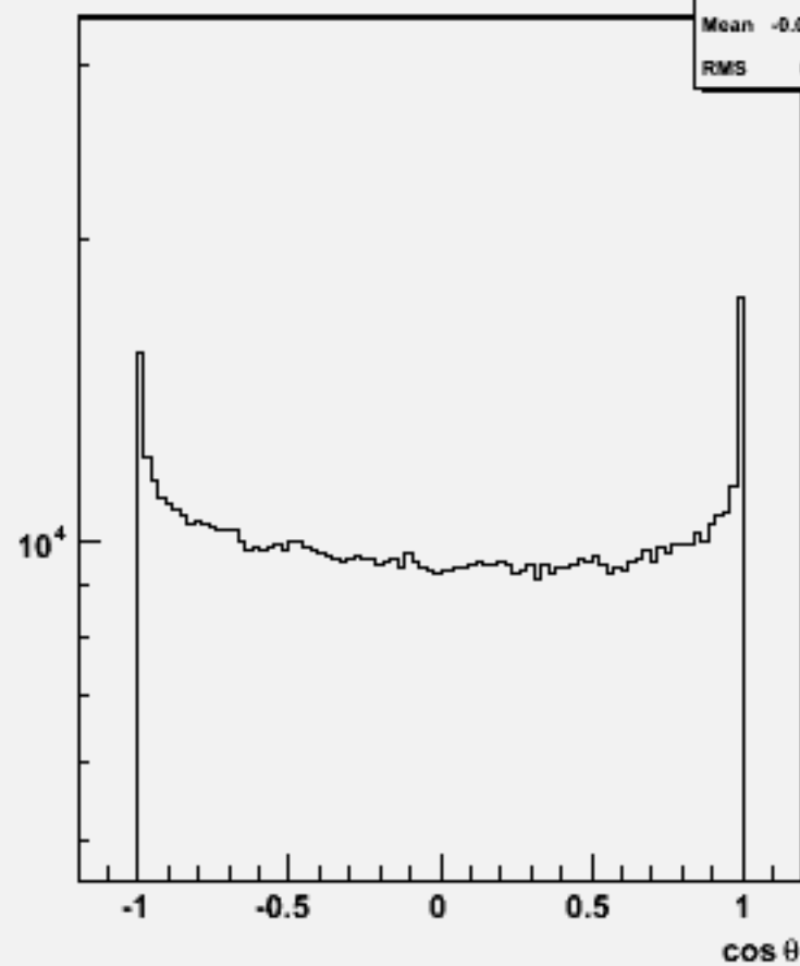
Particle \cos\theta : w101781 cccse2n2_o
