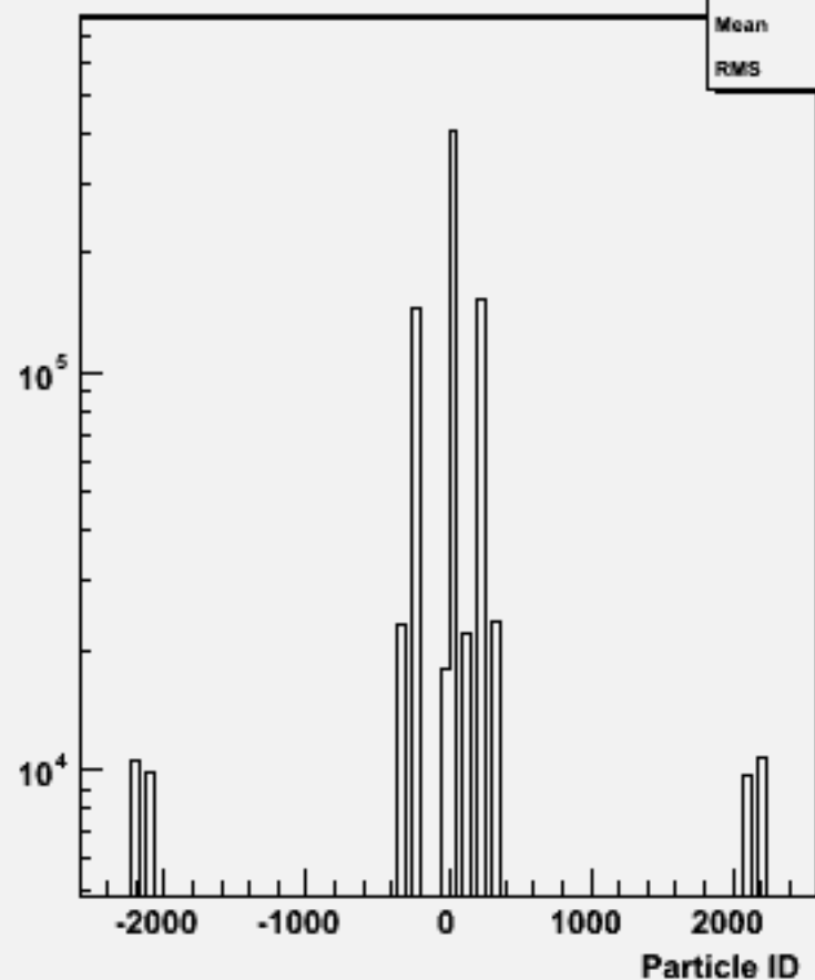
Particle ID : w101778 cccse1n1_o
