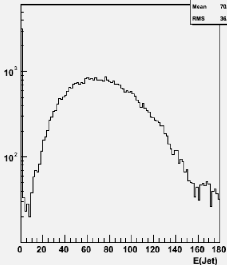
Jet energies(All jets)w101777 cccse1n1_o
