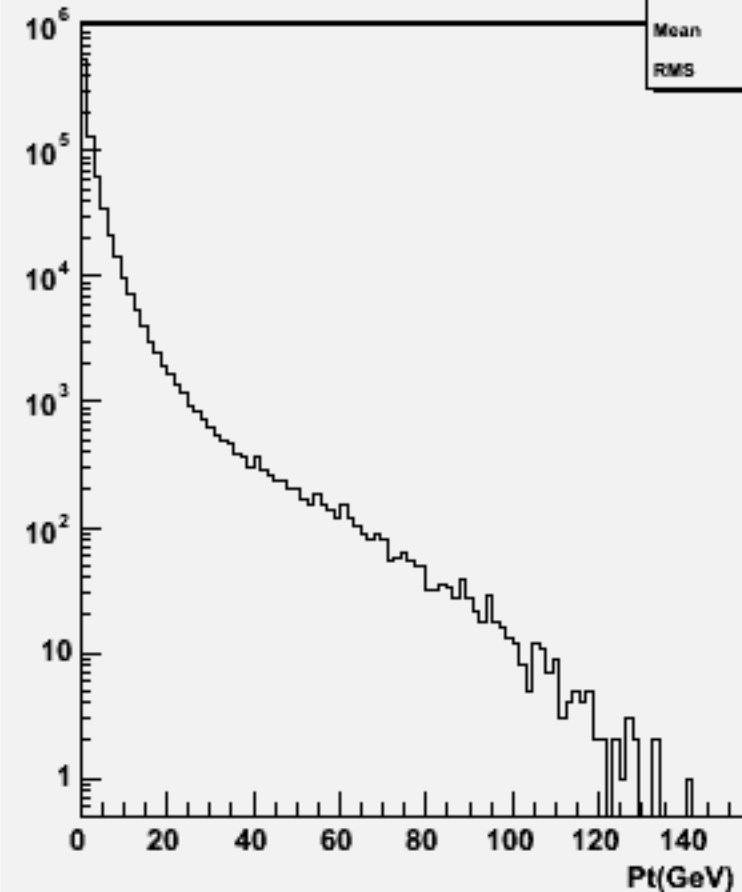
Particle Pt : w101776 cccse1n1_o
