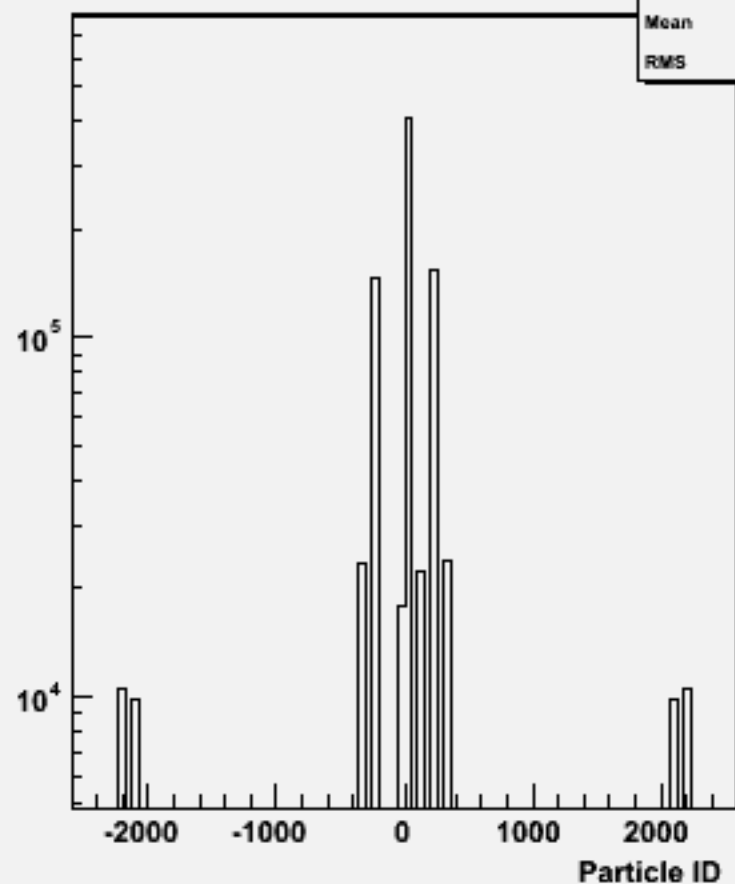
Particle ID : w101776 cccse1n1_o
