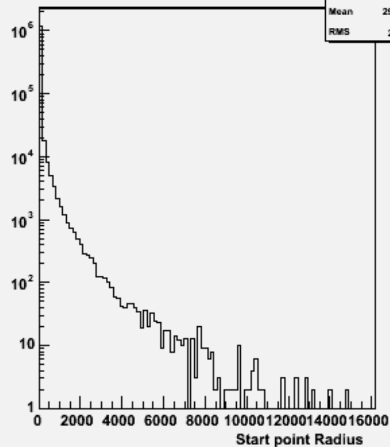
Start point R : w101773 ccudsc_o
