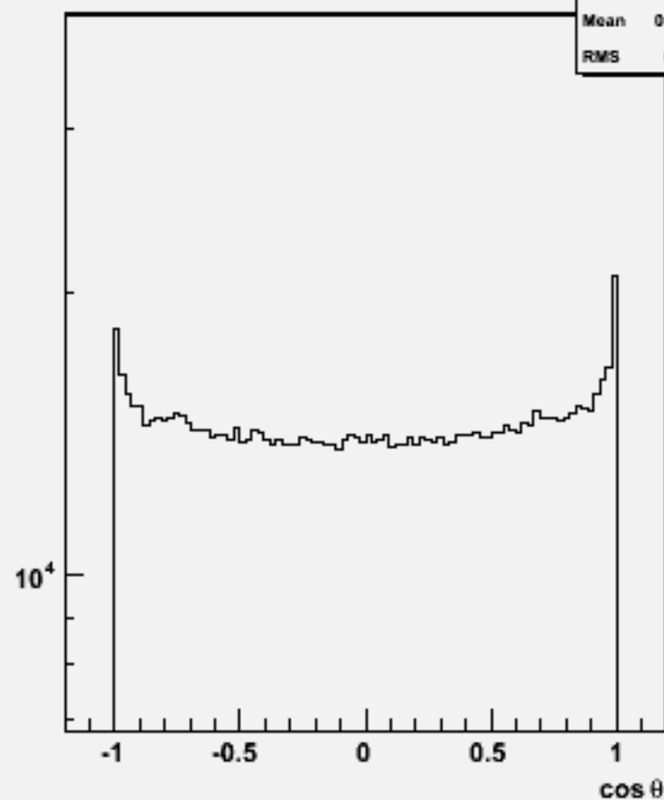
Particle cosθ : w101773 ccudsc_o
