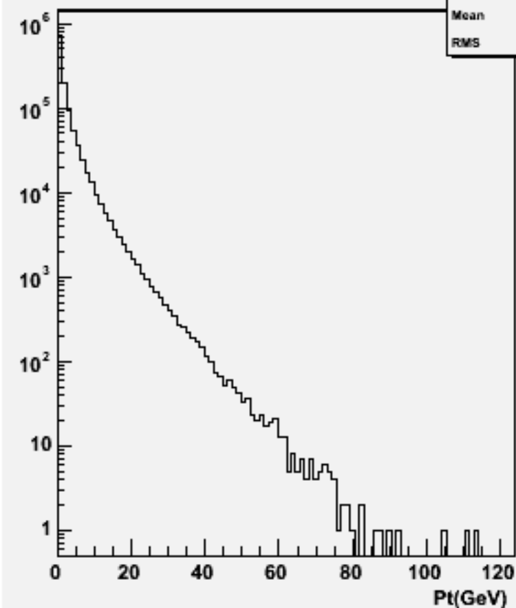
Particle Pt : w101773 ccudsc_o
