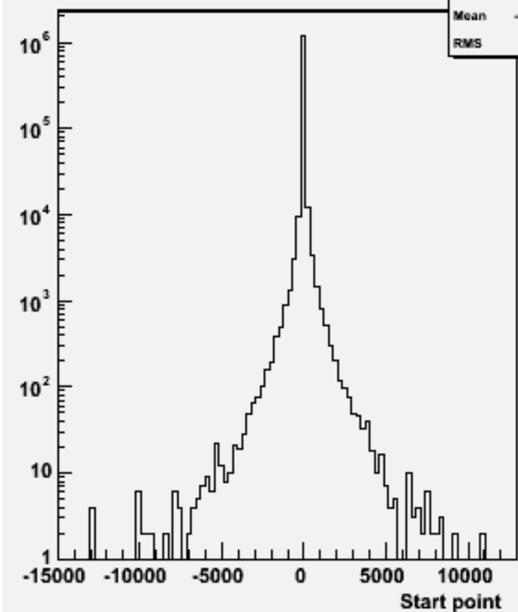
Start point Z : w101773 ccudsc_o
