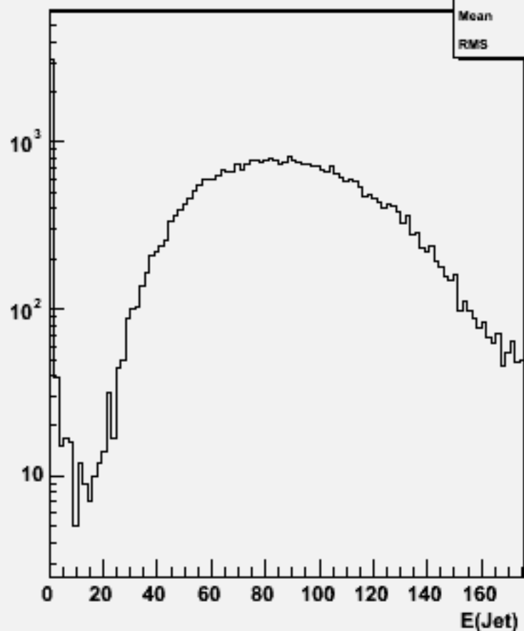
Jet energies(All jets)w101773 ccudsc_o
