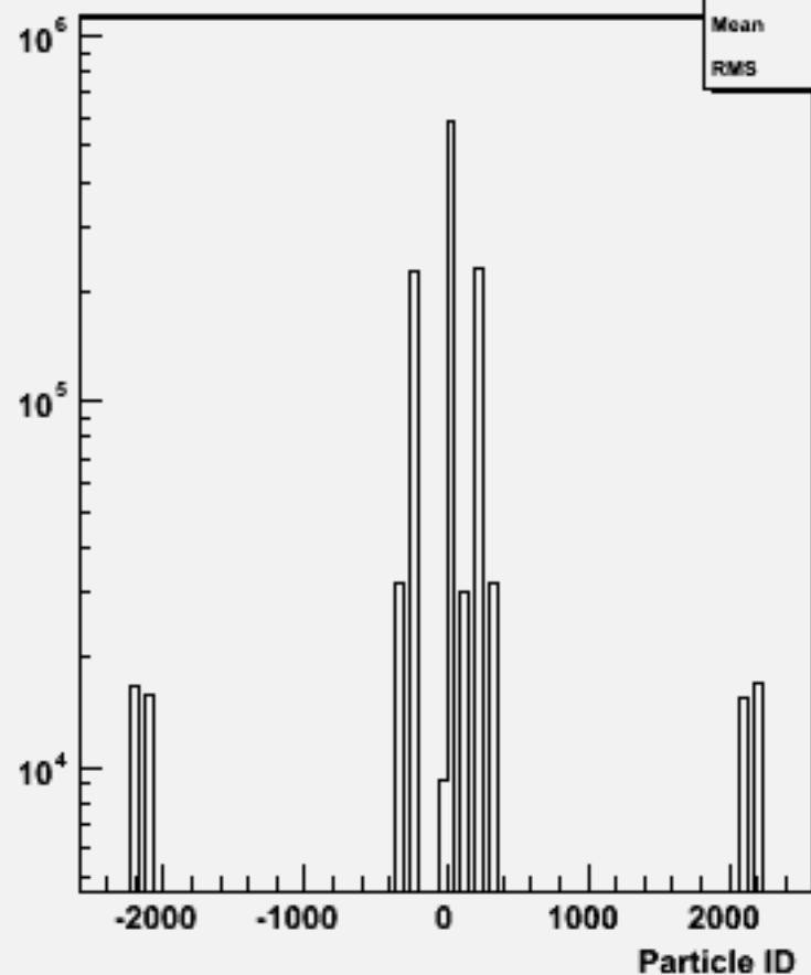
Particle ID : w101773 ccudsc_o
