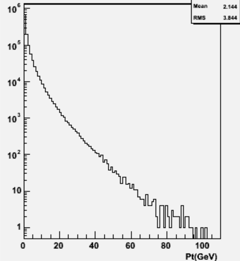
Particle Pt : w101769 ccuddu_o
