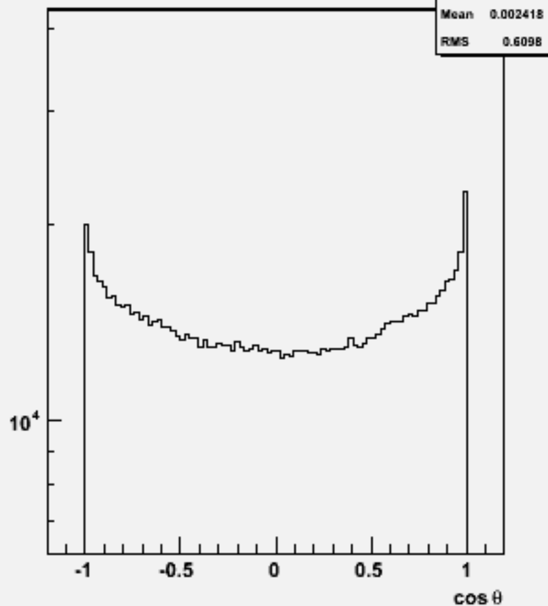
Particle \cos\theta : w101769 ccuddu_o
