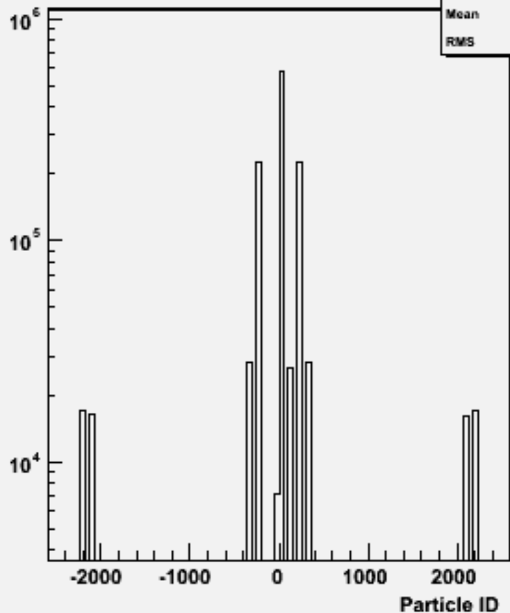
Particle ID : w101769 ccuddu_o
