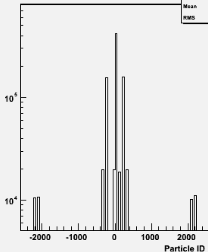
Particle ID : w101765 ccude3n3_o
