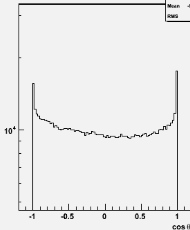
Particle cos \theta : w101765 ccude3n3_o
