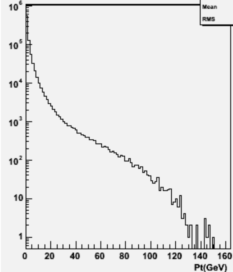
Particle Pt : w101765 ccude3n3_o
