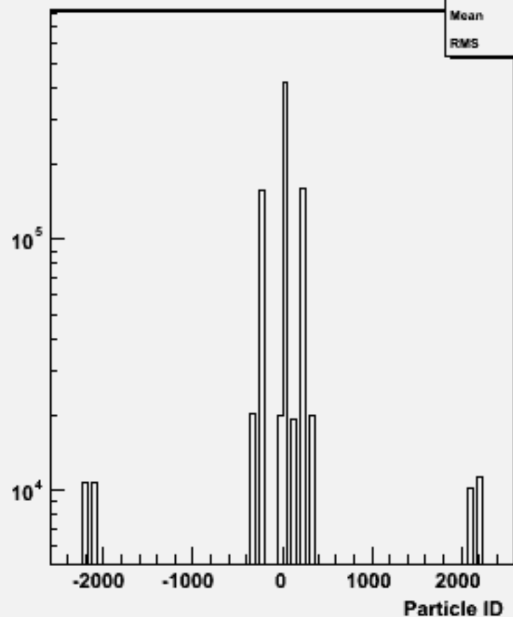
Particle ID : w101764 ccude3n3_o
