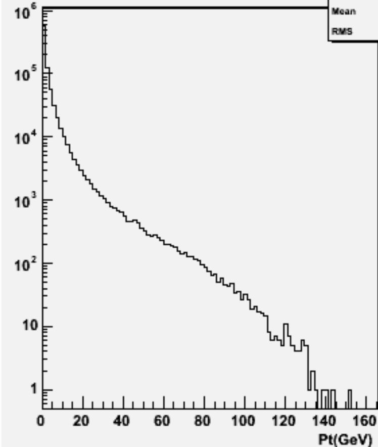
Particle Pt : w101764 ccude3n3_o
