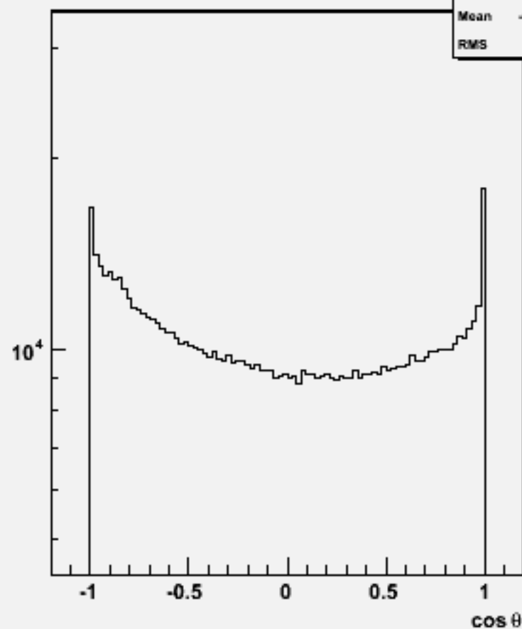
Particle cos \theta : w101764 ccude3n3_o
