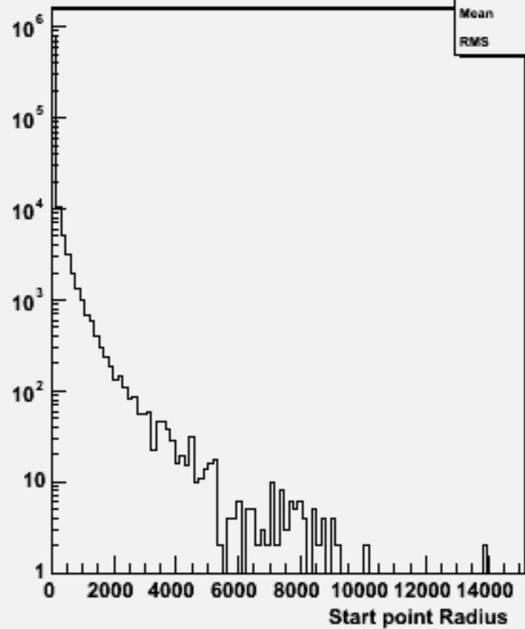
Start point R : w101760 ccude2n2_o
