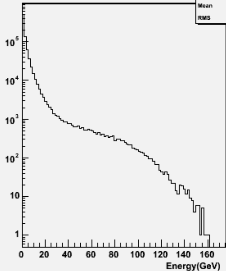
Start point R : w101760 ccude2n2_o
