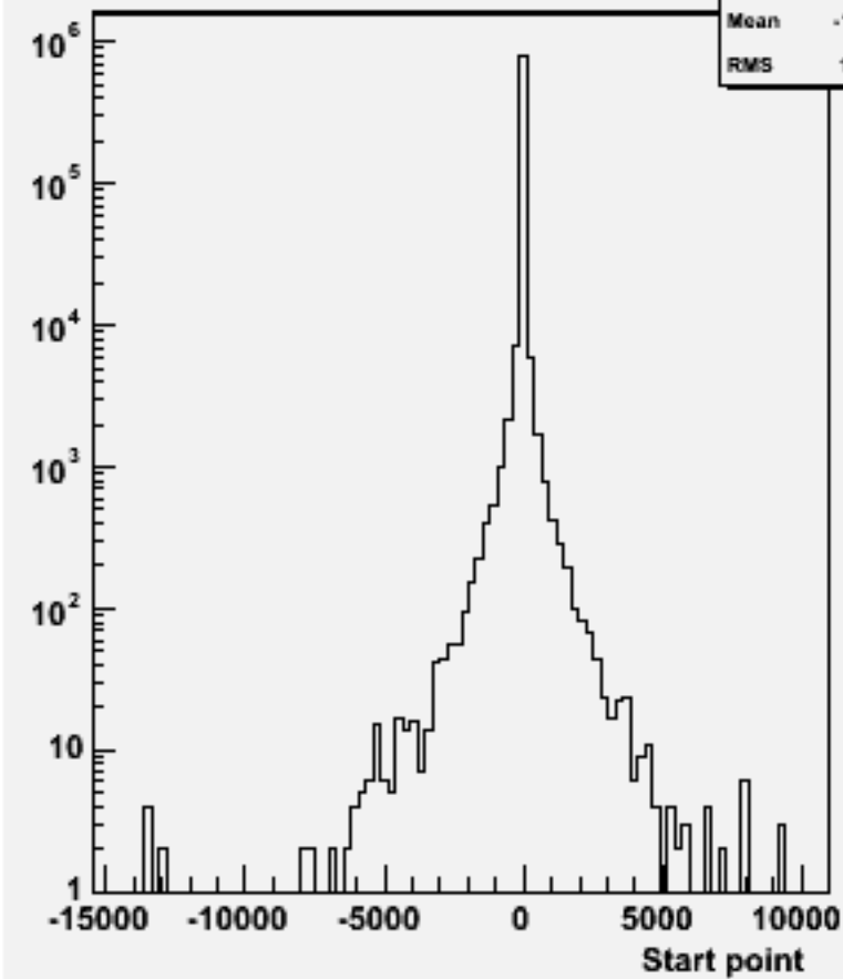
Start point Z : w101760 ccude2n2_o
