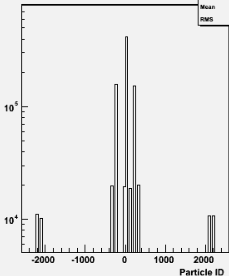
Particle ID : w101749 ccn3e3du_o
