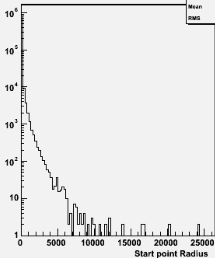
Start point R : w101749 ccn3e3du_o
