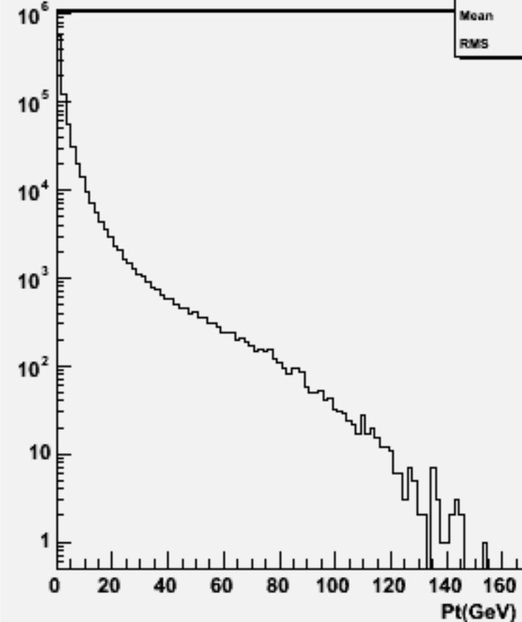
Particle Pt : w101749 ccn3e3du_o
