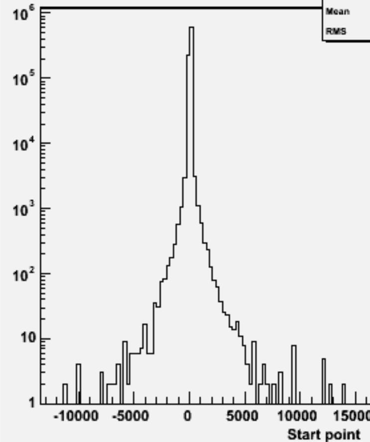
Start point Z : w101749 ccn3e3du_o
