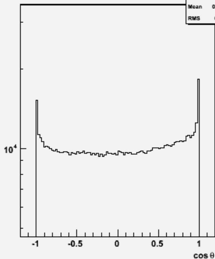
Particle \cos \theta : w101749 ccn3e3du_o
