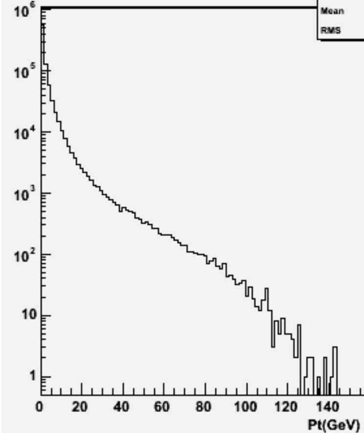
Particle Pt : w101748 ccn3e3du_o
