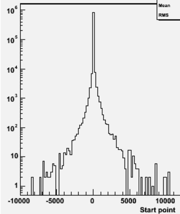
Start point Z : w101748 ccn3e3du_o
