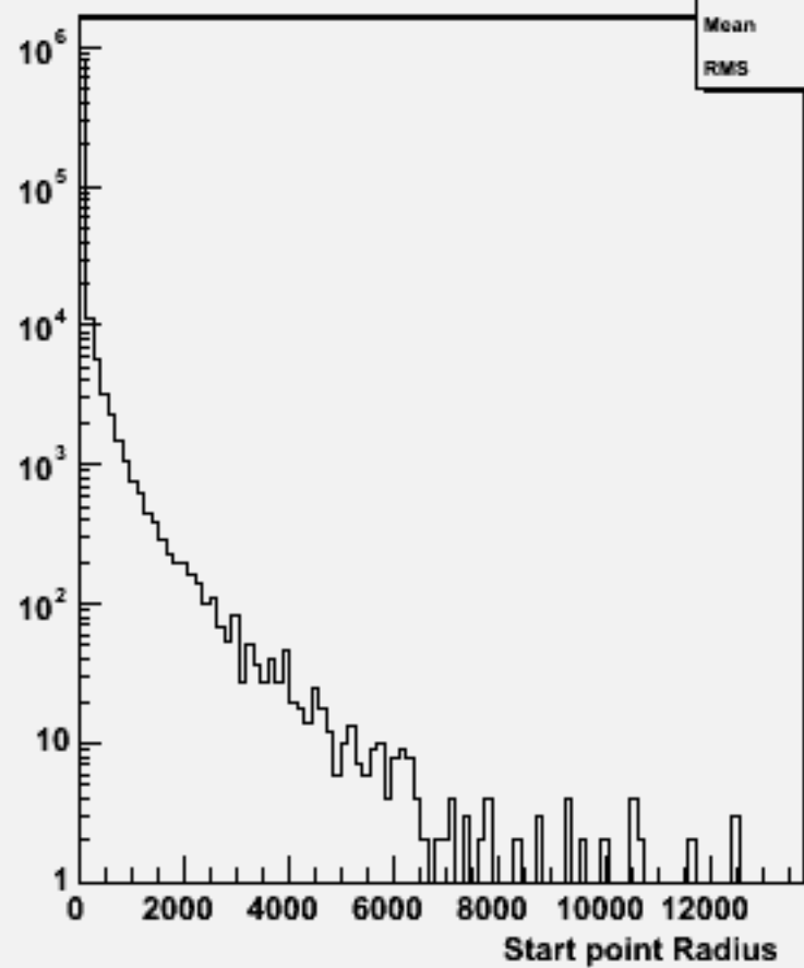
Start point R : w101748 ccn3e3du_o
