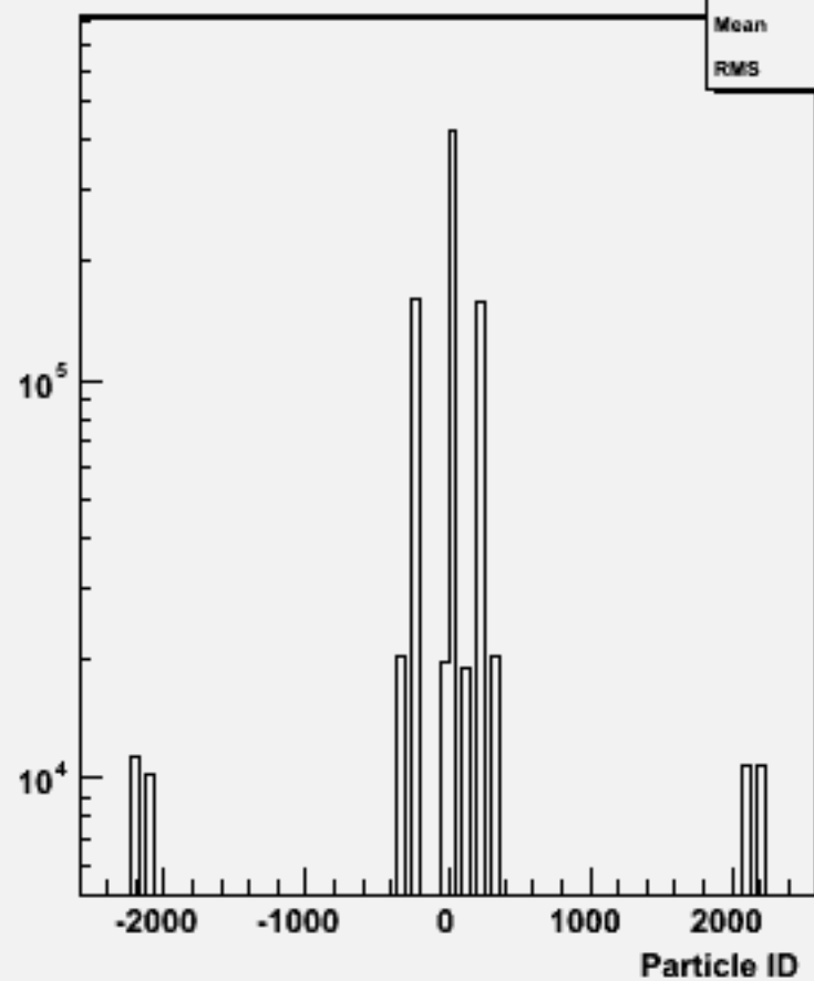
Particle ID : w101748 ccn3e3du_o
