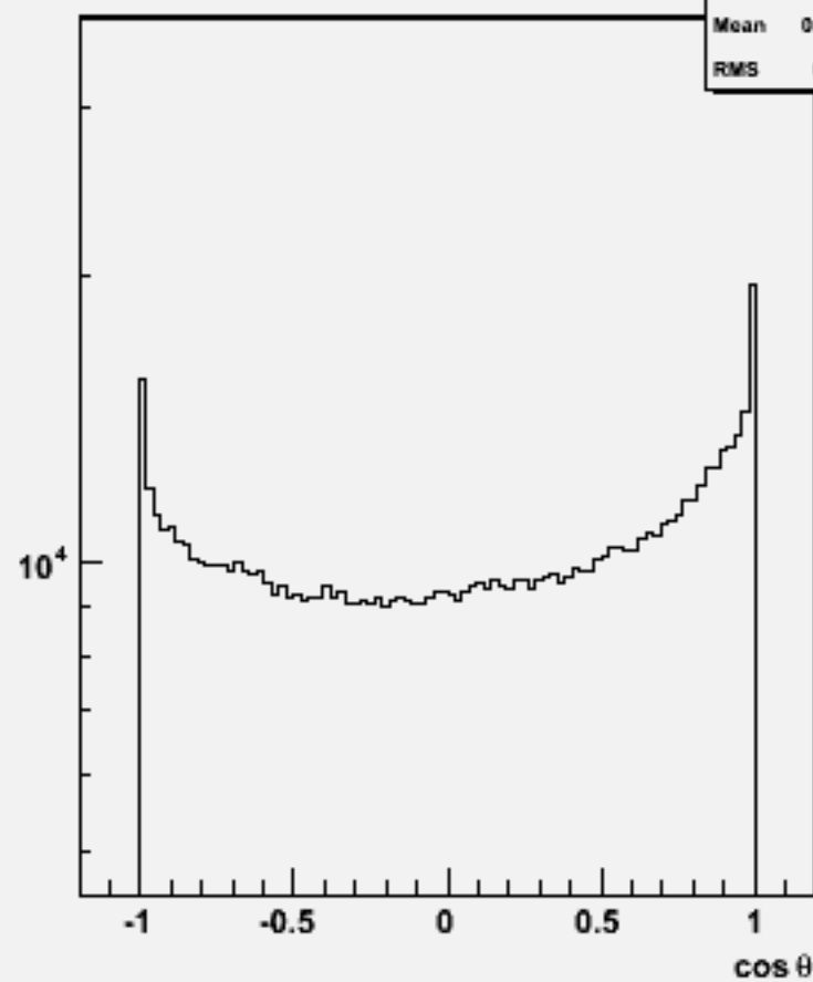
Particle cos \theta : w101748 ccn3e3du_o
