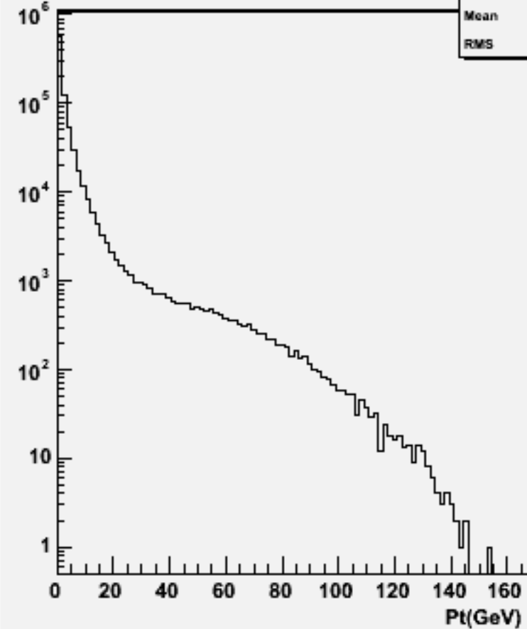
Particle Pt : w101733 ccn2e2sc_o
