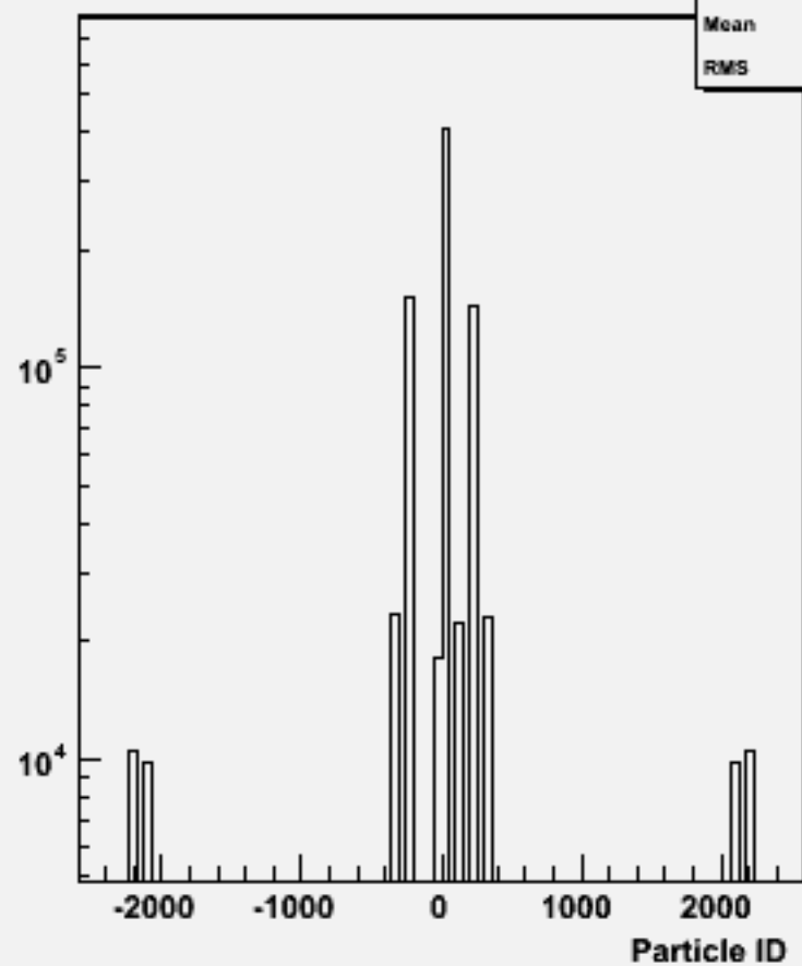
Particle ID : w101733 ccn2e2sc_o
