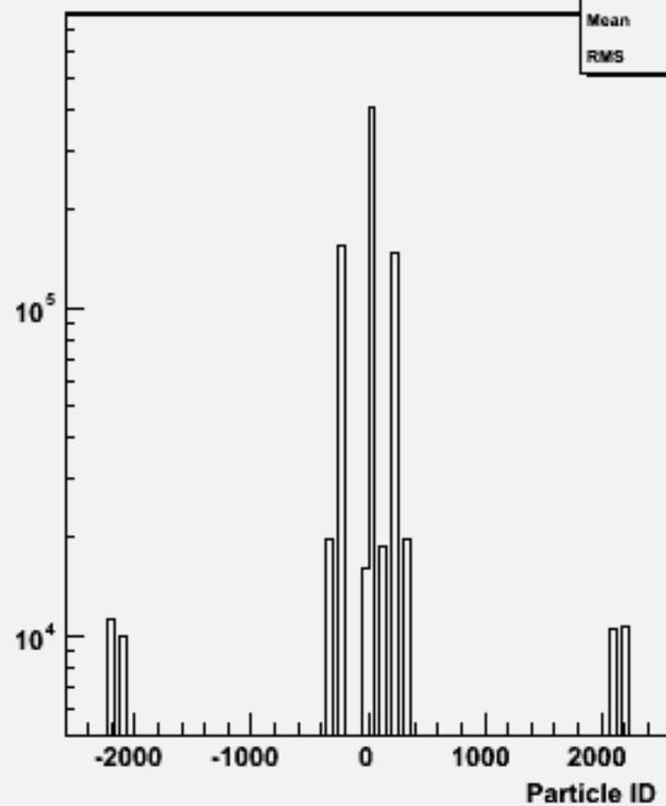
Particle ID : w101729 ccn2e2du_o
