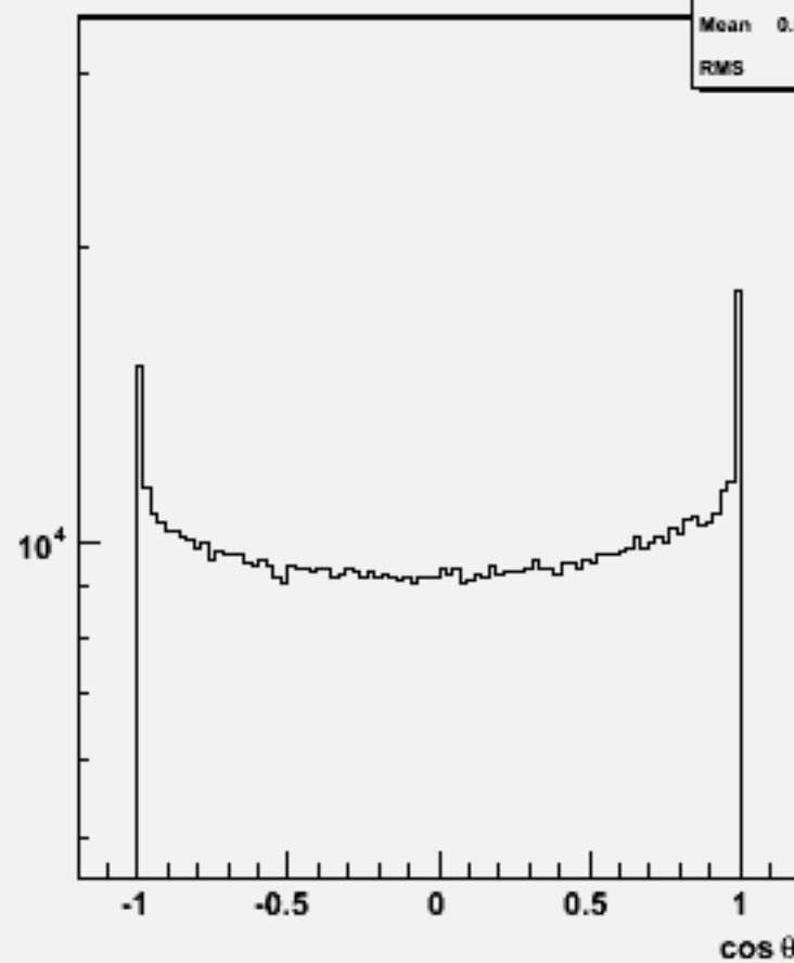
Particle cos \theta : w101729 ccn2e2du_o
