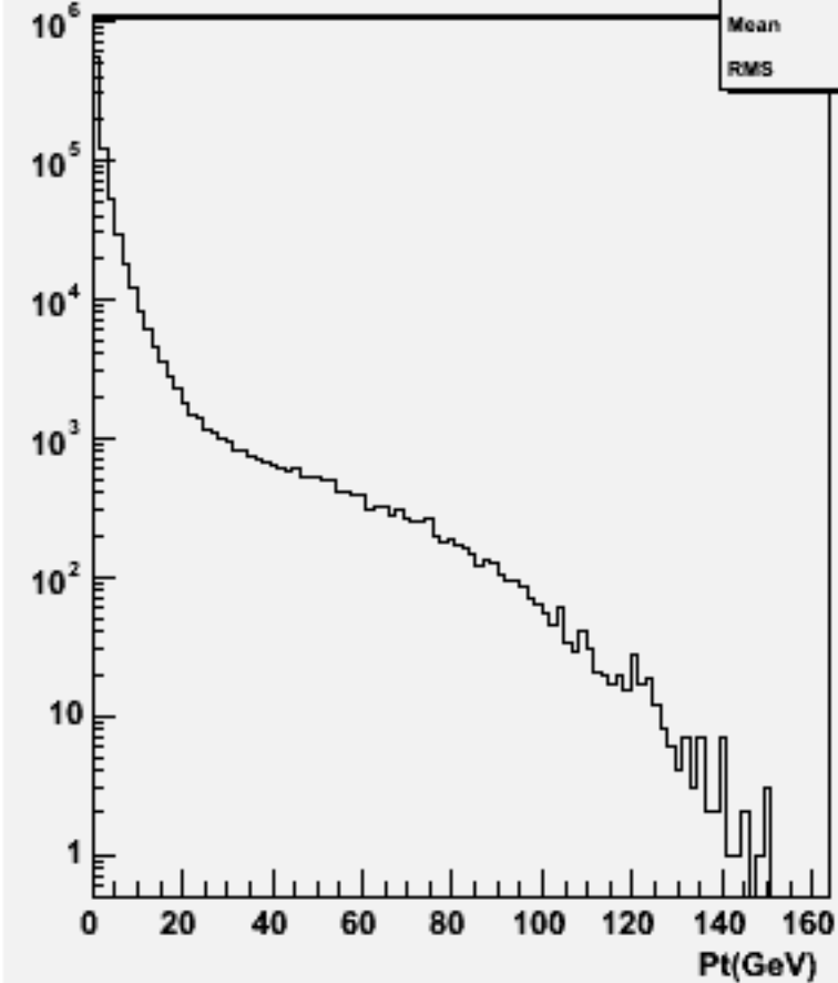
Particle Pt : w101729 ccn2e2du_o
