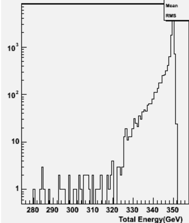
Pt Sum: w101720 ccn2e2e2n2_o
