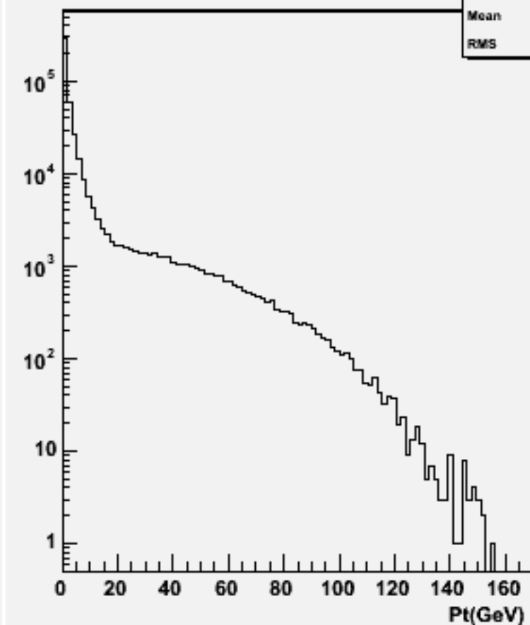
Particle Pt : w101720 ccn2e2e2n2_o
