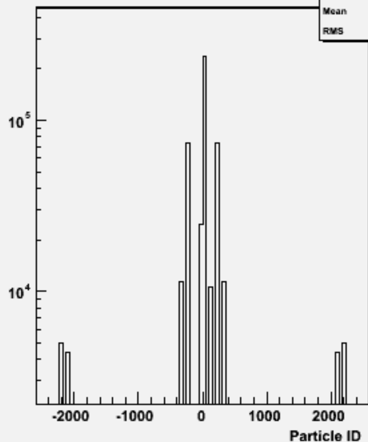
Particle ID : w101720 ccn2e2e2n2_o
