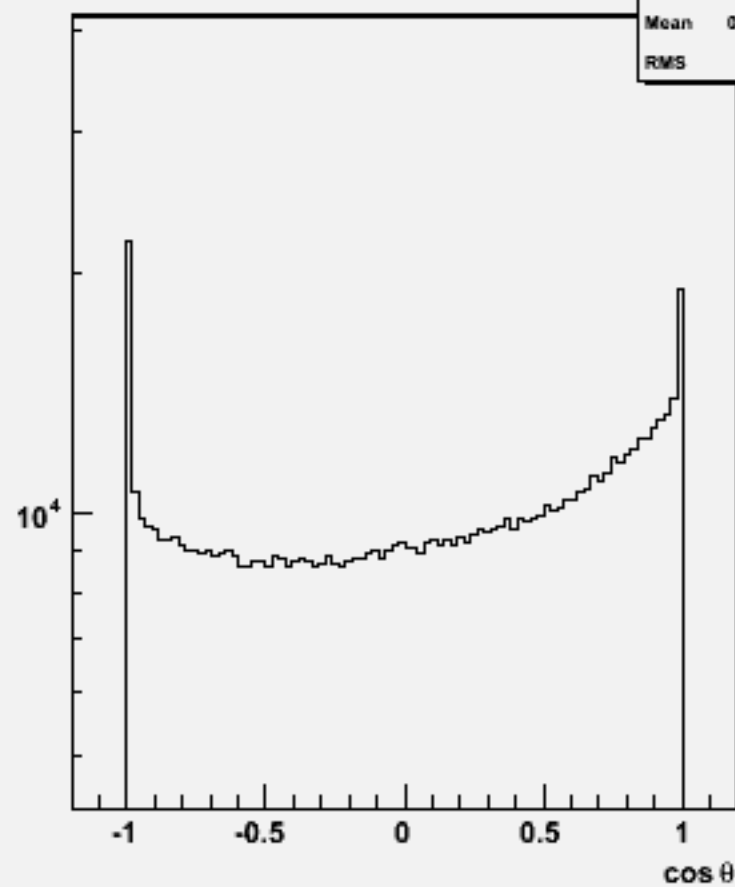
Particle cosθ : w101712 ccn1e1sc_o
