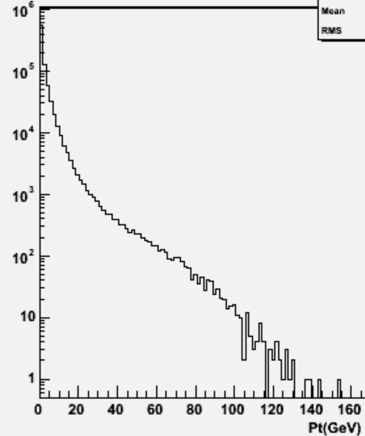
Particle Pt : w101712 ccn1e1sc_o
