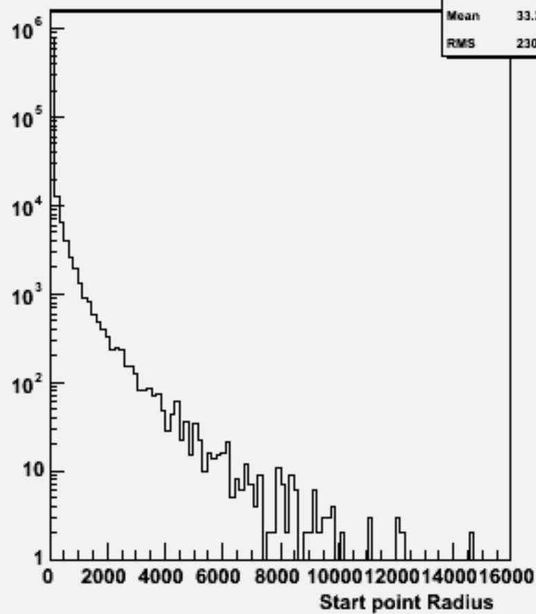
Start point R : w101712 ccn1e1sc_o
