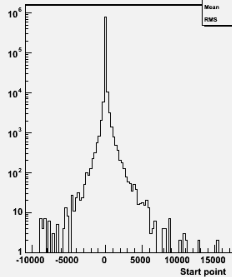
Start point Z : w101712 ccn1e1sc_o
