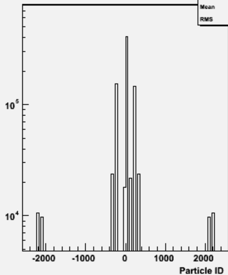
Particle ID : w101712 ccn1e1sc_o
